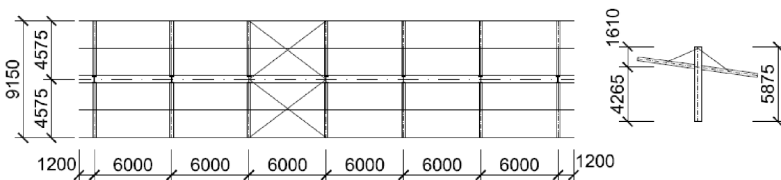
(Schéma půdorysu a příčné vazby zastřešení, kótováno v mm)
