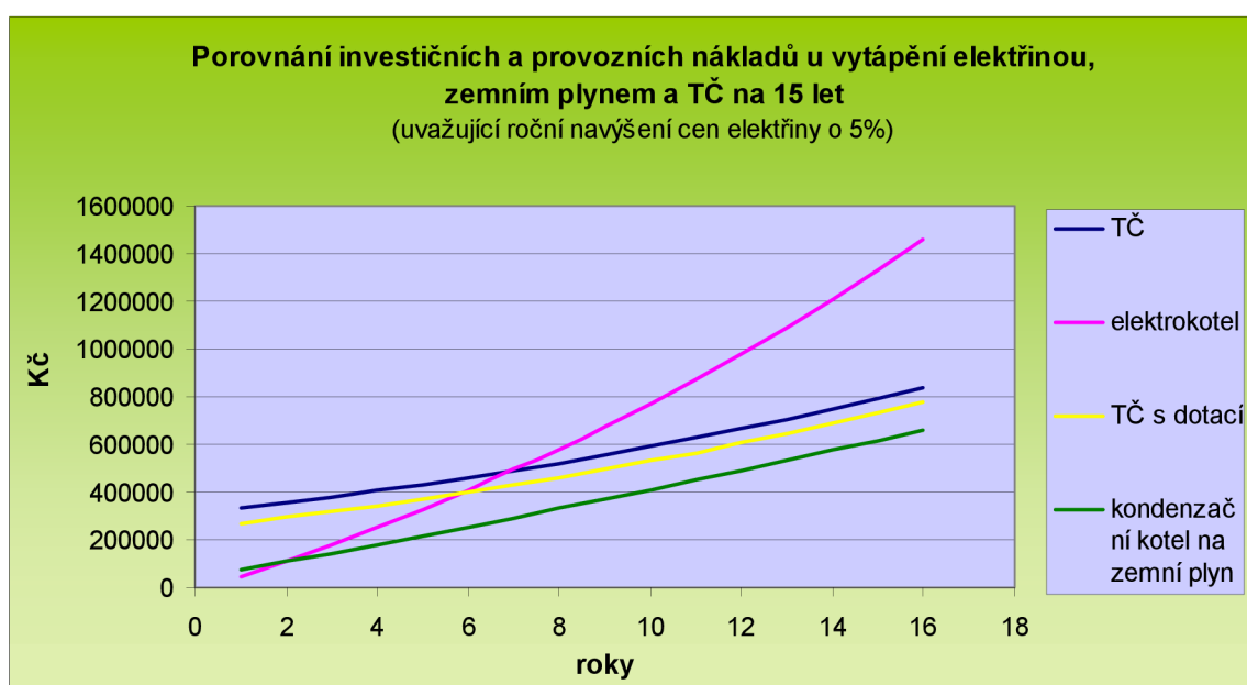
Obr. 11 – Porovnání investičních a provozních nákladů u vytápění elektrinou, zemním plynem a TČ na 15 let
