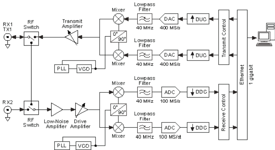
Obr. 1.13: USRP architektúra
