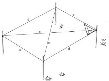
Obr.13 – Vyměření základů domu 121
