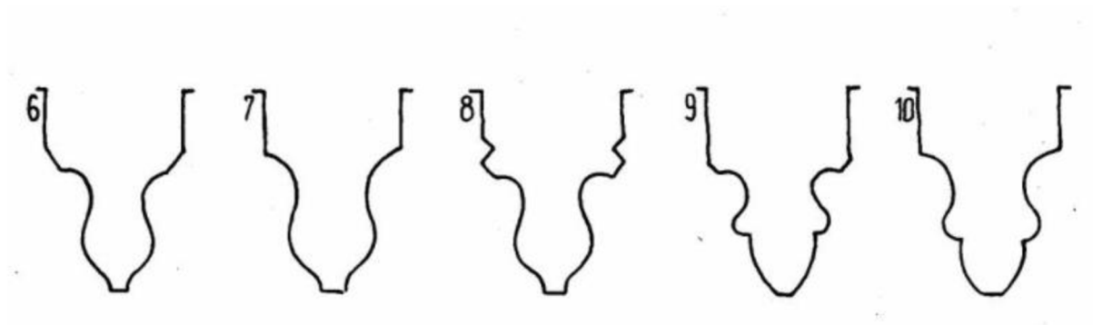
[27] Profilace žebíř posledního dvacetiletí 13. století, 6) Nymburk, děkanský kostel, presbytář 7) V. Brod, kapitulní síň, Čáslav, presbytář 8) V. Brod, stř. presbytář 9) Plzeň, minorité, boční loď 10) Zl. Koruna, Andělé str.
