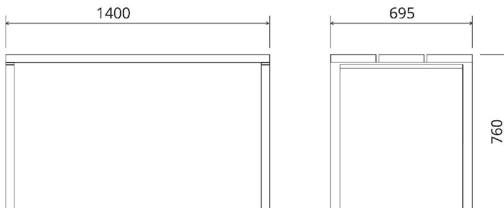
Obrázek 20: Schéma stolu
