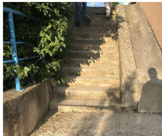
Obrázek 9: Schodiště – trhlina
