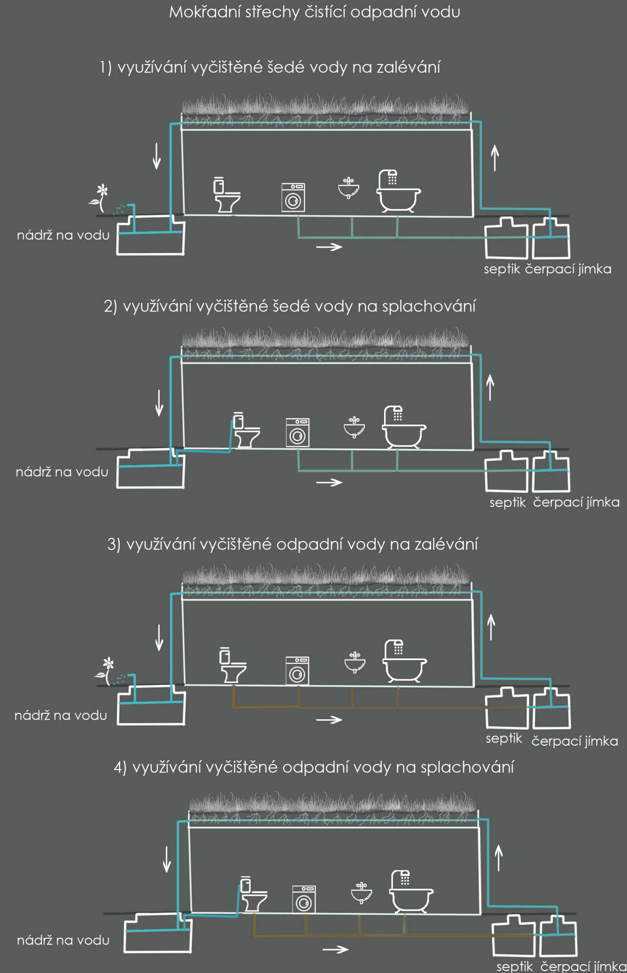
obr. 12 Schéma mokřadních střešek (autorka práce 2023)
