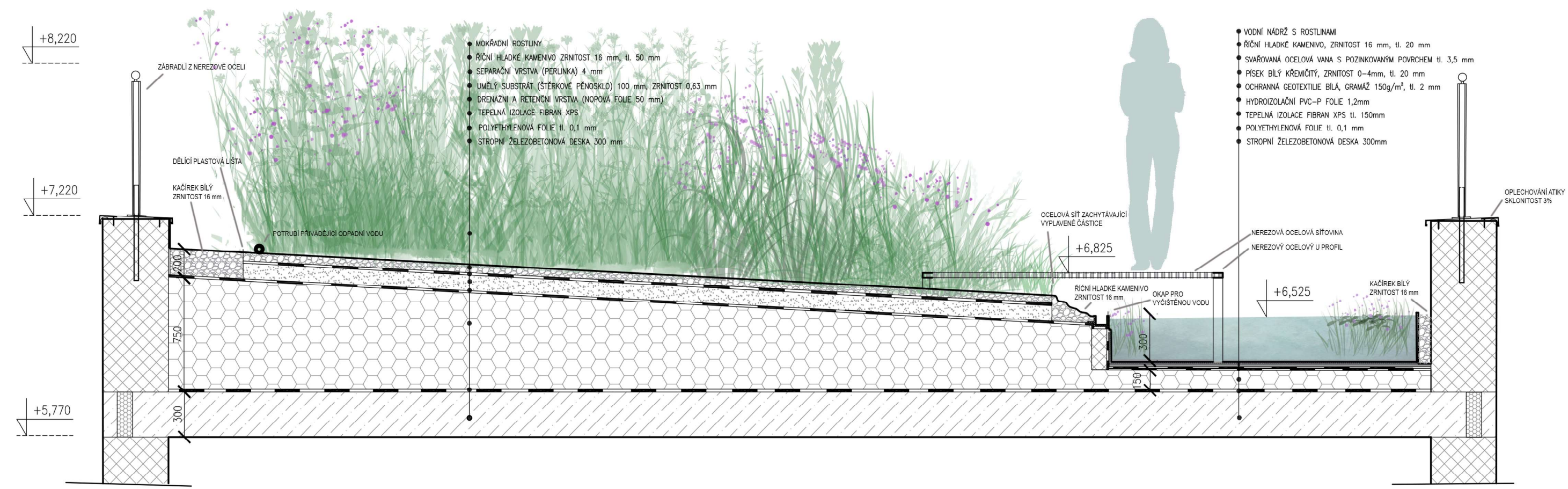
obr. 27 Řez (autorka práce 2023)
