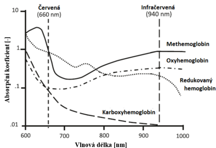
Obr. 2.2: Závislost absorpčního koeficientu na vlnové délce pro oxyhemoglobin, karboxyhemoglobin, methemoglobin a redukovaný hemoglobin. Převzato z [27].
