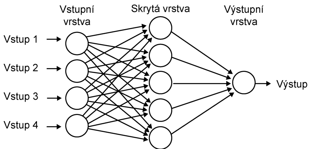
Obr. 3.6: Dopředná neuronová síť se čtyřmi vstupními příznaky a s jednou skrytou vrstvou. Výstupní vrstva dává řešení v podobě konkrétní hodnoty.
