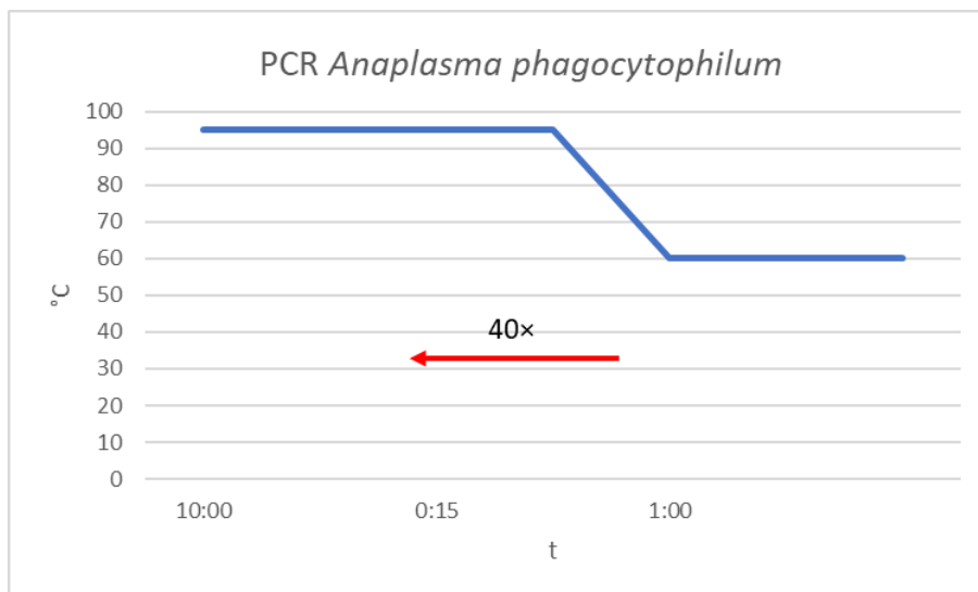
Obrázek 7 - zobrazení podmínek PCR reakce pro Anaplasma phagocytophilum
