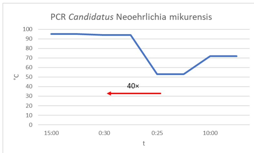
Obrázek 5 - zobrazení podmínek PCR reakce pro Candidatus Neoehrlichia mikurensis
