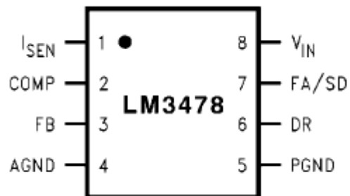
Obr. 20 Měníč LM3478
