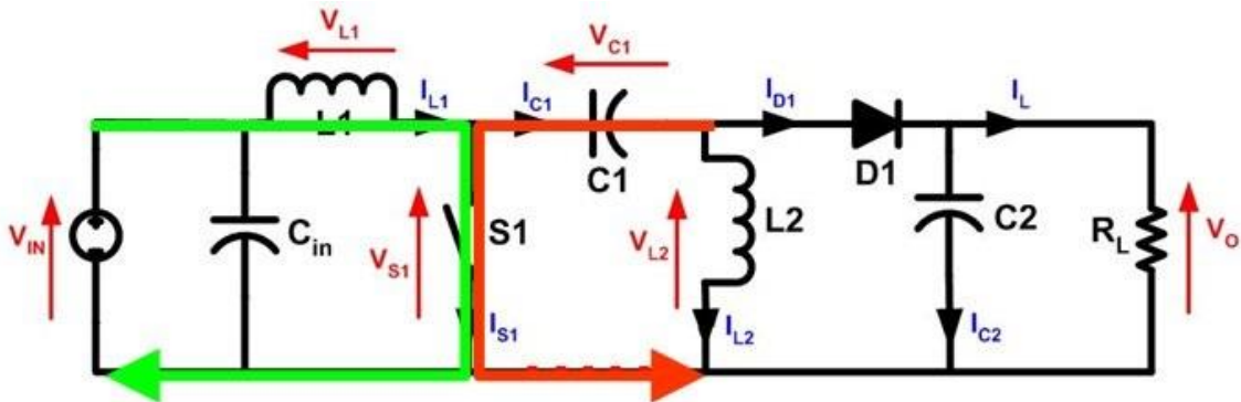
Obr. 12 Když S1 uzavřen, proud se zvyšuje přes L1 (zelená) a C1 vybije zvyšující proud na L2
