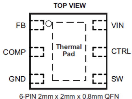
Obr. 21 Měníč TPS61170
