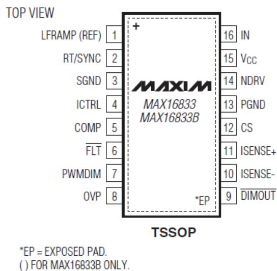
Obr. 19 Měnič MAX16833/16833B
