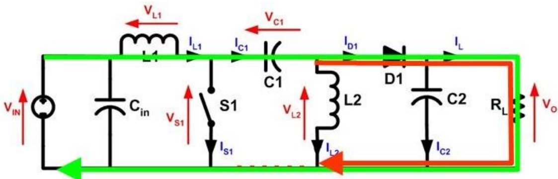
Obr. 13 Když S1 je zapnut, proudy L1 (zelené) a proud L2 (červená) produkují proud zátěže
