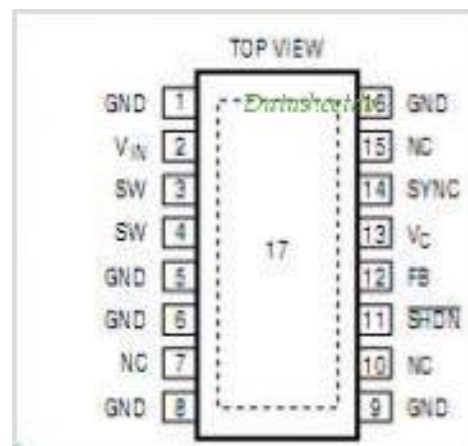
Obr. 22 Měnič LT3436
