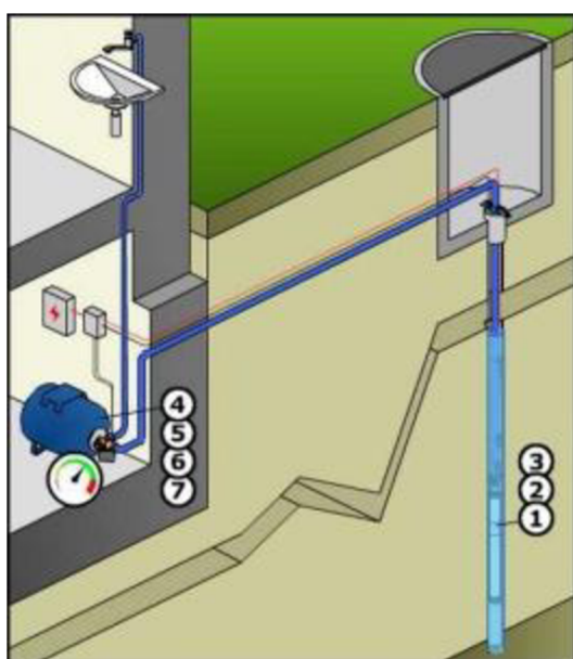
Obr. č. 14 – Schéma domácí vodárny s vrtem 39)
