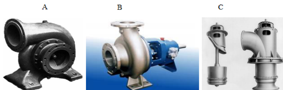
Obr. č. 12 – radiální(A), diagonální(B), axiální čerpadlo(C) 37)
