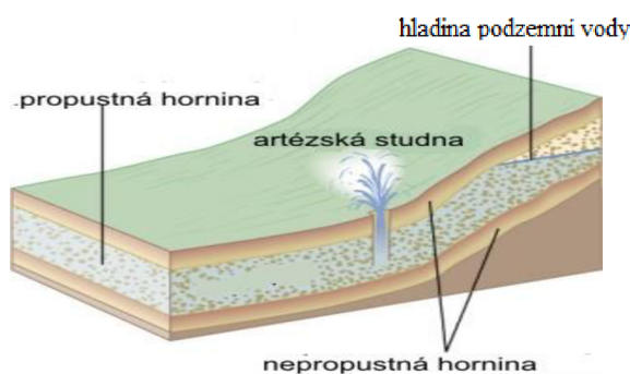
Obr. č. 5 – Artézská studna 14)
