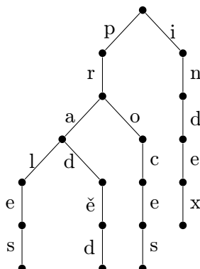
Obrázek 4.1: Struktura Trie.
