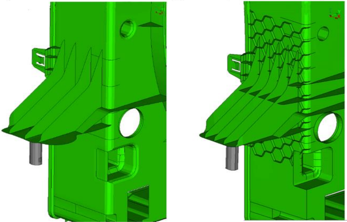
Obr. 43 Porovnání počtu žebér na rámu pro zvýšení celkové pružnosti [13]
