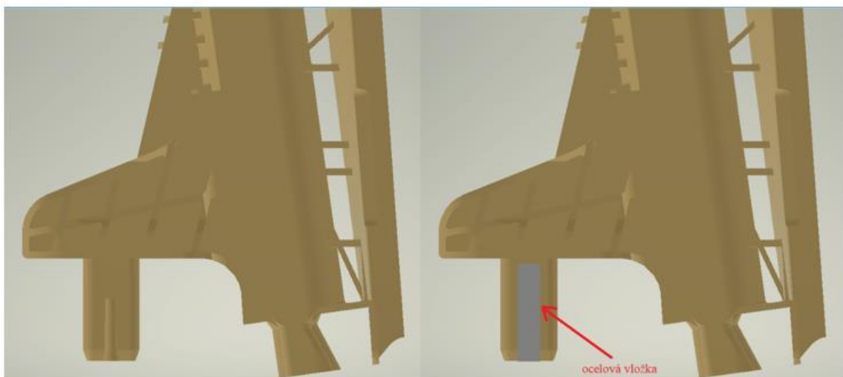
Obr. 44 Porovnání čepu bez a s ocelovou vložkou
