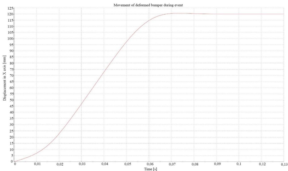
Obr. 37 Graf kinematického pohybu deformovaného příčnicku [13]
