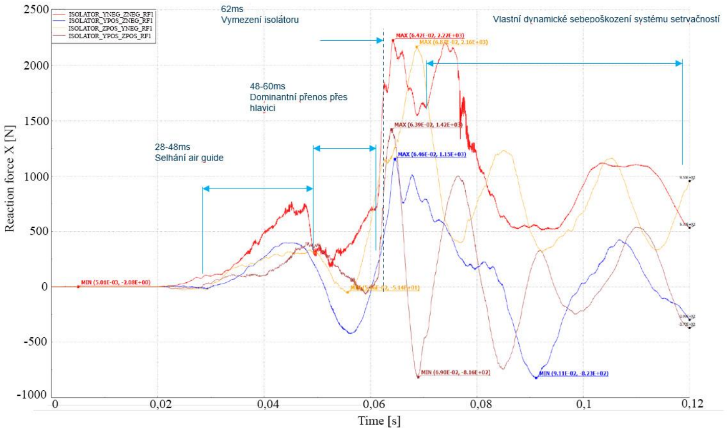
Obr. 41 Graf závislosti reakční síly izolátoru na času [13]
