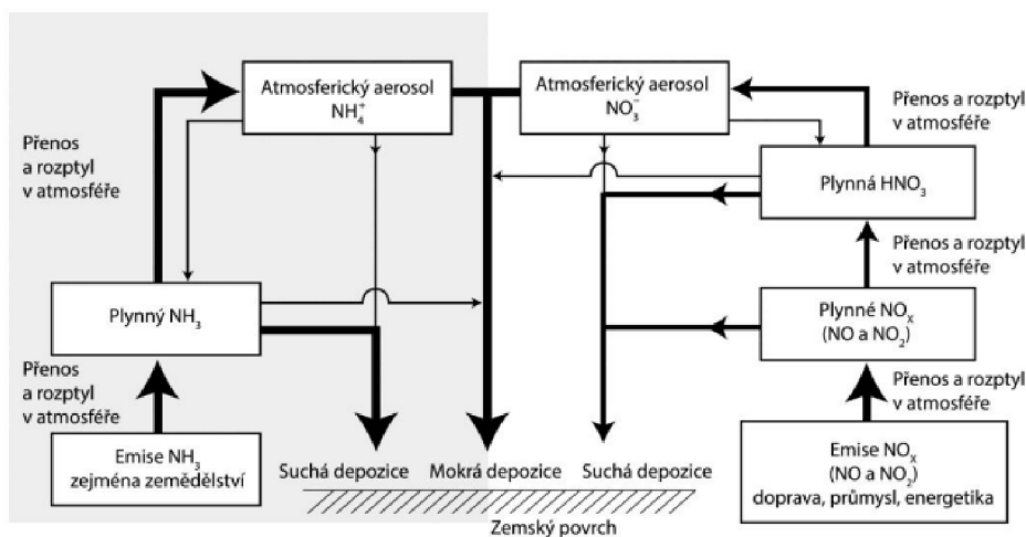
Obrázek 3 - Schéma atmosférické deponice dusíku (Hůnová et al. 2019)
