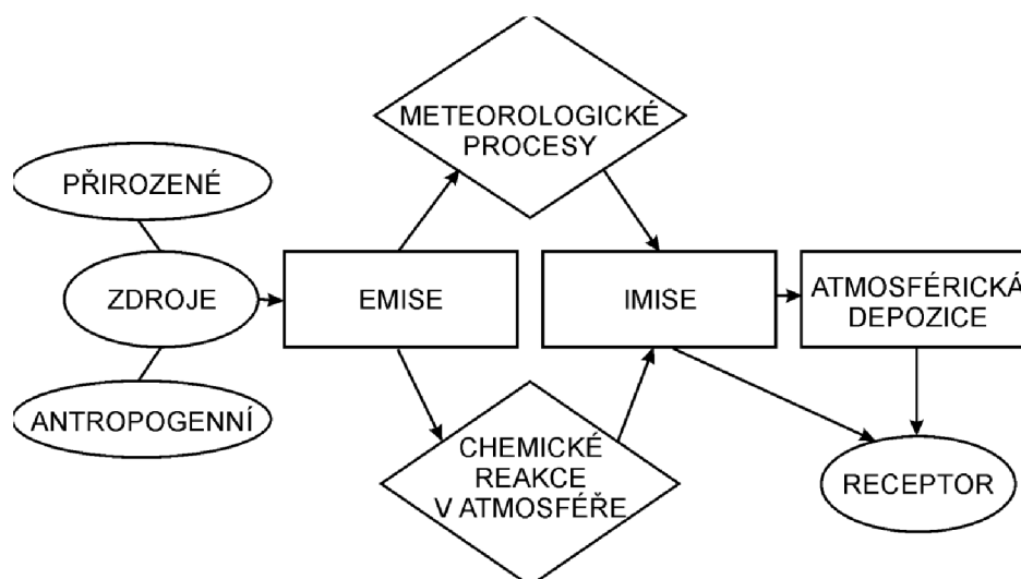
Obrázek 1 - Schéma procesů, jimiž podléhají látky znečišťující ovzduší (Hůnová 2009)
