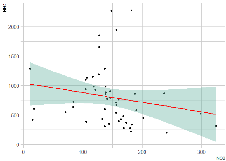
Graf 7 - Znáornění možné závislosti mezi \text{NH}_4^+ a \text{NO}_2
