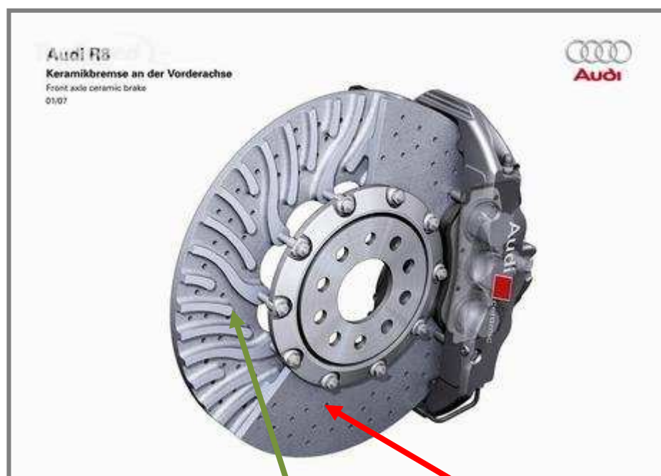
Funkční plocha disku Žebra tvarovaná tak, aby mezi nimi rotací disku vznikalo proudění vzduchu
