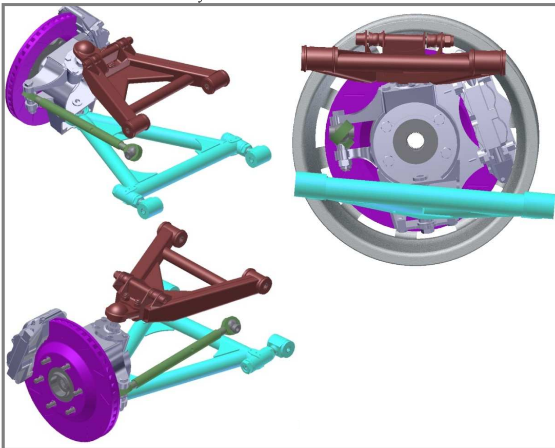
Obr. 7 Ukázka zpracovaných dílů kolem štítu
