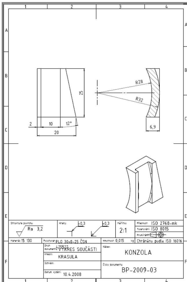
Obr. 18 Výkres konzoly
