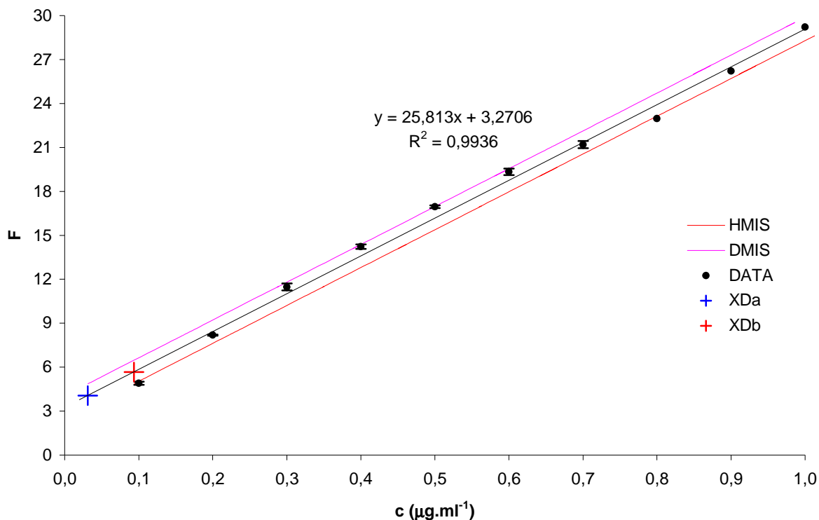
Obr. 50: Kalibrační závislost 0,1 – 1 µg.ml -1 Sc 3+ s intervaly spolehlivosti. Koncentrace morinu 2,22 \cdot 10^{-4} mol.l -1 , E = 505 V při pH 2,5
