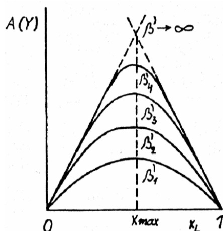
Obr. 20: Tvar variačních křivek pro komplexy 1:1, pro různé podmíněné konstanty stability. x_{\max} – maximum závislosti [ML_n] = f(x_L) , \beta_1' - \beta' – podmíněné konstanty stability.
