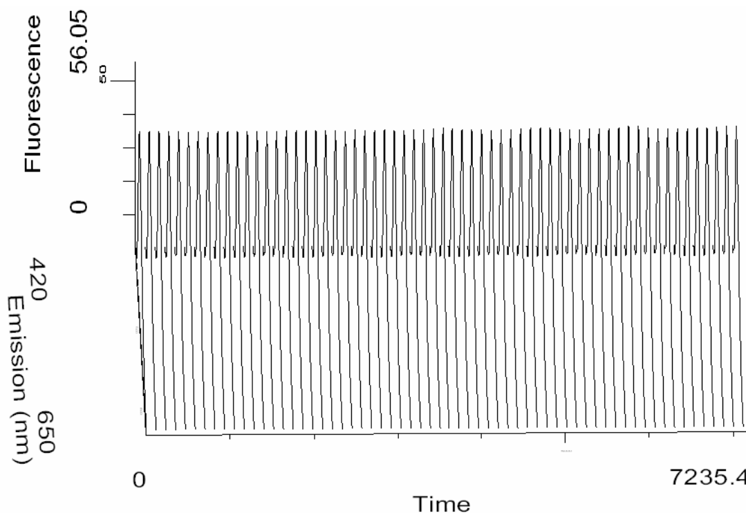
Obr. 33: 3D časové spektrum komplexu 1,11 \cdot 10^{-5} \text{ mol.l}^{-1} ( 0,5 \text{ } \mu\text{g.ml}^{-1} ) \text{Sc}^{3+} a 1,11 \cdot 10^{-4} \text{ mol.l}^{-1} 8-hydroxychinolin-5-sulfonové kyseliny v přítomnosti 0,0012 \text{ mol.l}^{-1} zephyraminu, E = 610 \text{ V} a při \text{pH } 4,5 . Obrázek stejný jako obr. 32 pouze z jiné perspektivy.
