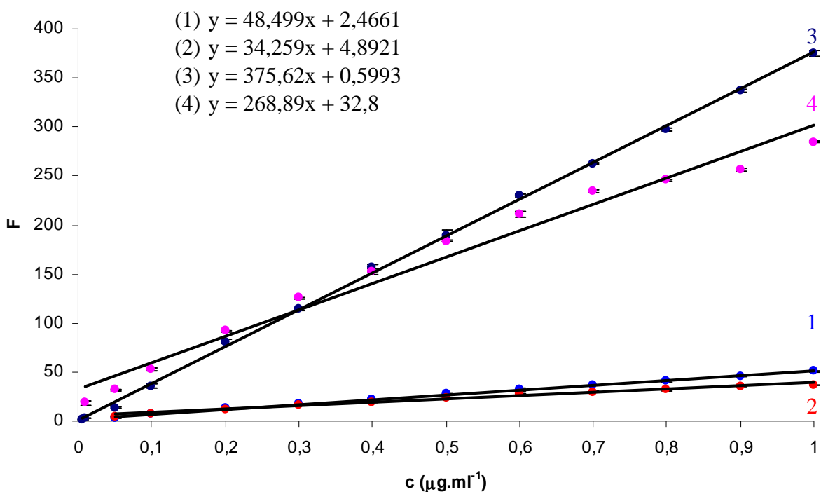
Obr. 37: Kalibrační závislosti komplexu Sc^{3+} pro koncentrace 0,1 - 1 \mu\text{g}\cdot\text{ml}^{-1} a koncentraci činidla 1,11 \cdot 10^{-4} \text{ mol}\cdot\text{l}^{-1} při \text{pH} = 4,5 a E = 700 \text{ V} (1) v nepřítomnosti zephyraminu i HTMA (hexamethylentetramin), (2) v nepřítomnosti zephyraminu a 0,05 \text{ mol}\cdot\text{l}^{-1} HTMA, (3) v přítomnosti 0,0012 \text{ mol}\cdot\text{l}^{-1} zephyraminu a v nepřítomnosti HTMA, (4) v přítomnosti 0,0012 \text{ mol}\cdot\text{l}^{-1} zephyraminu a 0,05 \text{ mol}\cdot\text{l}^{-1} HTMA.
