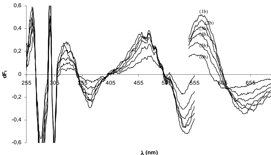
Obr. 60: První derivace excitačních a emisních (b) spekter komplexu s měnící se koncentrací skandia v přítomnosti 5,56 \cdot 10^{-5} \text{mol}\cdot\text{l}^{-1} lumogallionu při E = 845 \text{ V} při \text{pH} 5 . 1 - 1 \mu\text{g}\cdot\text{ml}^{-1} , 2 - 0,8 \mu\text{g}\cdot\text{ml}^{-1} , 3 - 0,6 \mu\text{g}\cdot\text{ml}^{-1} , 4 - 0,4 \mu\text{g}\cdot\text{ml}^{-1} , 5 - 0,2 \mu\text{g}\cdot\text{ml}^{-1} , 6 - 0 \mu\text{g}\cdot\text{ml}^{-1}
