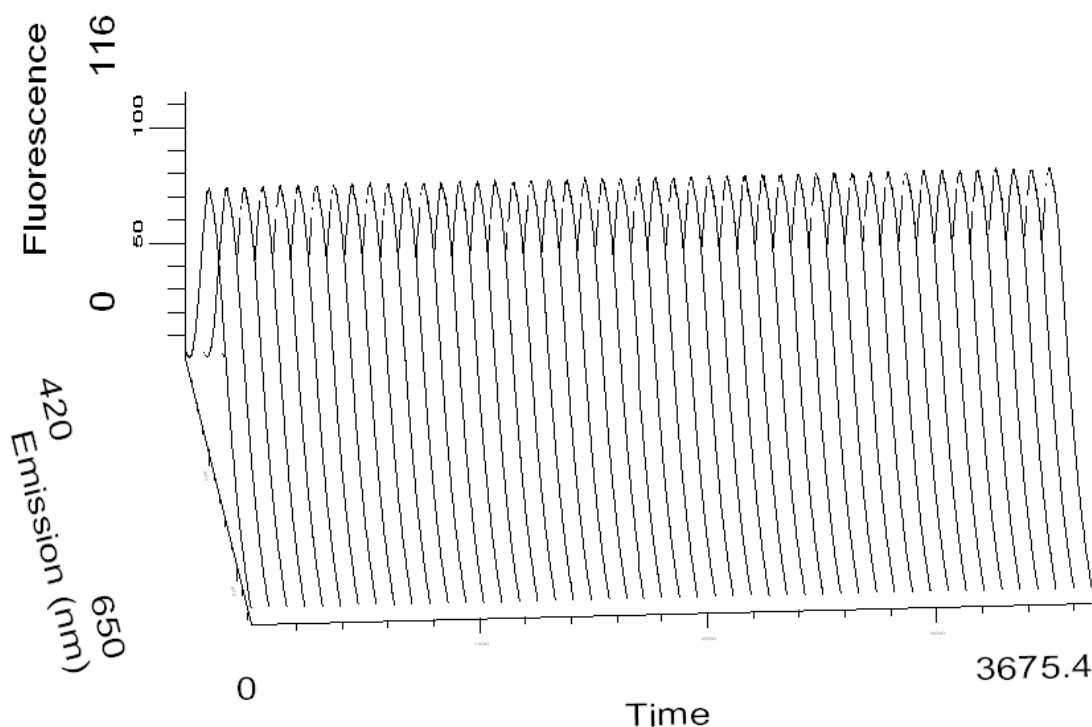
Obr. 26: 3D časové spektrum komplexu 2,22 \cdot 10^{-5} \text{ mol.l}^{-1} ( 1 \text{ } \mu\text{g.ml}^{-1} ) \text{Sc}^{3+} a 1,11 \cdot 10^{-4} \text{ mol.l}^{-1} 8-hydroxychinolin-5-sulfonové kyseliny, E = 740 \text{ V} a při pH 4,5. Obrázek odpovídá obr. 25 je snímán z jiné perspektivy.
