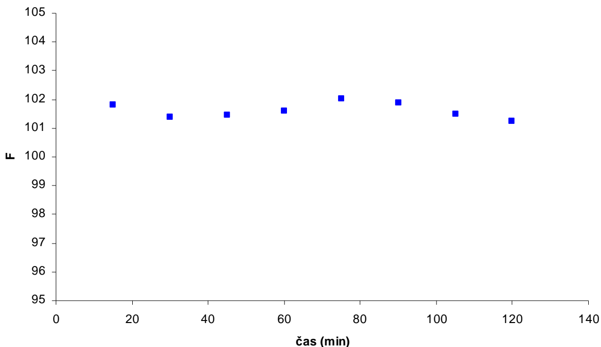
Obr. 24: Časová závislost fluorescence komplexu 2,22 \cdot 10^{-5} \text{ mol.l}^{-1} ( 1 \mu\text{g.ml}^{-1} ) \text{Sc}^{3+} a 1,11 \cdot 10^{-4} \text{ mol.l}^{-1} 8-hydroxychinolin-5-sulfonové kyseliny, E = 730 \text{ V} a při \text{pH } 4,5 .
