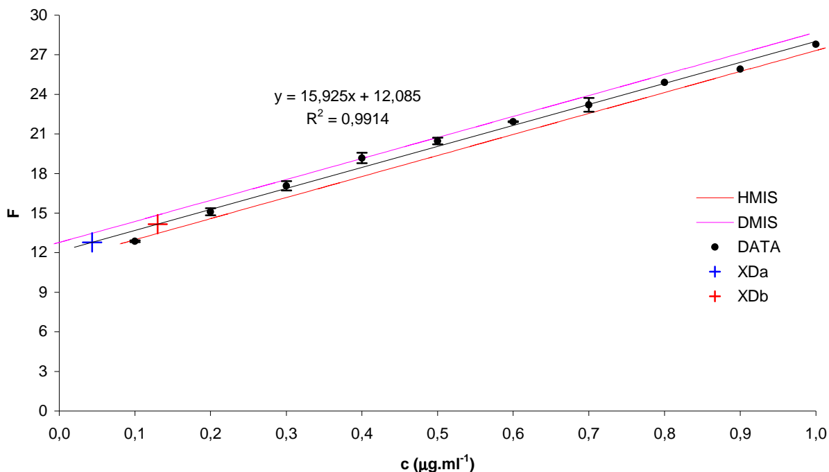
Obr. 59: Kalibrační závislost s intervaly spolehlivosti pro 0,1 - 1 \mu\text{g}\cdot\text{ml}^{-1} \text{Sc}^{3+} a lumogallionu 1,11 \cdot 10^{-4} \text{mol}\cdot\text{l}^{-1} při \text{pH} = 5 a E = 845 \text{ V} .
