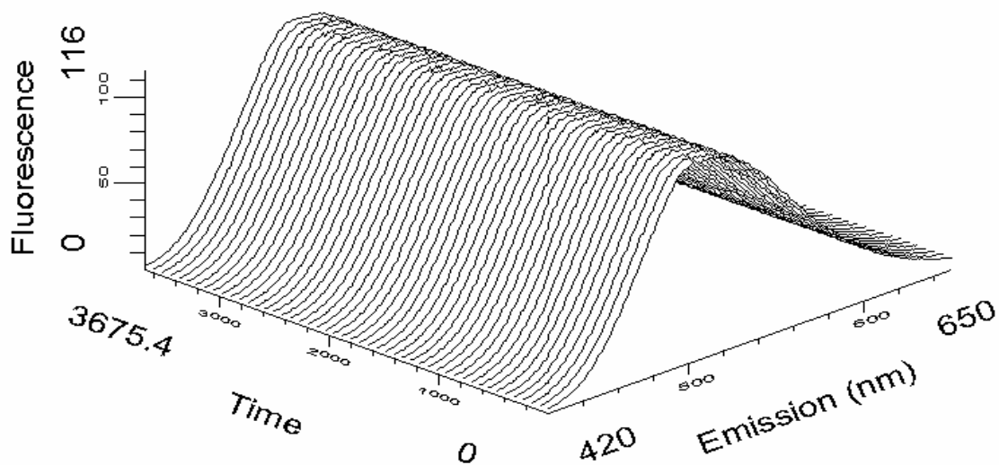
Obr. 25: 3D časové spektrum komplexu pro 2,22 \cdot 10^{-5} \text{ mol.l}^{-1} ( 1 \text{ } \mu\text{g.ml}^{-1} ) \text{Sc}^{3+} a 1,11 \cdot 10^{-4} \text{ mol.l}^{-1} 8-hydroxychinolin-5-sulfonové kyseliny, E = 740 \text{ V} a při pH 4,5.
