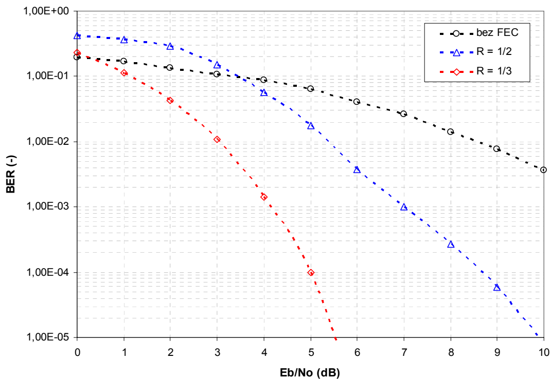
Obr. 3.10. Závislost BER na poměru E_b/N_0 pro různé kódové poměry, činitel rozptření SF = 128, 300000 přenesených bitů.
