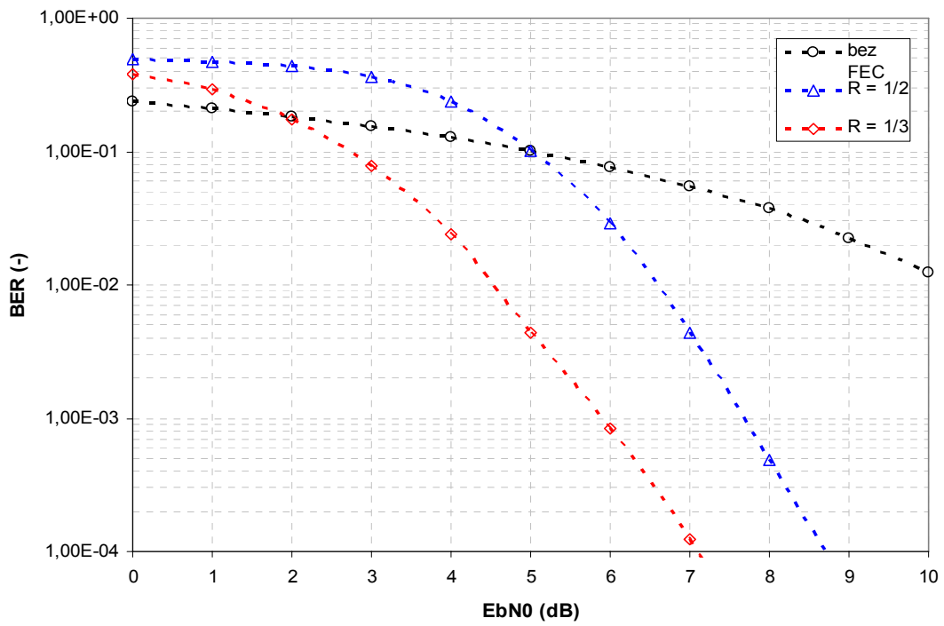
Obr. 3.6. Závislost BER na poměru E_b/N_0 pro různé kódové poměry, činitel rozprostření SF = 8, 4800000 přenesených bitů.
