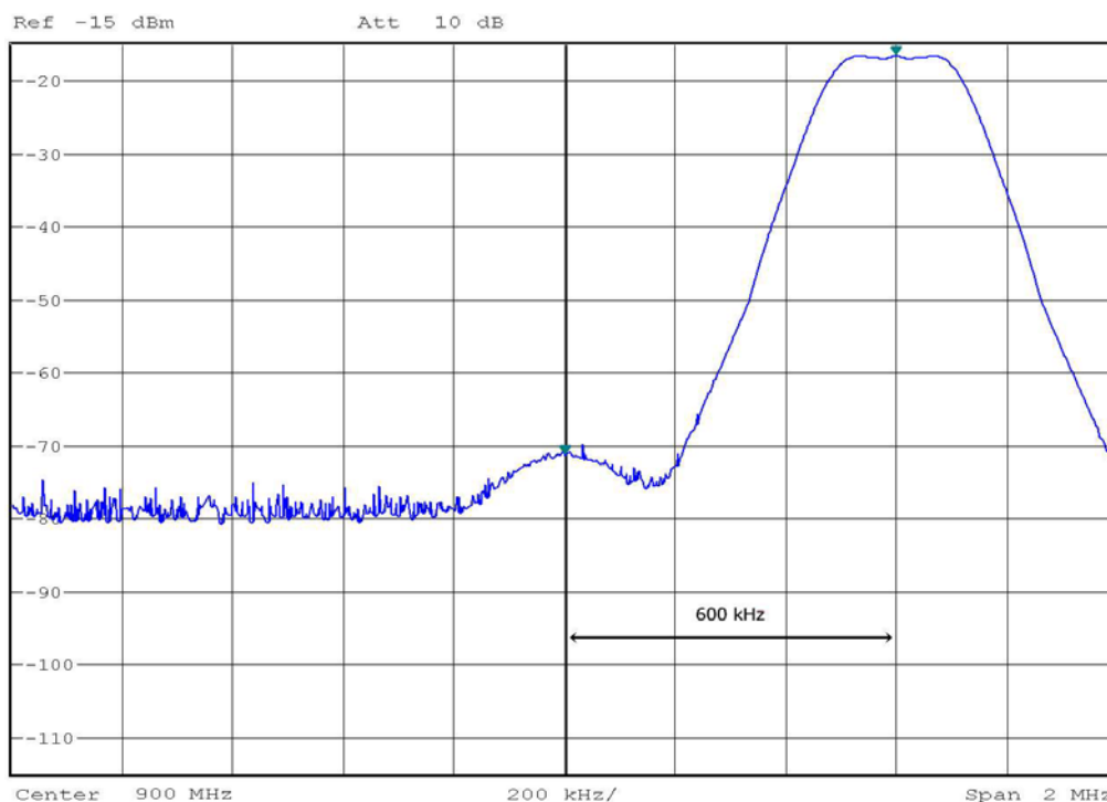
Obr. 5.13. Spektrum užitečného (vlevo) a silného interferujícího (vpravo) GSM - EDGE signálu na společném kanálu (Adjacent Channel Interference). Užitečný signál má minimální požadované CNR = 9 dB, interferenční signál je větší o 55 dB (hranice pro dosažení BER = 10^{-3} ).
