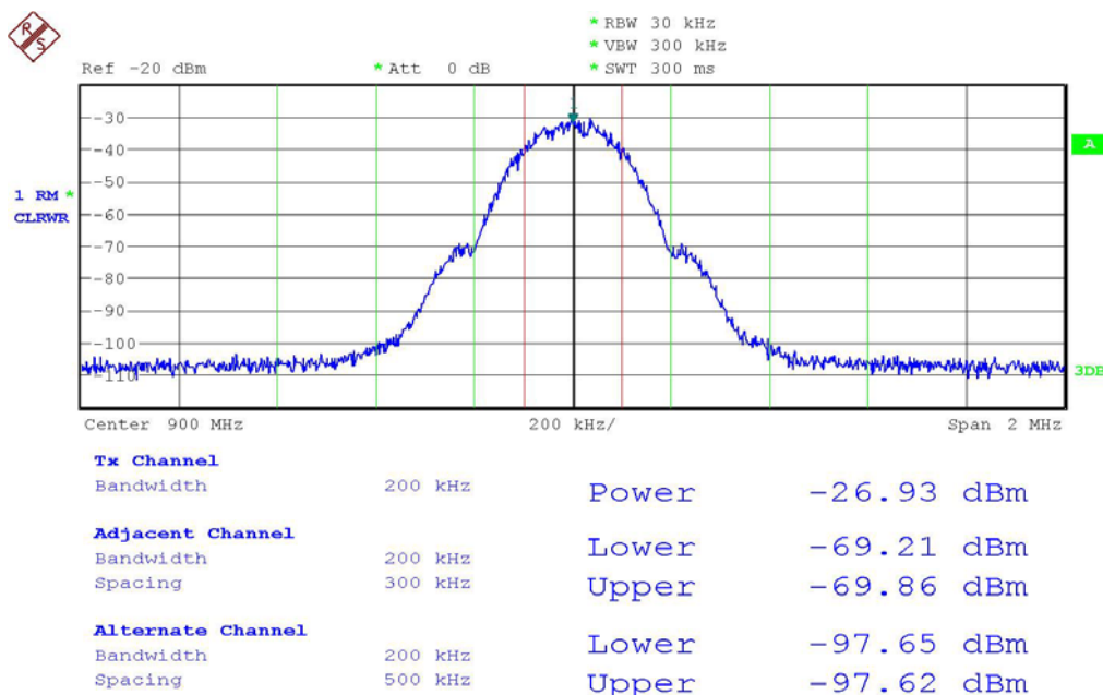
Obr. 5.6. Měření ACLR GSM - EDGE (modulace 8-PSK, MCS-5 – 9).
