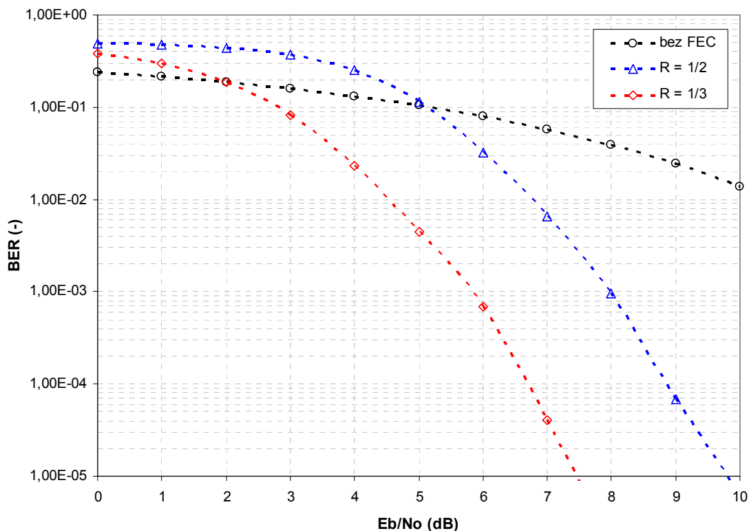
Obr. 3.5. Závislost BER na poměru E_b/N_0 pro různé kódové poměry, činitel rozptření SF = 4, 9600000 přenesených bitů.
