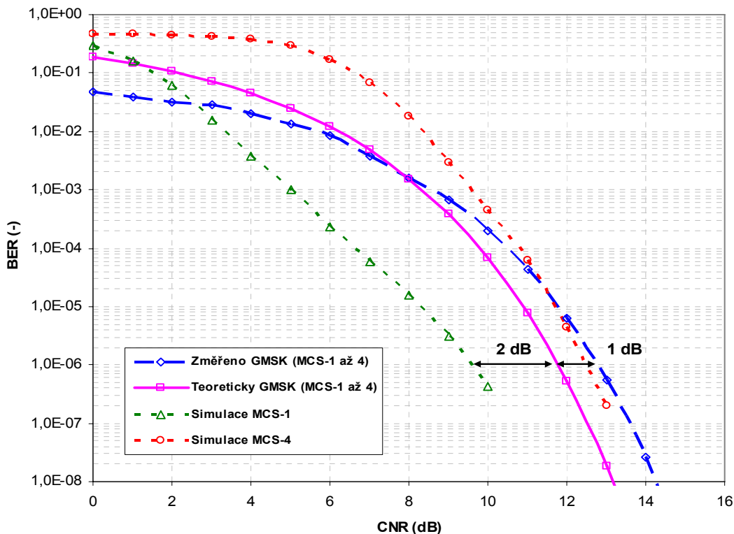
Obr. 5.5. Srovnání změřených a simulovaných hodnot závislosti BER na CNR, modulace GMSK, kanál AWGN.
