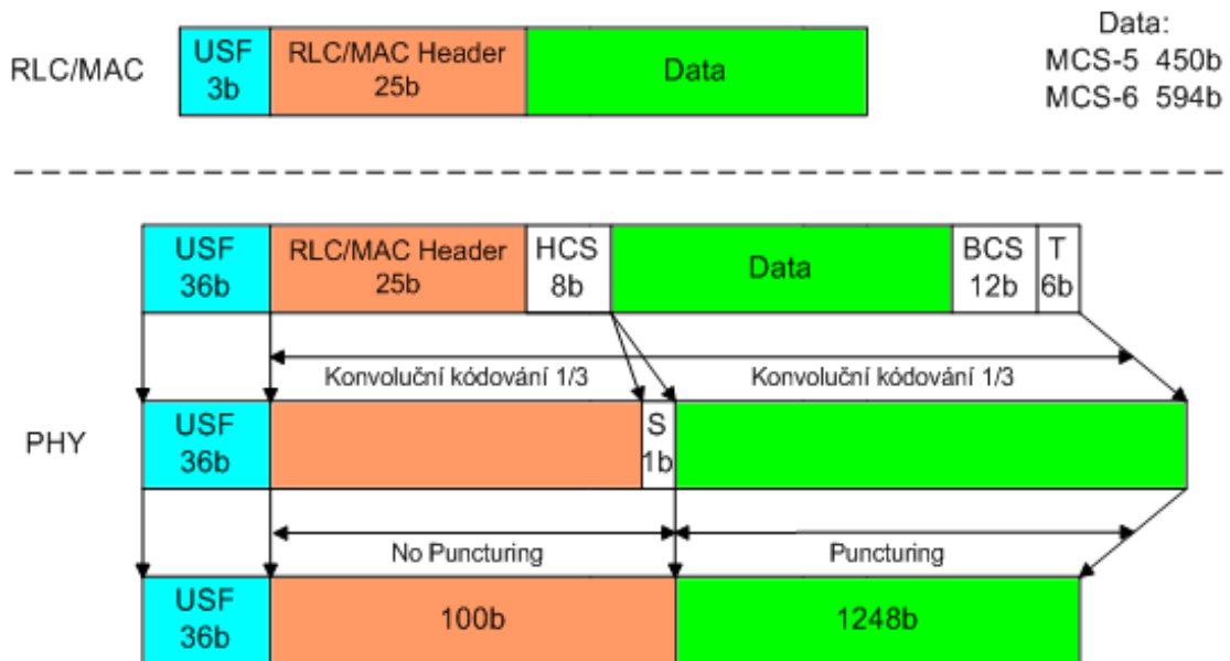
Obr. 2.7. Kódování dat pro schémata MCS-5 a MCS-6.
