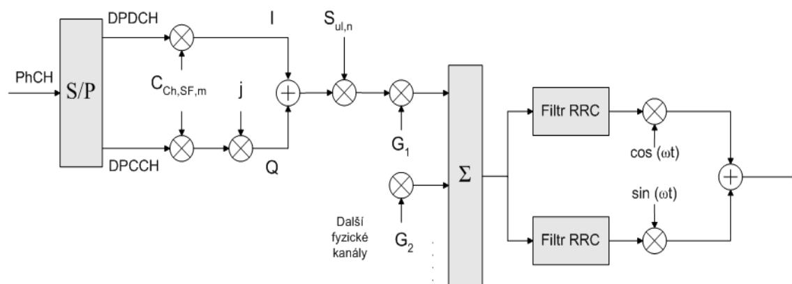
Obr. 2.27. Mapování, rozprostírání, skramblování, slučování kanálů a modulace UMTS v downlinku.
