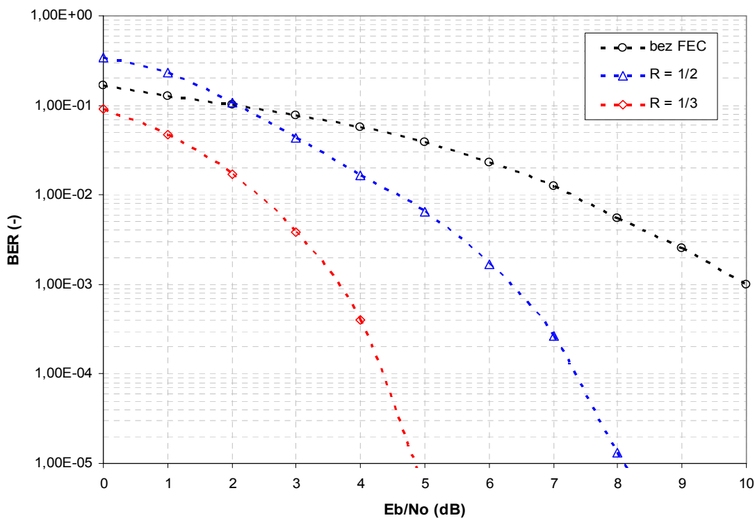
Obr. 3.11. Závislost BER na poměru E_b/N_0 pro různé kódové poměry, činitel rozptření SF = 256, 150000 přenesených bitů.
