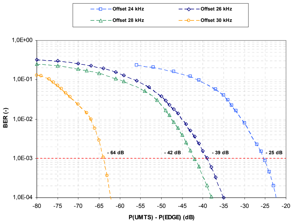
Obr. 4.13. Závislost bitové chybovosti BER na rozdílu úrovní užitečného signálu UMTS (referenční kanál 12,2 kb/s) a rušícího signálu GSM-EDGE a na vzdálenosti nosných.
