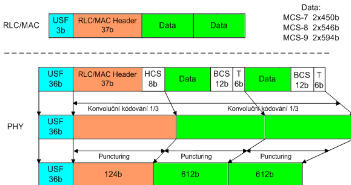
Obr. 2.10. Kódování dat pro schémata MCS-7 až MCS-9.
