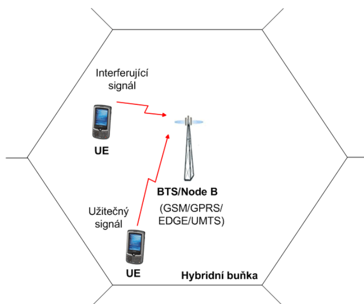
Obr. 5.17. Interferenční schéma (Inter-system Interference).
