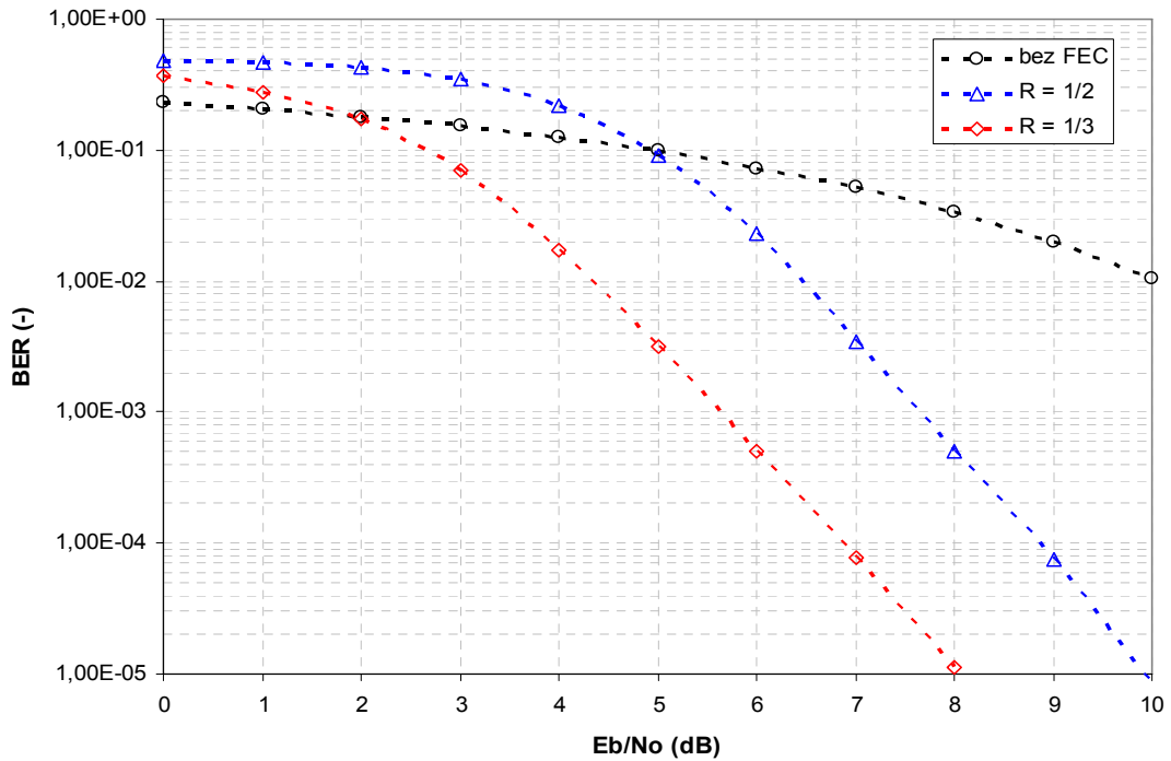
Obr. 3.7. Závislost BER na poměru E_b/N_0 pro různé kódové poměry, činitel rozprostření SF = 16, 2400000 přenesených bitů.
