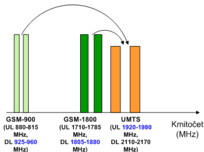
Obr. 1.1. Možné rušení systému UMTS systémem GSM.
