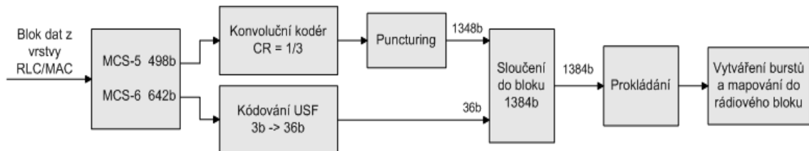
Obr. 2.9. Model kódování dat v základním pásmu (MCS-5 a MCS-6).
