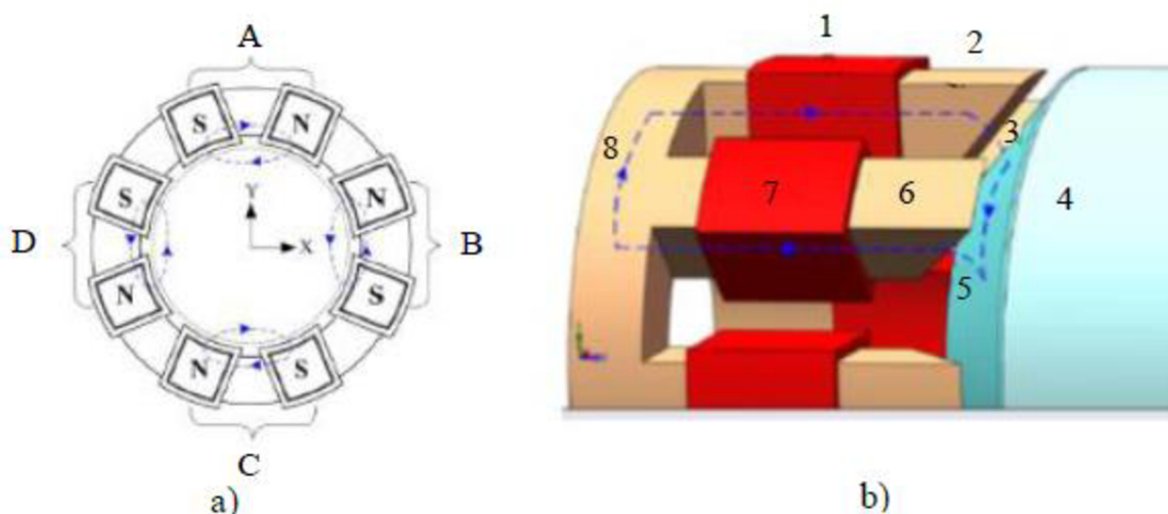
Obr. 2-11 Uspořádání pólů jedné strany magnetického ložiska, b) uzavírání magnetického toku v jedné pólové dvojici [1]
