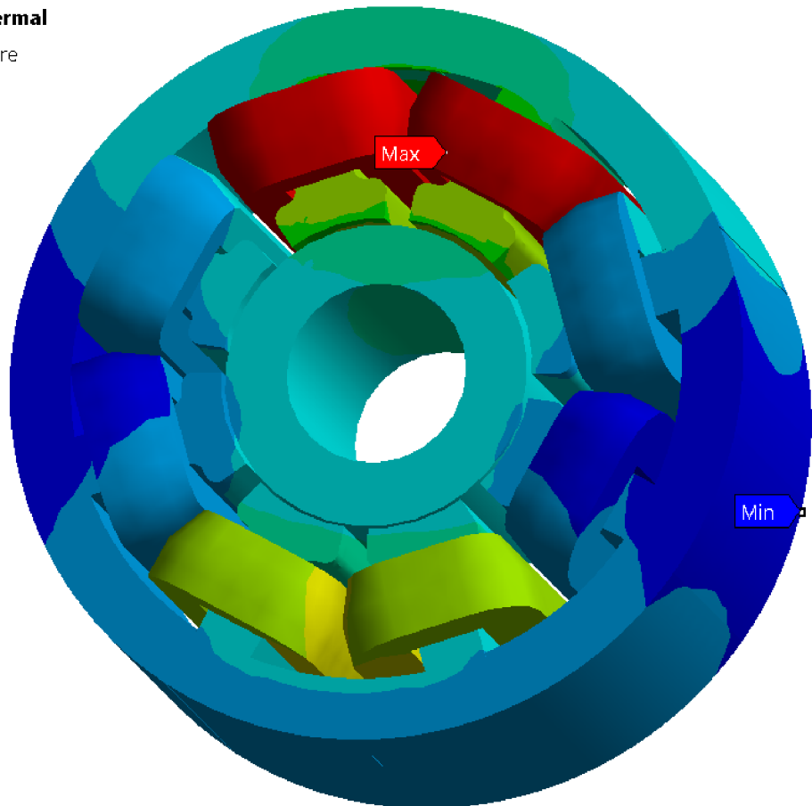
Obr. 7-2 Oteplení ložiska
