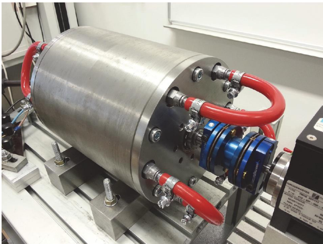
Obr. 5-1 Vysokootáčkový elektrický stroj pro návrh hybridního magnetického ložiska [19].
