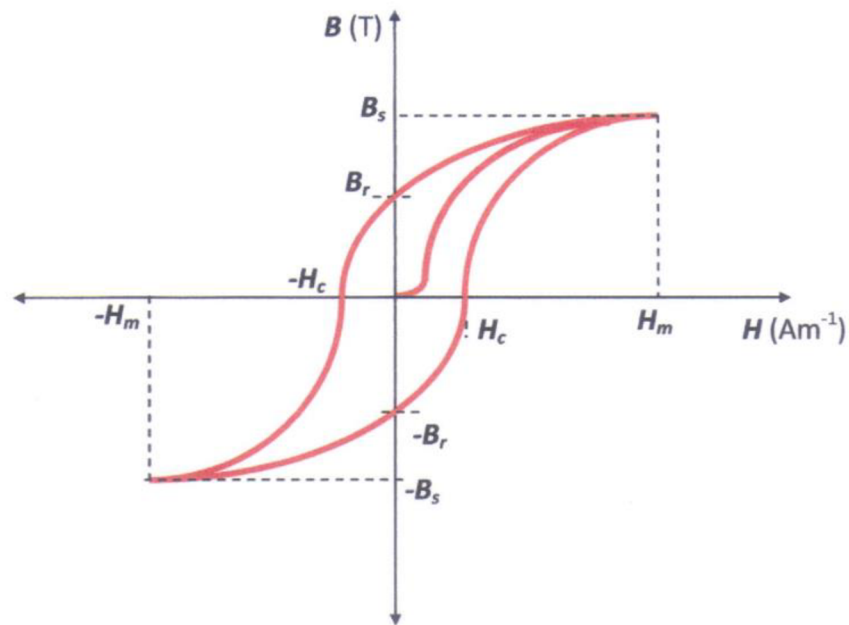
Obr. 5-2 Hysterézní smyčka [9]
