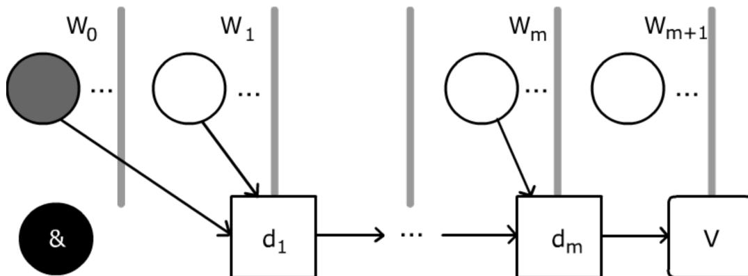
Obr. 3.1: Rozhodovacie okna [8, 15]
