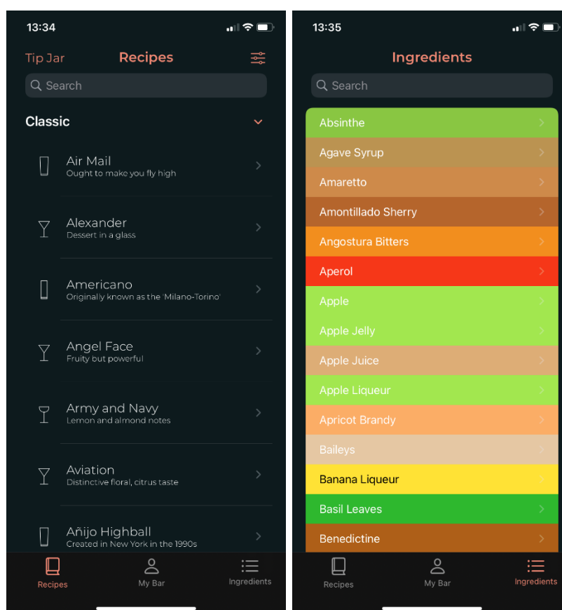
Obrázek 1- aplikace Imbible [31]
