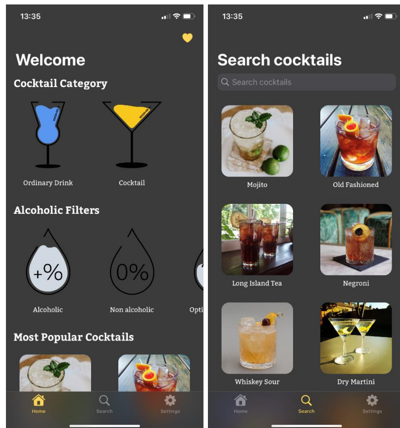
Obrázek 2 - aplikace CocktailHut [32]
