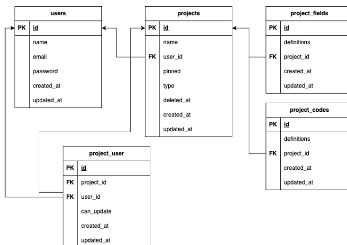
Obr. 5.9: Štruktúra databázy
