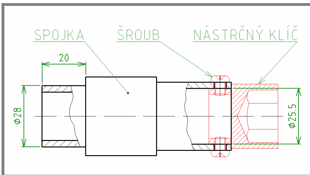
Obr. 3-1 Přípojovací rozměry
