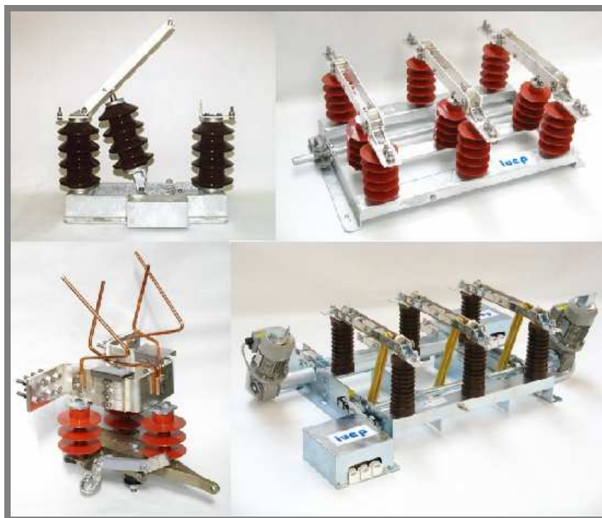
Obr. 1-3 Ukázka odpojovačů vysokého napětí firmy IVEP: venkovní jednopólový (vlevo nahoře), venkovní trojité (vpravo nahoře), venkovní trakční (vlevo dole), vnitřní trojité (vpravo dole) [6]
