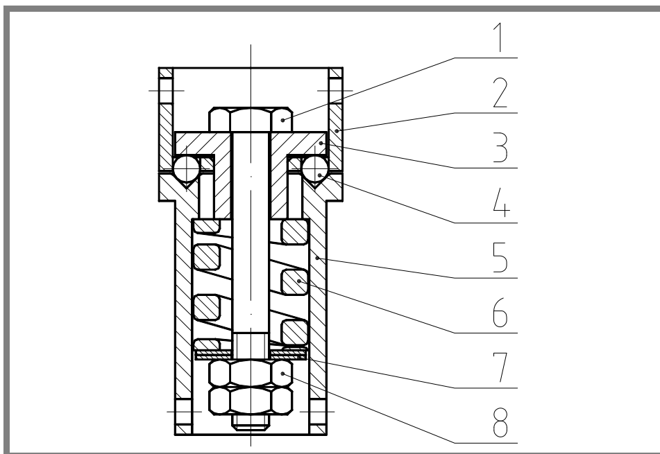
Obr. 5-7 Návrh konstrukce spojky – výsledná varianta: 1-šroub; 2-unašeč; 3-přítlačník; 4-kulička; 5-přířuba; 6-pružina; 7-podložky pružiny; 8-nastavovací matice
