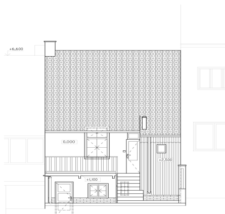
Obrázek 5 - Pohled uliční po přestavbě
