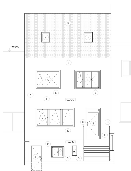
Obrázek 7 - Pohled dvorní po přestavbě
