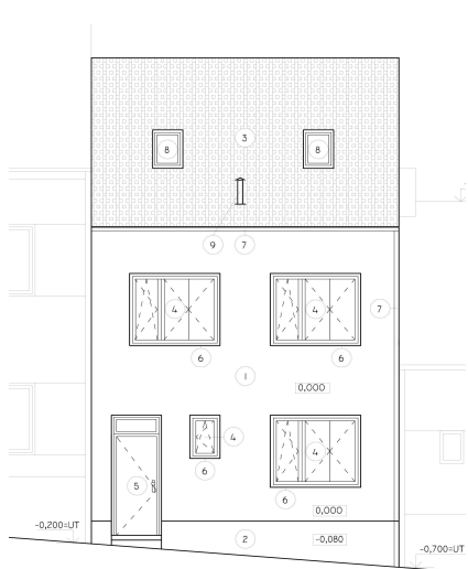
Obrázek 6 - Pohled uliční po přestavbě
