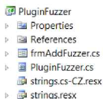
Obrázek 8-10: PluginFuzzer
