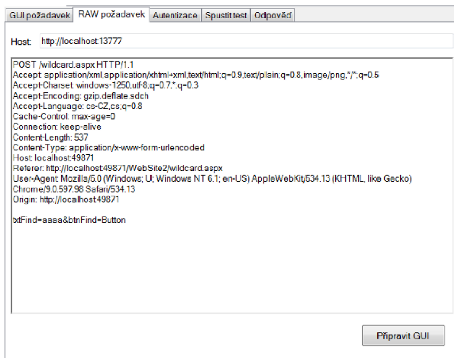
Obrázek 8-15: RAW požadavek
