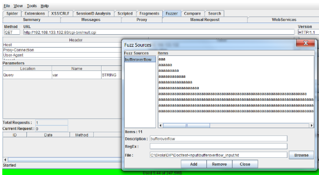
Obrázek 5-6: WebScarab – fuzzer
