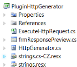
Obrázek 8-7: PluginHTTPGenerator
