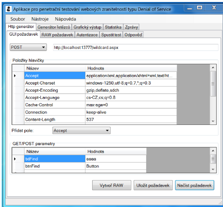
2-1: Http generátor
