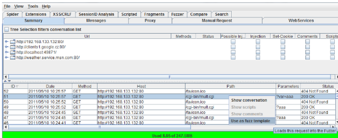
Obrázek 5-5: WebScarab – proxy
