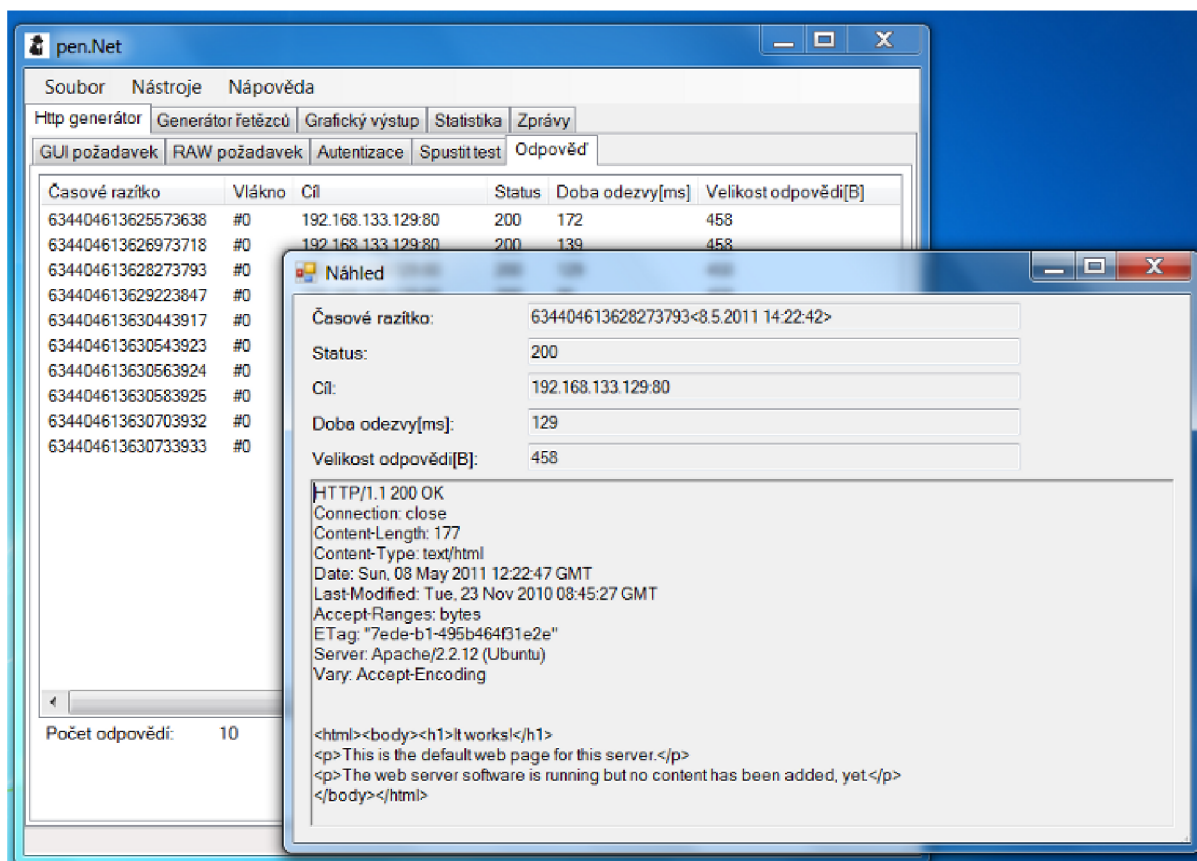
Obrázek 8-18: Odpověď
