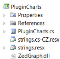
Obrázek 8-12: PluginCharts
