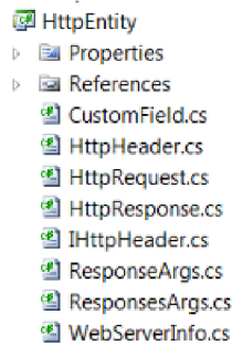
Obrázek 8-8: HTTPEntity
