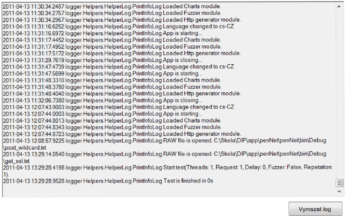
1-3: Zprávy
