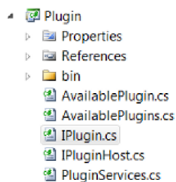
Obrázek 8-5: Plugin
