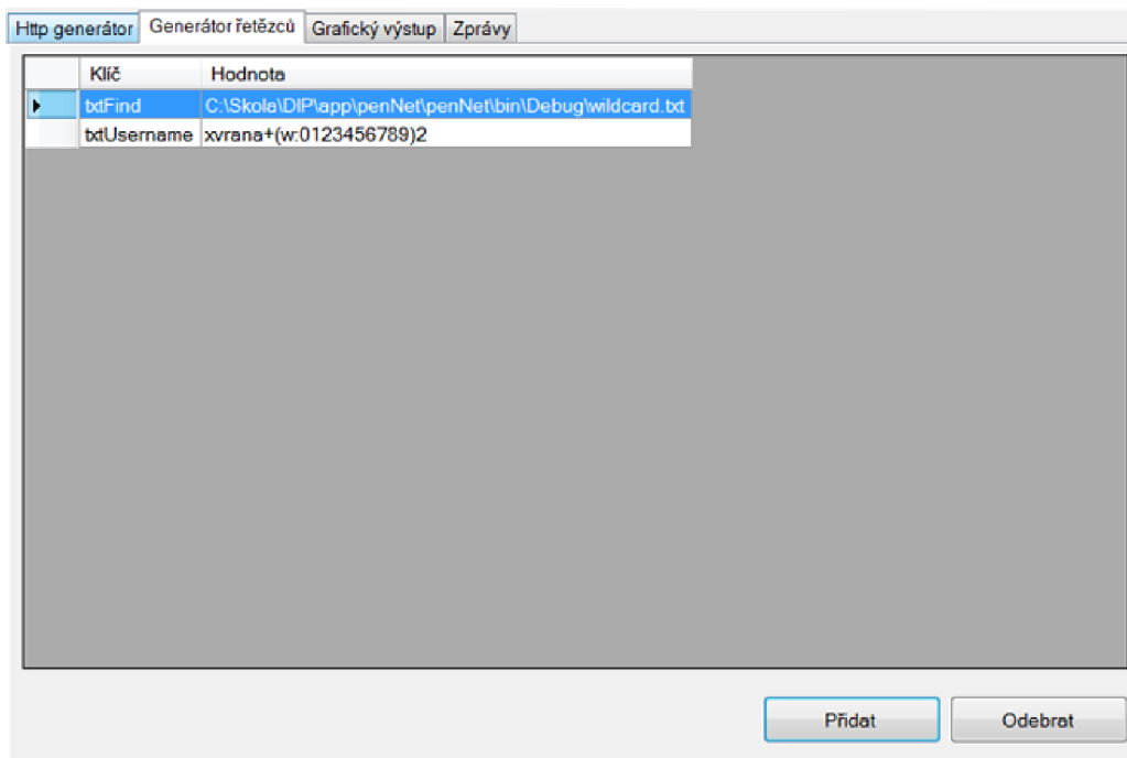
3-1: Generátor řetězců
