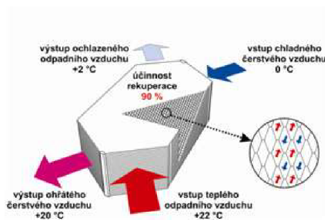
Obr. 12 Deskový rekuperační výměník [6]
