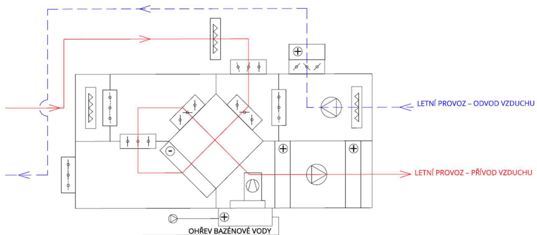
Obr. 41 Provozní režim v letním období
