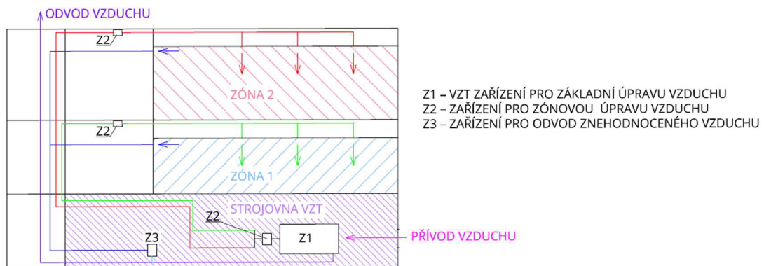
Obr. 8 Znáznornění zónového vzduchového systému
