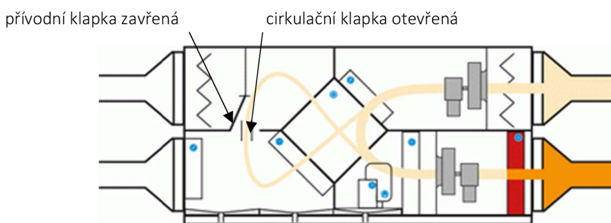
Obr. 49 Schéma – cirkulační režim
