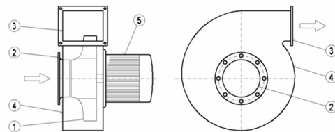
Obr. 22 Radiální ventilátor se spirální skříň [10]
