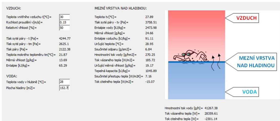
Obr. 33 Výpočet vodních zisků
