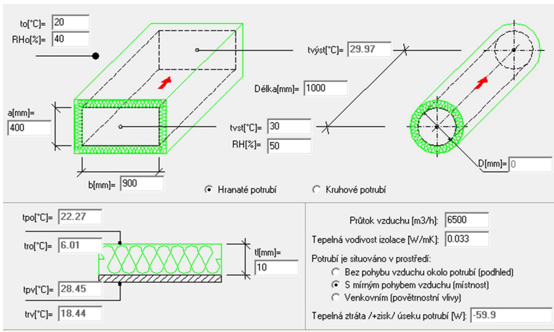
Obr. 48 Zimní období – sání vzduchu z prostoru bazény, prostor strojovny
