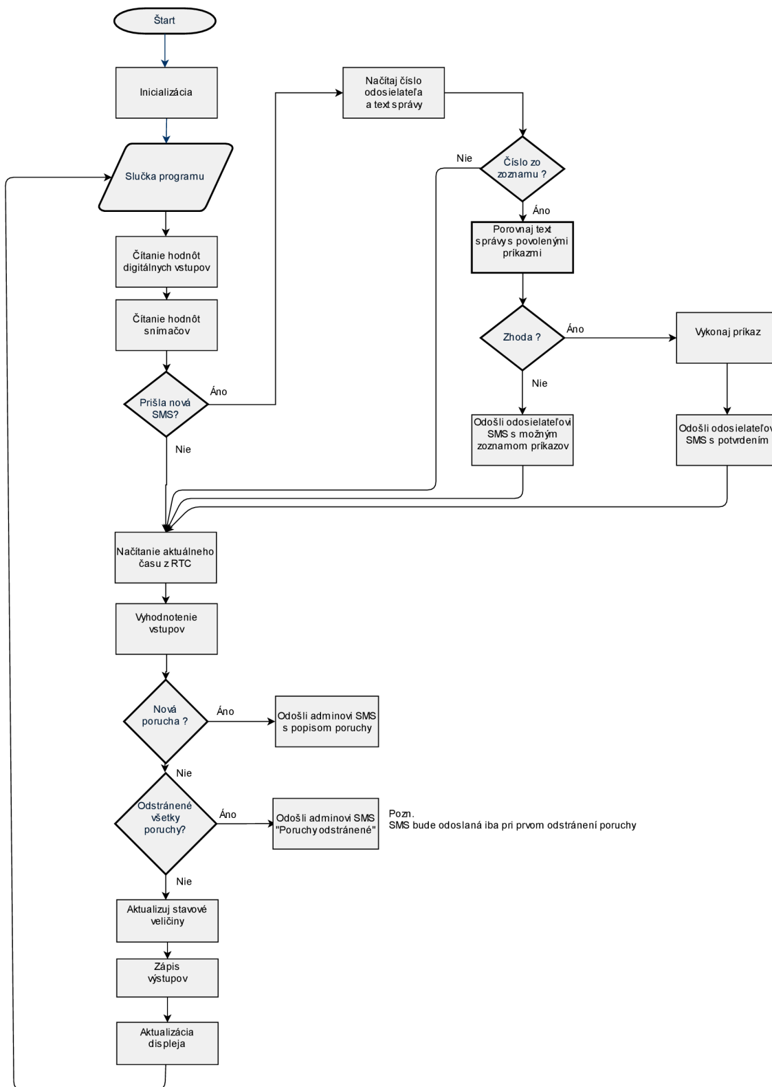
Obr. 17 Zjednodušený vývojový diagram implementovaného programu
