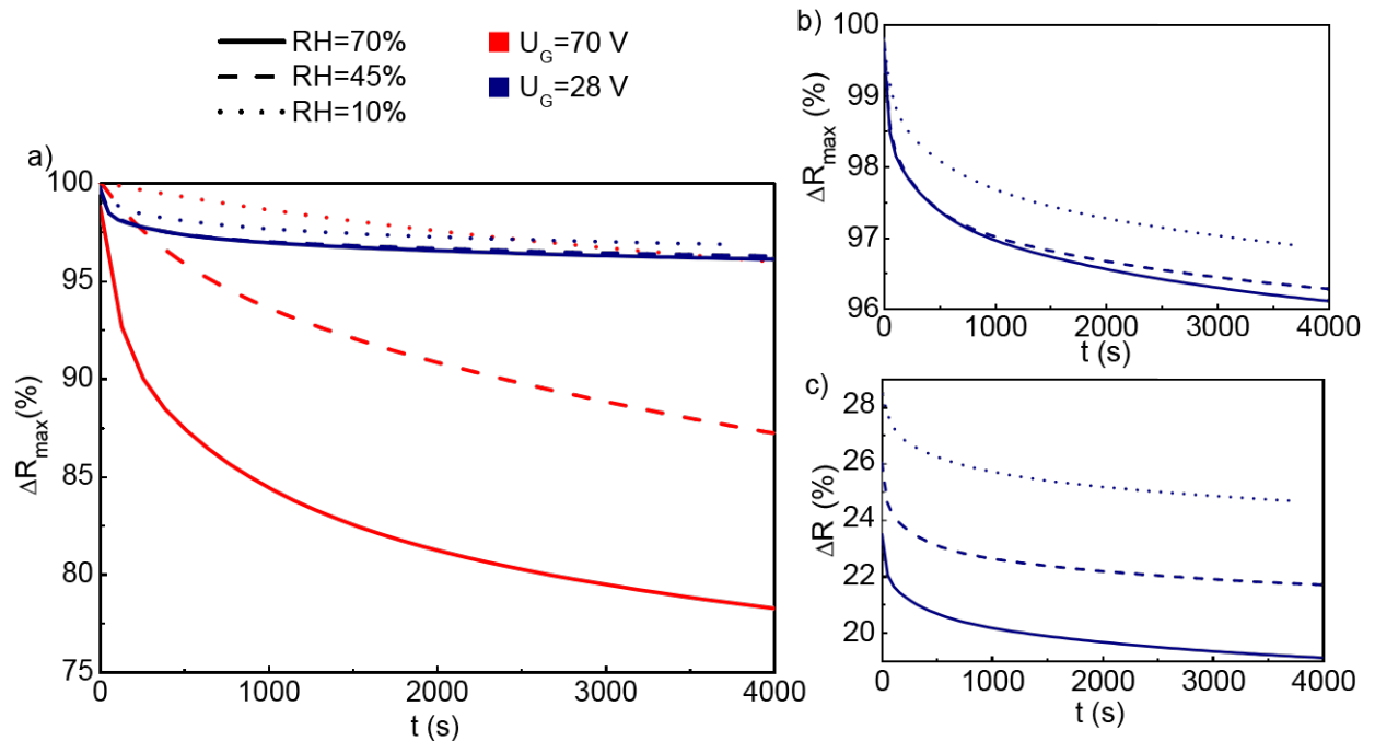
Obr. 4.5: a) Zmena odporu grafénu definovaná vzťahom \Delta R_{max}(t) = (R_{max} - R(t)) \cdot 100\%/R_{max} po priložení hradlového napätia 70 V (červené krivky) a 28 V (modré krivky) pri relatívnych vlhkostiach 10%, 45% a 70%, ktoré sú odlišené tvarom krivky. b) Detail grafu a) pre zmenu odporu po priložení hradlového napätia 28 V. c) Zmena odporu grafénu definovaná vzťahom \Delta R(t) = (R(t) - R(0)) \cdot 100\%/R(0) .
