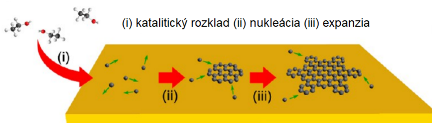
Obr. 2.7: Znárodnenie rastu grafénu pomocou chemickej depozície z plynnej fázy pri použití substrátu s nízkou hodnotou rozpustnosti uhlíka. Prevziate a upravené od [16].
