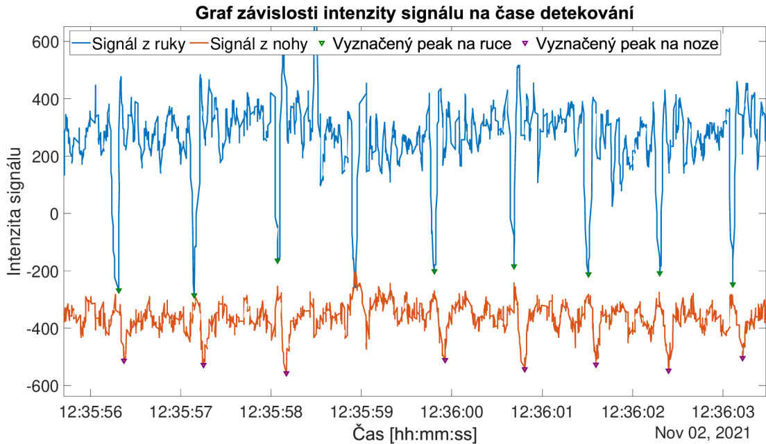
Obrázek 5.5: Znázornění vybraných křivek spolu se signifikantními peaky.
