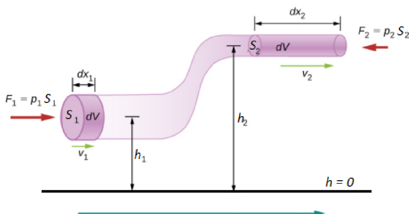
Obrázek 2.1: Bernoulliho rovnice proudění kapaliny v trubici o nesteržném průřezu [20] (upraveno).
