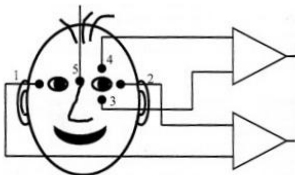
Obrázek 2 Rozmístění elektrod [1].
