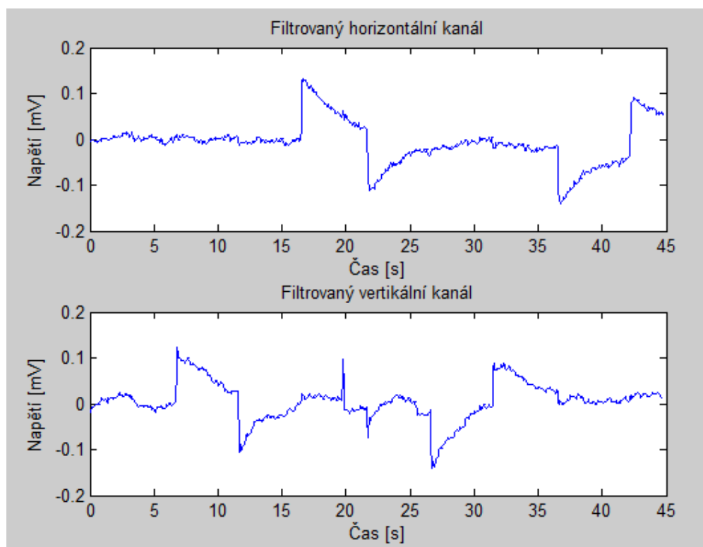
Obrázek 15 Filtrovaný signál.
