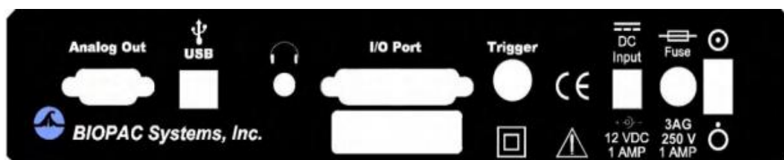
Obrázek 5 Zadní panel [2].
