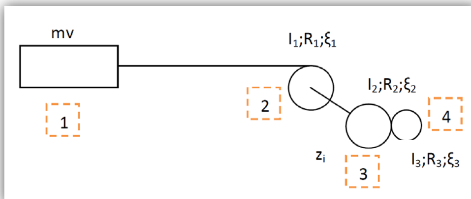
Obrázek 5.4: Jezdec - schéma
