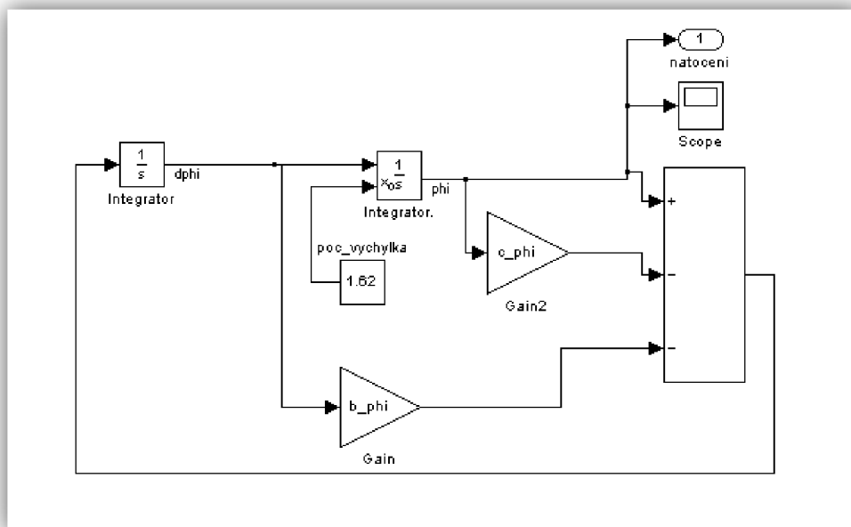
Obrázek 5.2: Simulinkové schéma kyvadla
