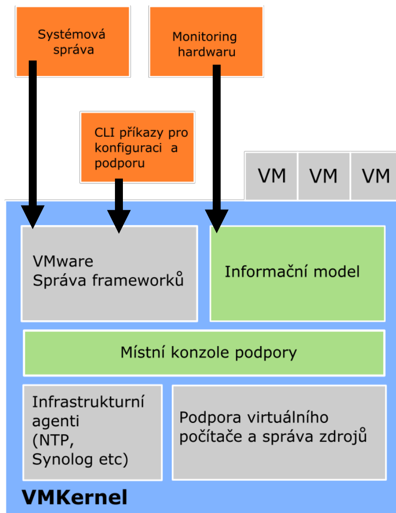
Obrázek 10 - Architektura ESXi
