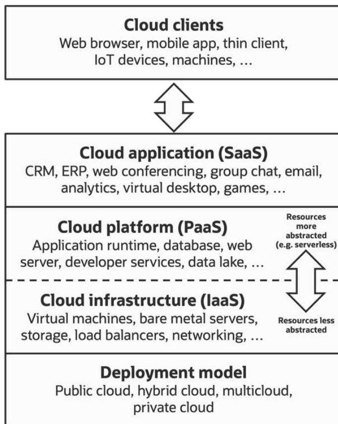
Obrázek 4 - Modely služeb cloud computingu uspořádané jako vrstvy
