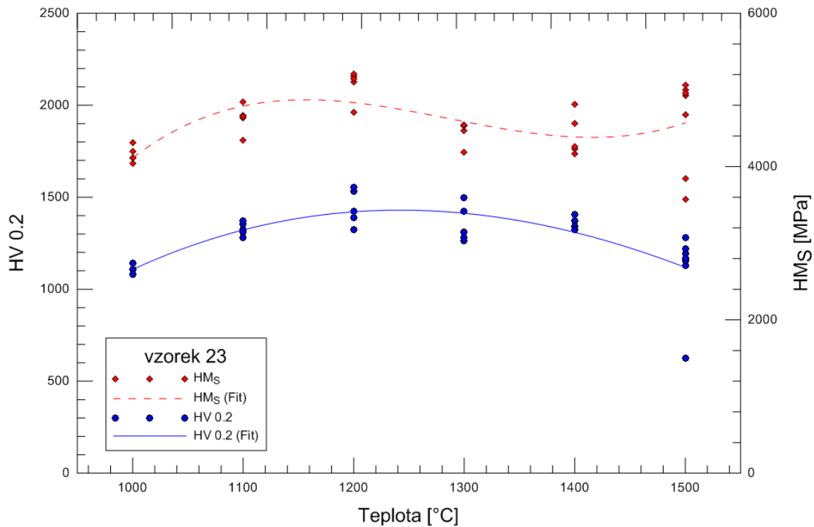
Graf 5.9: Závislost HV\ 0.2 a HM_S na teplotě žíhání pro vzorek matrice č. 23.
