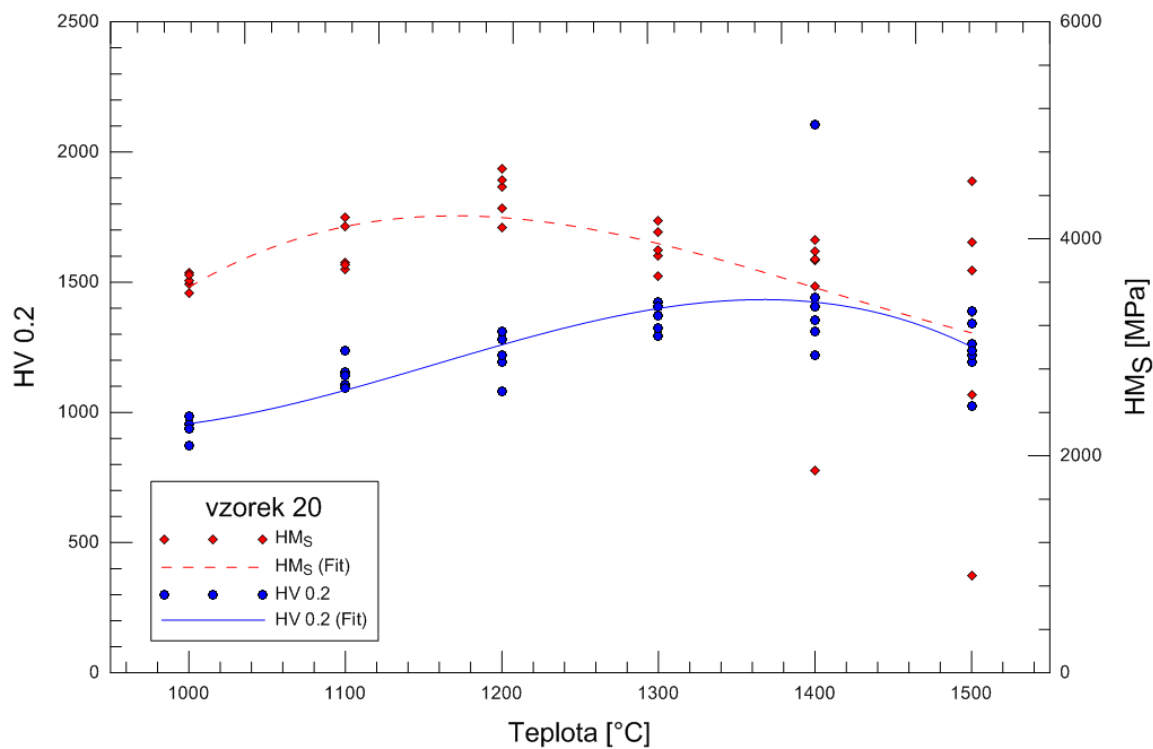
Graf 5.7: Závislost HV 0.2 a HMS na teplotě žhání pro vzorek matrice č. 20.
