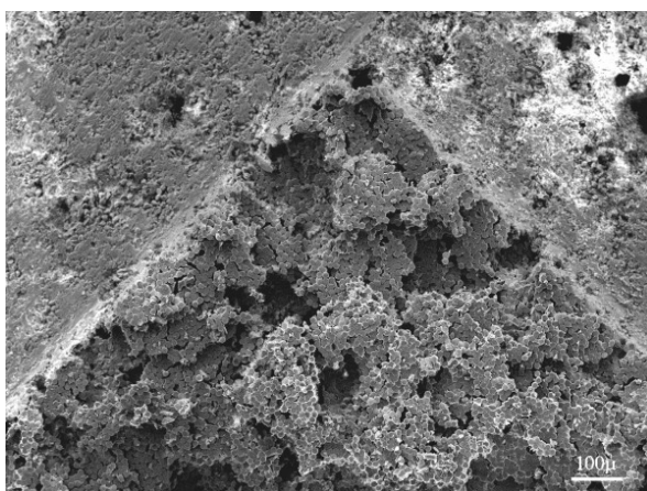
Obrázek 5.15: Charakteristický lomový reliéf v místě vzniku trhliny typický pro zkoumané kompozity (vlevo) a detail (vpravo).
