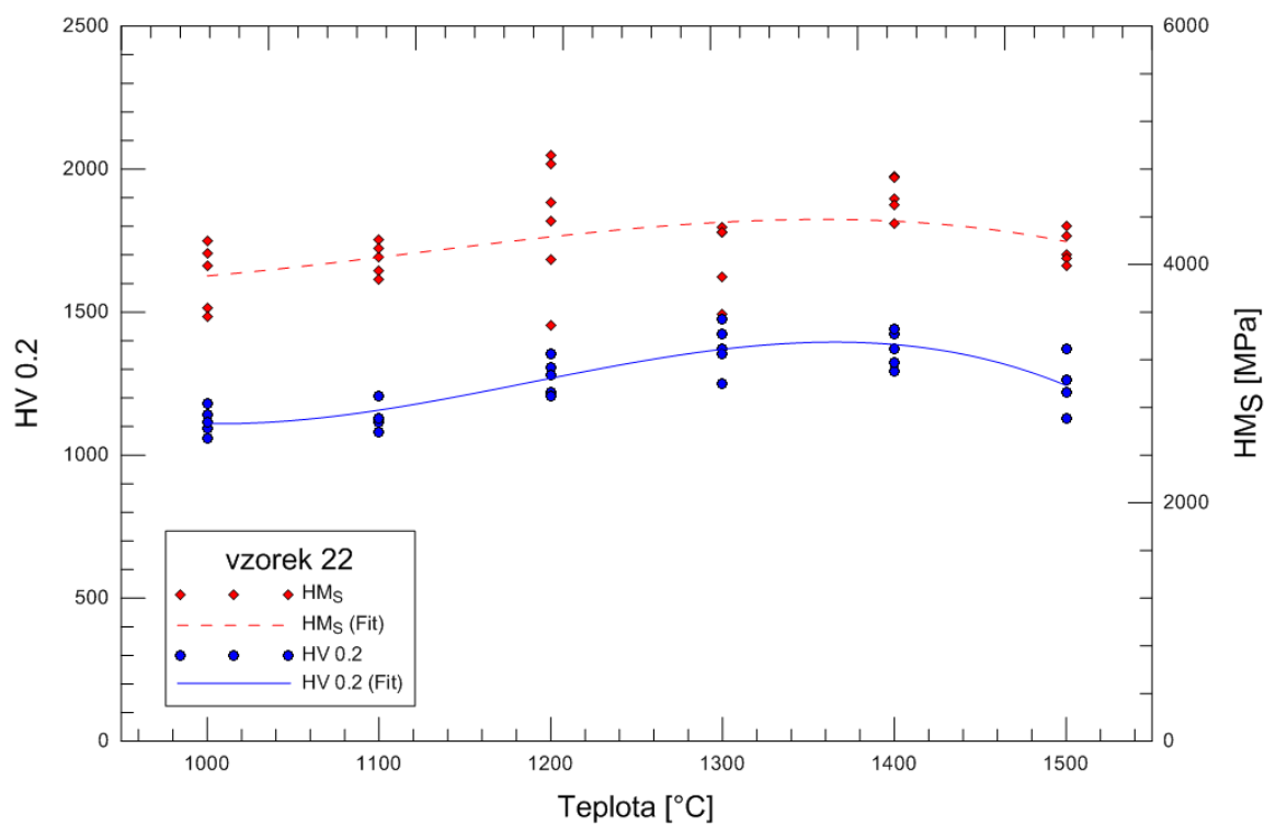
Graf 5.8: Závislost HV 0.2 a HMS na teplotě žhání pro vzorek matrice č. 22.
