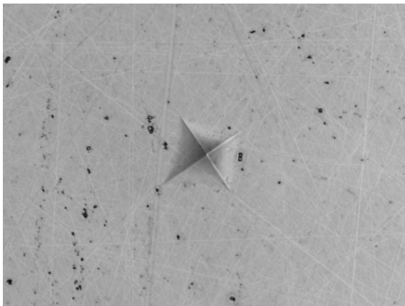
Obrázek 5.5: Typický asymetrický vpich pro vzorek matrice č. 29 způsobený nerovnoběžností podstavy s rovinou výbrusu.
