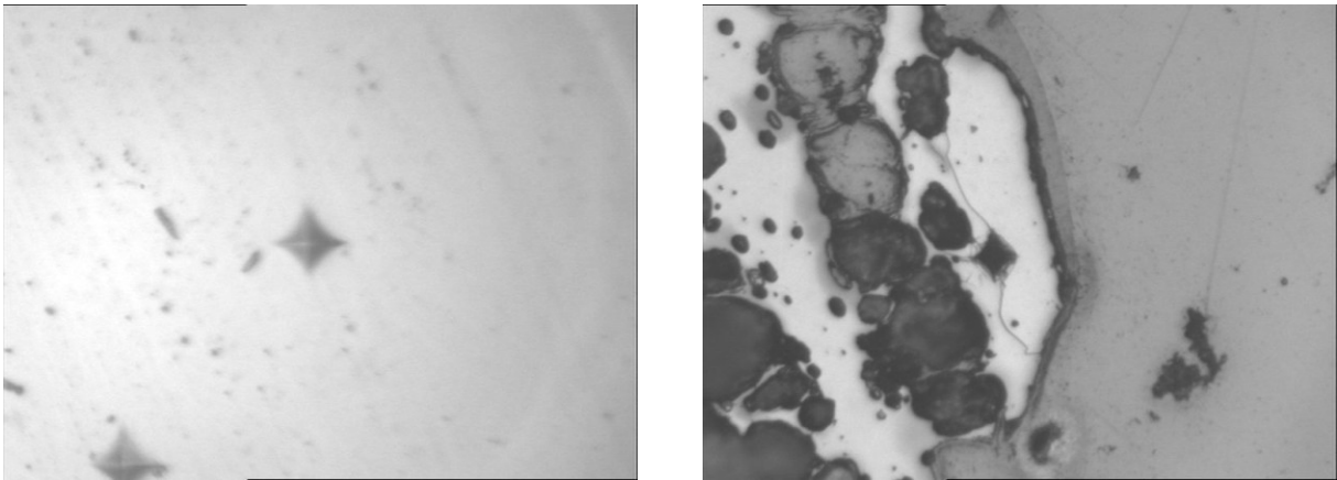
Obrázek 2.10: Vpich diamantovým hrotem do matrice, vpravo ukázka poškozeného vpichu. Zvětšení obou vpichů je 600×.
