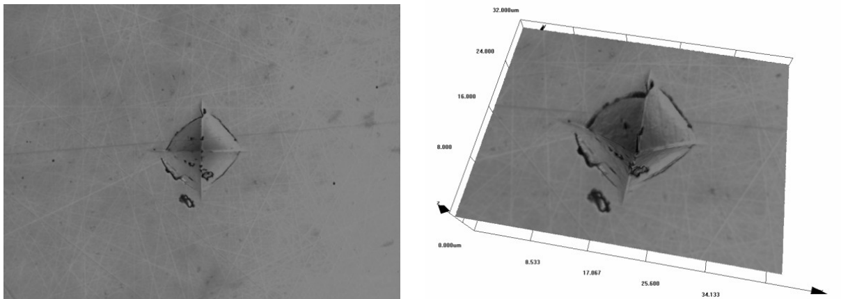
Obrázek 5.6: Charakteristický vpich pro vzorek matrice č. 30 pyrolyzovaný při teplotě 1000 °C.
