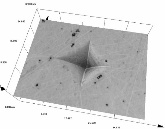
Obrázek 5.5: Typický asymetrický vpich pro vzorek matrice č. 29 způsobený nerovnoběžností podstavy s rovinou výbrusu.
