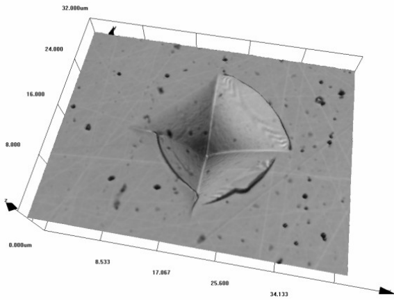
Obrázek 5.4: Vzorek č. 28, viditelná pórovitost matrice žíhané při teplotě 1100 °C, vpravo poškozené hrany vpichu u matrice žíhané při teplotě 1300 °C.
