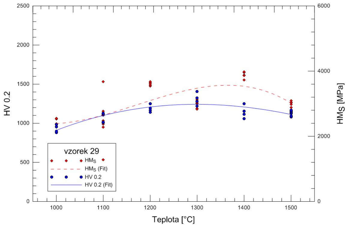
Graf 5.14: Závislost HV 0.2 a H_M na teplotě žhání pro vzorek matrice č. 29.
