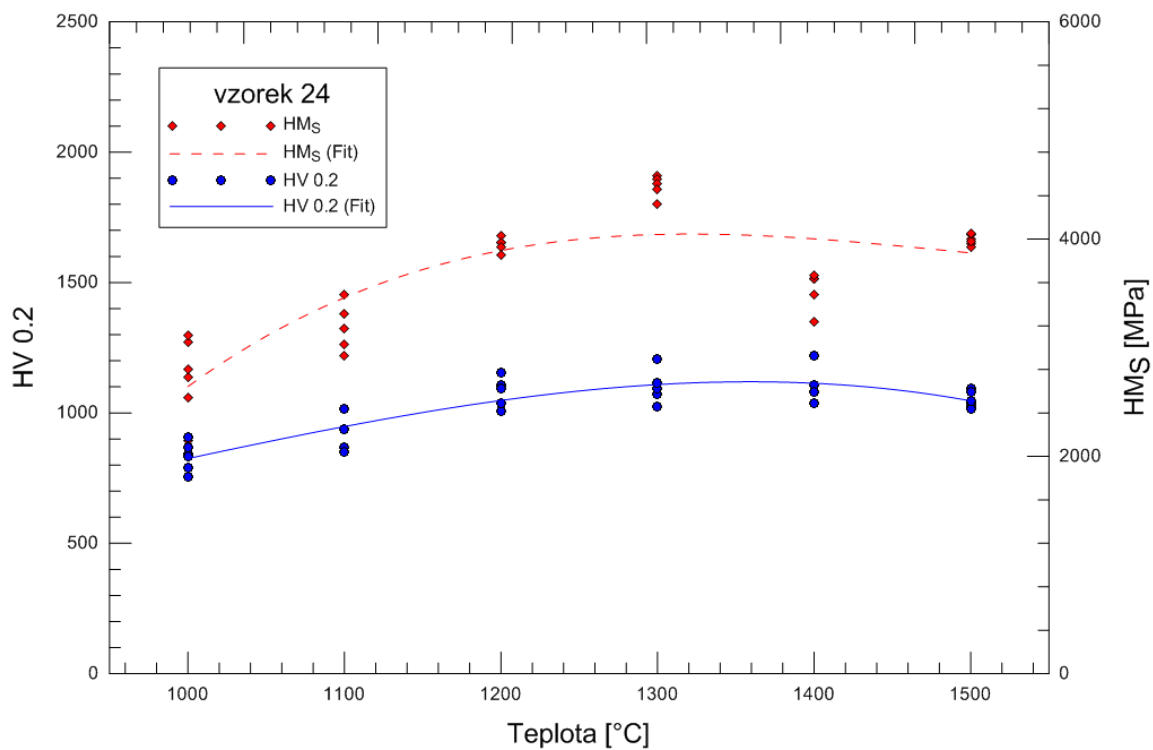
Graf 5.10: Závislost HV\ 0.2 a HM_S na teplotě žíhání pro vzorek matrice č. 24.
