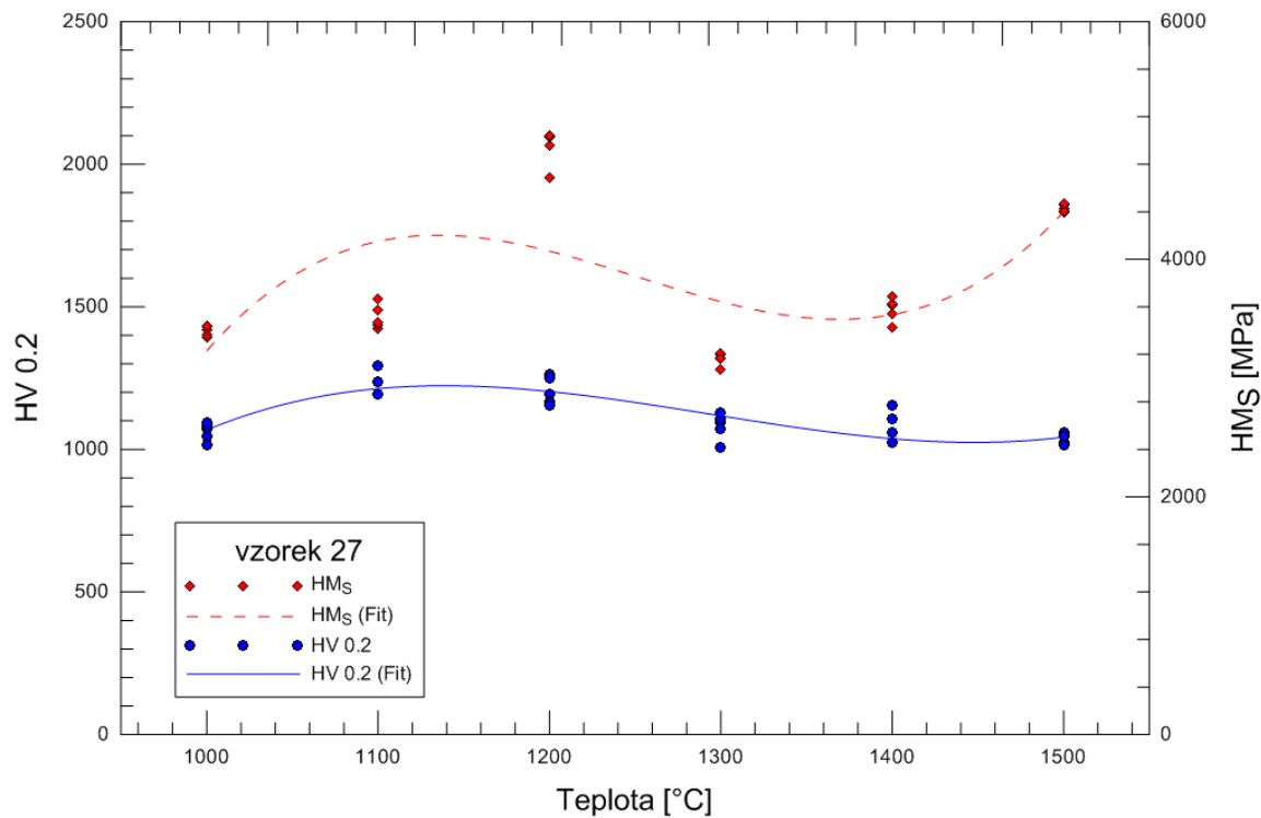
Graf 5.12: Závislost HV 0.2 a HM_S na teplotě žíhání pro vzorek matrice č. 27.
