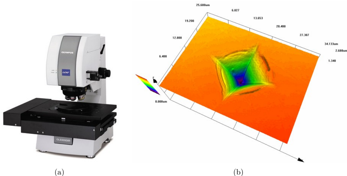
Obrázek 4.10: Konfokální mikroskopie. (a) Olympus LEXT OLS 3100 s AFM modulem 2 , (b) 3D rekonstrukce vpichu pomocí dat získaných z konfokálního mikroskopu.
