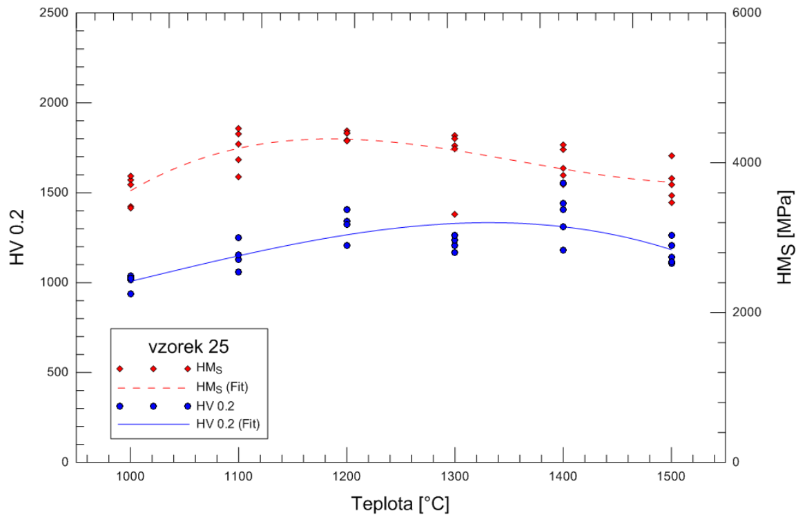
Graf 5.11: Závislost HV 0.2 a HM_S na teplotě žíhání pro vzorek matrice č. 25.
