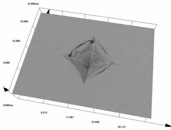
Obrázek 5.3: Charakteristický vpich pro vzorek č. 27.
