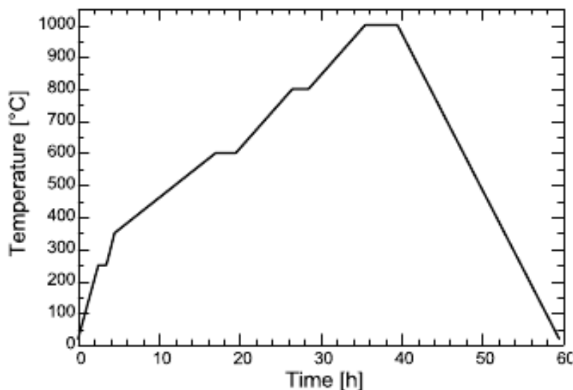
Obrázek 4.2: Teplotní profil pyrolýzy polysiloxanových matric [31].
