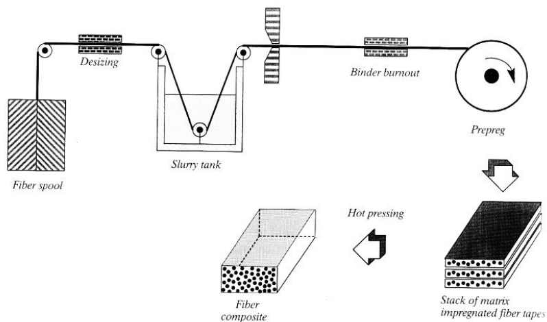
Obrázek 2.6: Namáčení vláken do kompozitní matrice [7].
