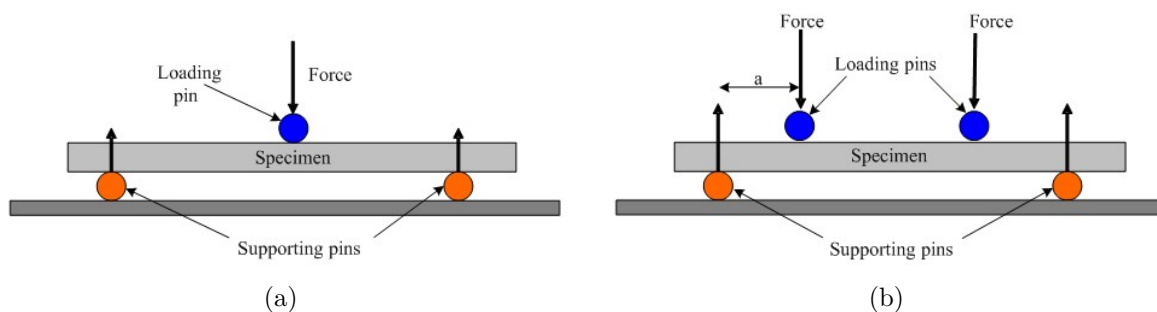
Obrázek 2.12: Ohybový test. (a) Třibodový ohyb, (b) čtyřbodový ohyb [28].
