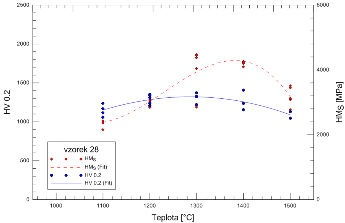
Graf 5.13: Závislost HV 0.2 a H_M na teplotě žhání pro vzorek matrice č. 28.
