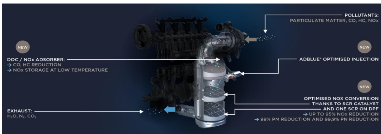
Obr. 42 Způsob snižování emisí motoru 1.5 BlueHDI [61]
