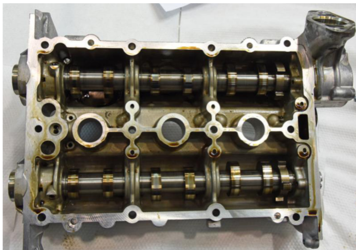
Obr. 26 Pohled na viko hlavy válců s řešením pro úchyt čerpadla (pravý roh vika) [39]
