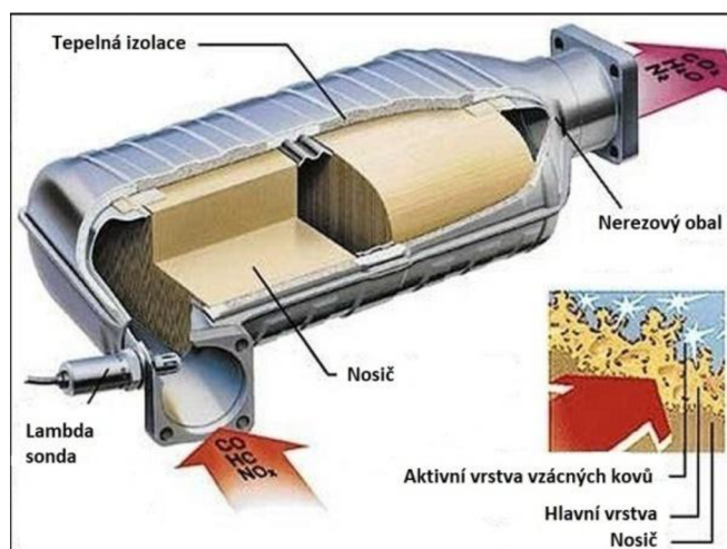
Obr. 13 Řez třicestným řízeným katalytickým konvertorem [20]
