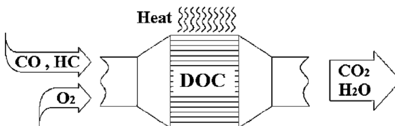
Obr. 20 Oxidační katalytický konvertor pro vznětové motory [28]
