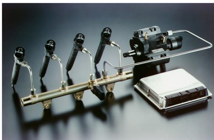
Obr. 15 Soustava vysokotlakého okruhu vstříkovaní systému Common rail [23]
