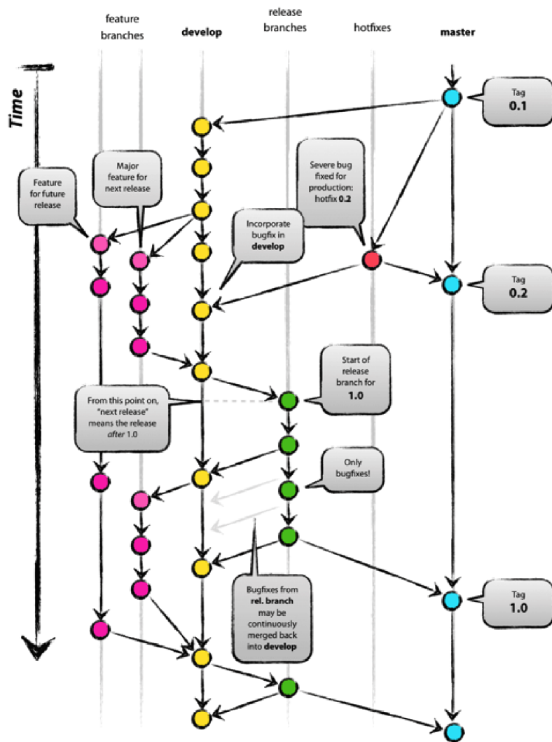
Obrázek 3.3: Gitflow workflow
