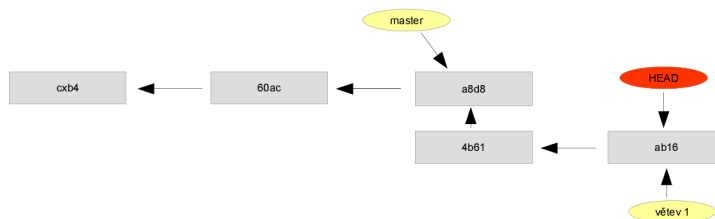
Obrázek 2.5: Git práce v nové větvi
