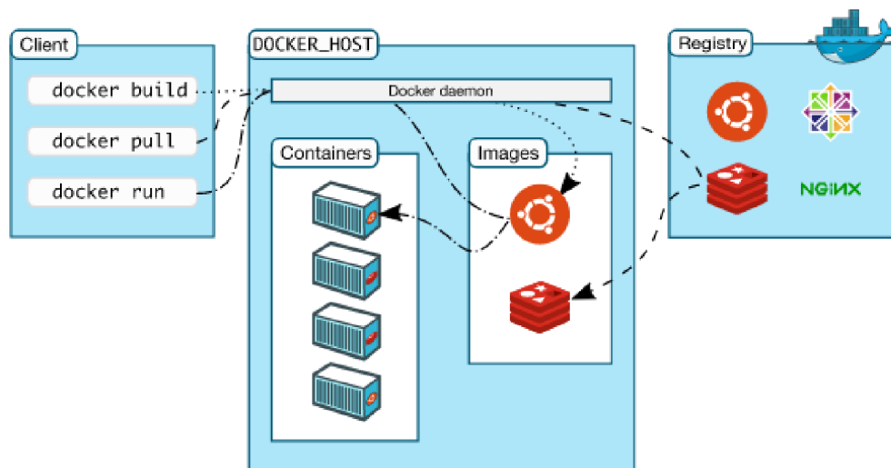
Obrázek 2.1: Architektura Dockeru
