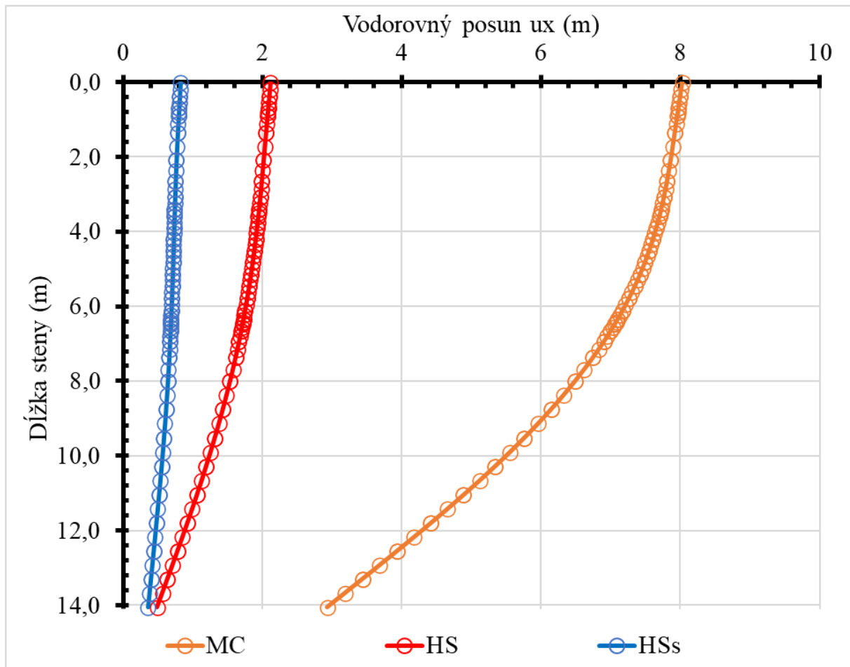
Obr. 25 Strop 1 – porovnanie vodoravných posunov
