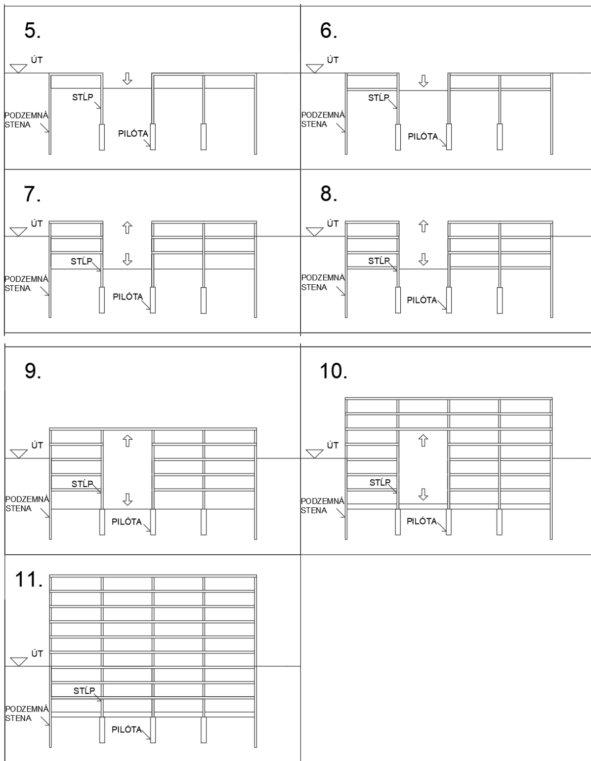
Obr. 1 Fázy výstavby- Metóda „Top down“
