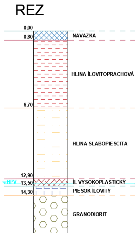
Obr. 5 Priečný rez v mieste paženia
