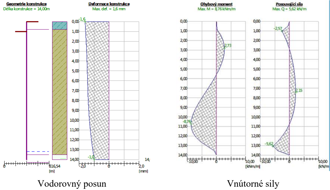
Obr. 7 Odkop 1
