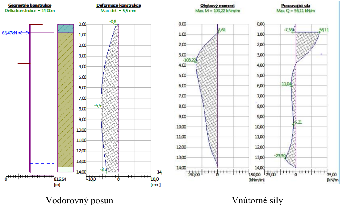
Obr. 8 Odkop 2
