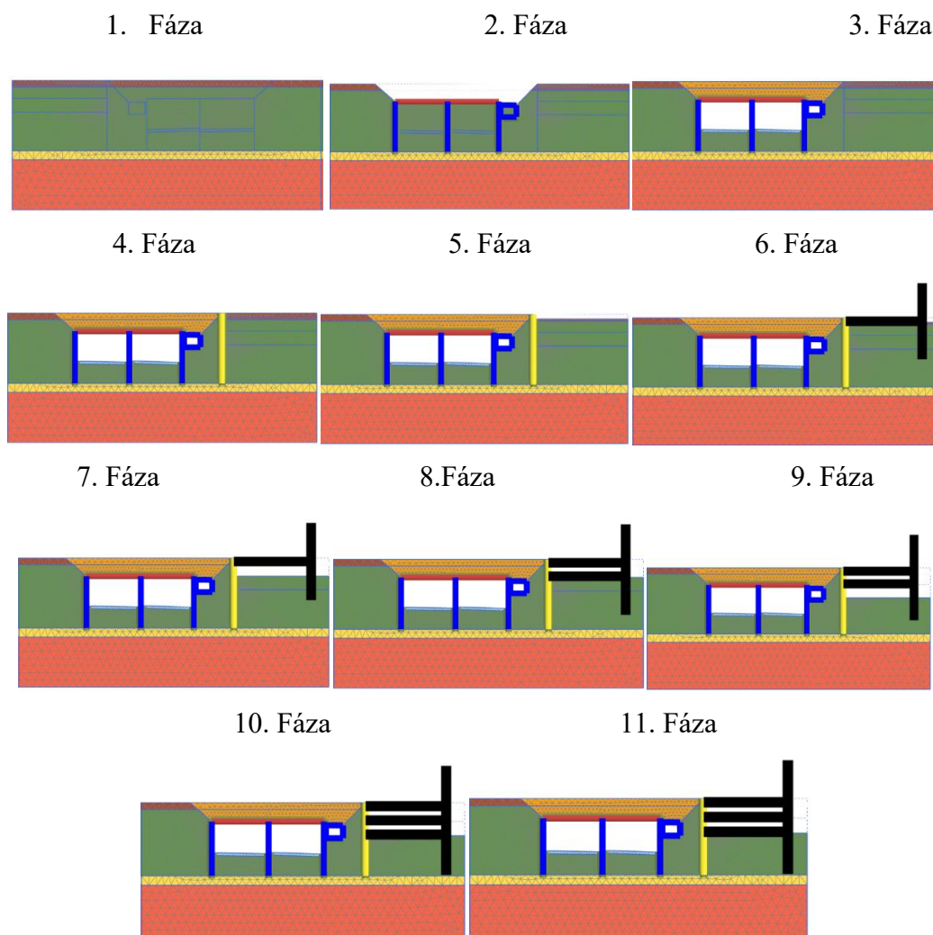
Obr. 14 Fázy výpočtu
