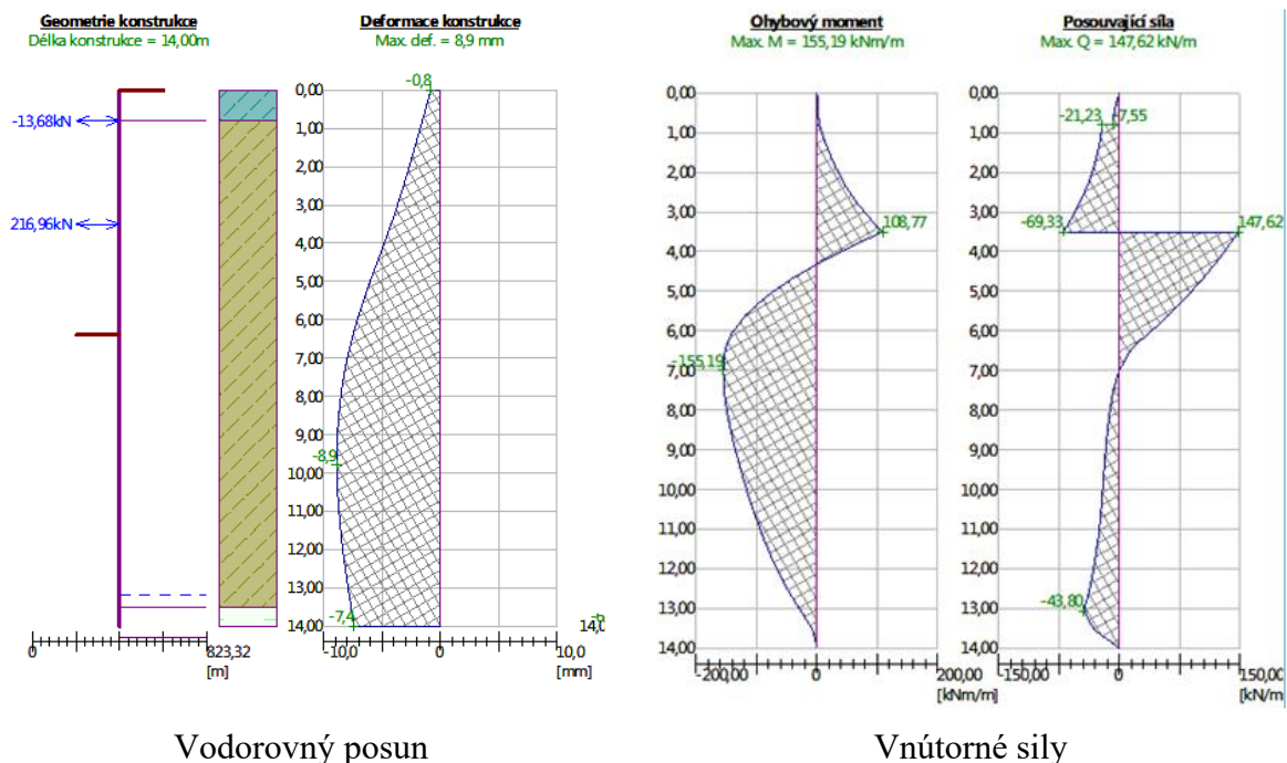
Obr. 9 Odkop 3
