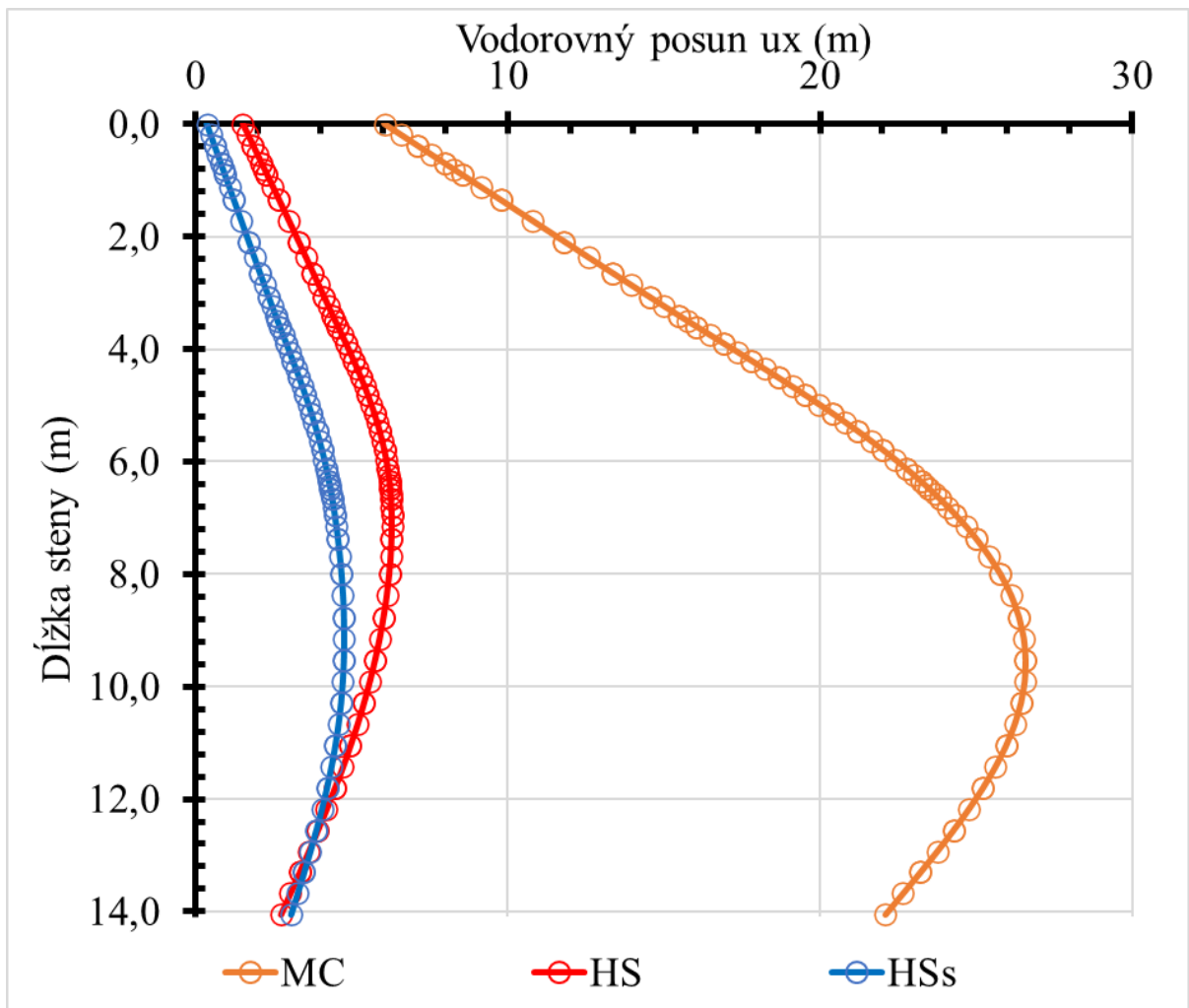
Obr. 27 Doska – porovnanie vodorovných posunov
