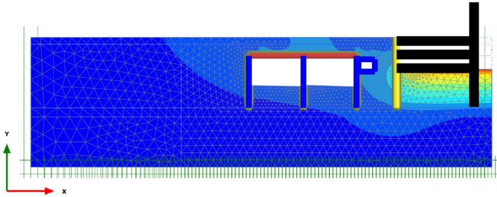
Obr. 18 Fáza 10 – Doska - Izplochy celkových posunov v okolí konštrukcie pre MC model
