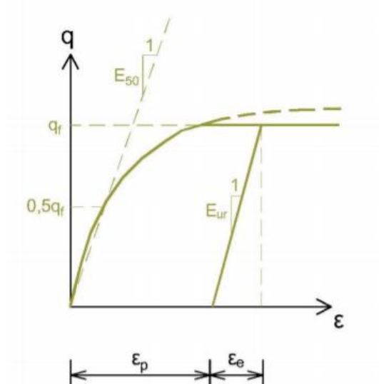
Obr. 12 Pracovný diagram HS modelu (10)
