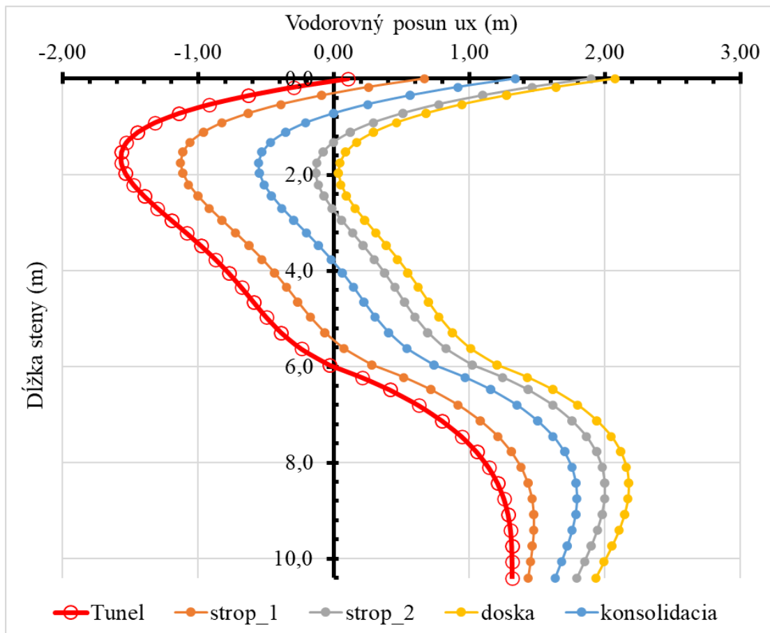
Obr. 37 Vodorovný posun – Favá stena
