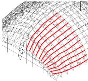
Obrázok 12: Väznice
