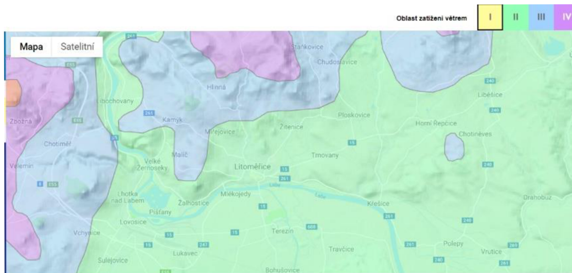
Obrázok 10: veterná mapa
