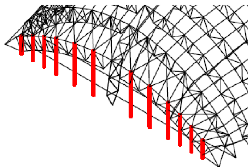
Obrázok 9: Stĺpy
