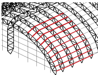
Obrázok 17: Väznice
