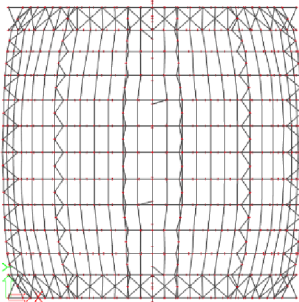
Obrázok 4: A Pôdorys
