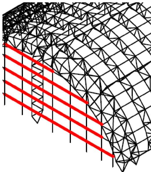
Obrázok 19: Paždíky
