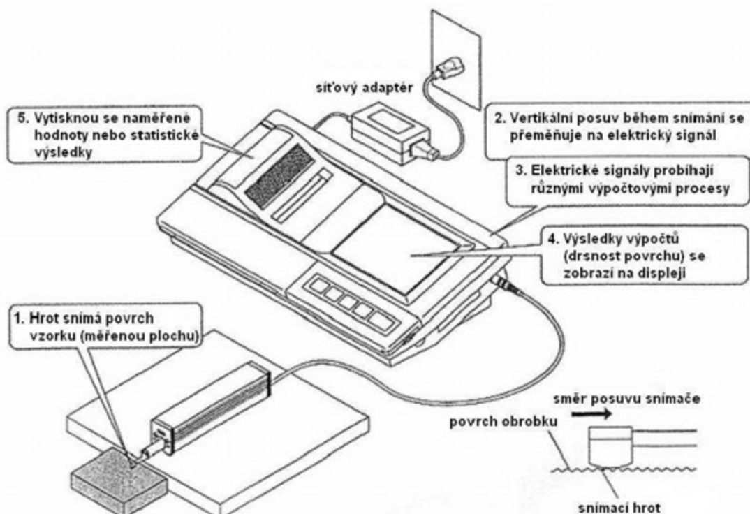
Obr. 4.3. Schéma přístroje Mitutoyo SJ-301
