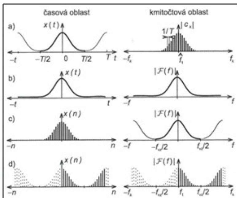
Obr. 2.11. Vztahy mezi časovou a kmitočtovou oblastí
