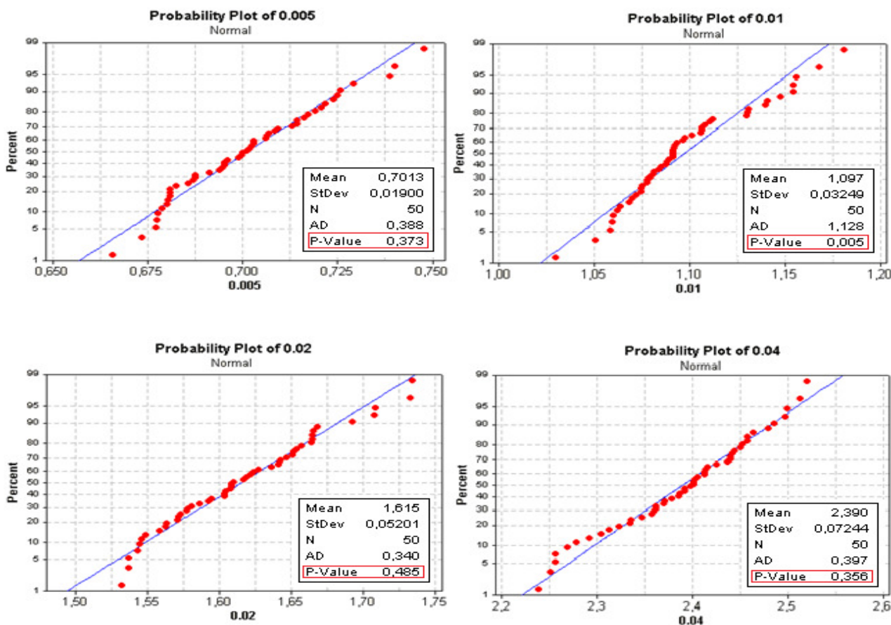
Obr. 6.2. Testy normality pro určení vlivu hloubky úběru na průměrnou aritmetickou úchytku posuzovaného profilu funkční plochy
