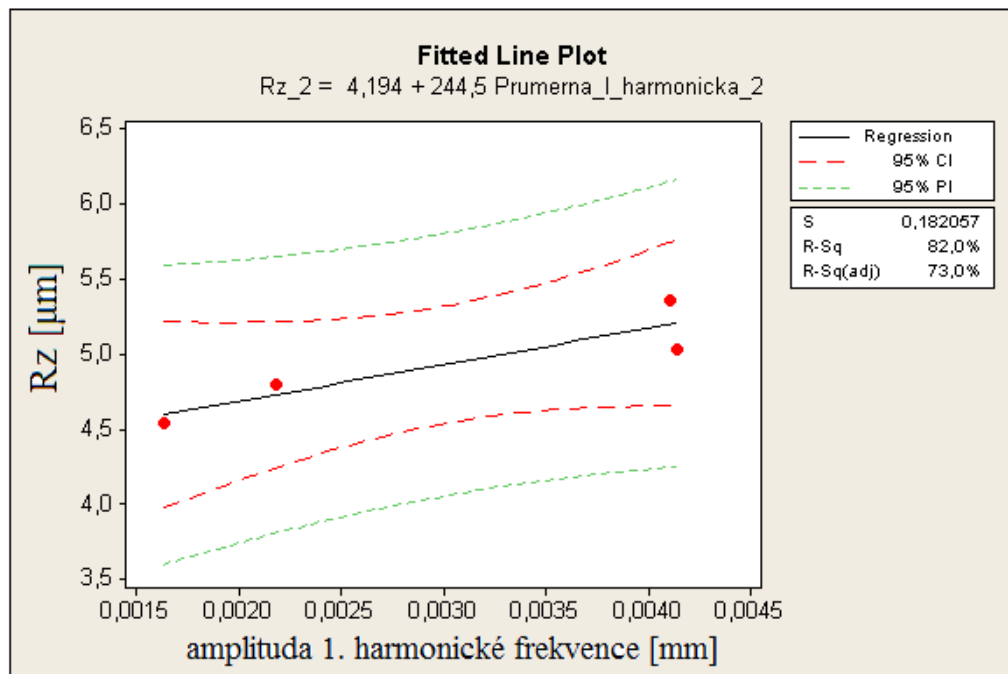
Obr. 7.10. Závislost parametru úchylky posuzovaného profilu Rz na amplitudě 1. harmonické frekvence při konstantní a_p a proměnné v_f v 2. roce
