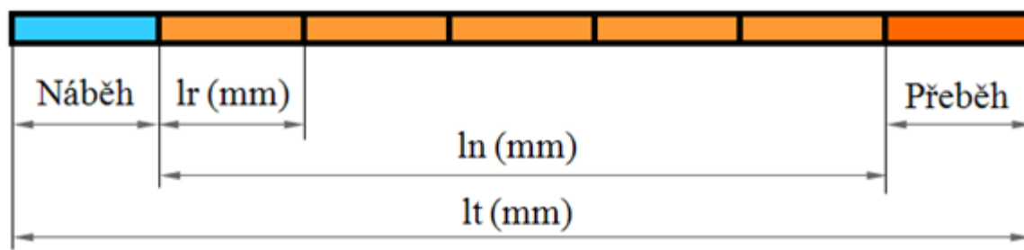
Obr. 3.2. Měřicí dráha snímače
