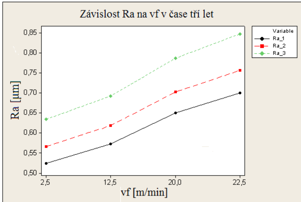
Obr. 7.15. Závislost průměrné aritmetické úchylky posuzovaného profilu Ra na posuvové rychlosti v době tří let
