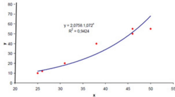
Obr. 2.19. Exponenciální regrese
