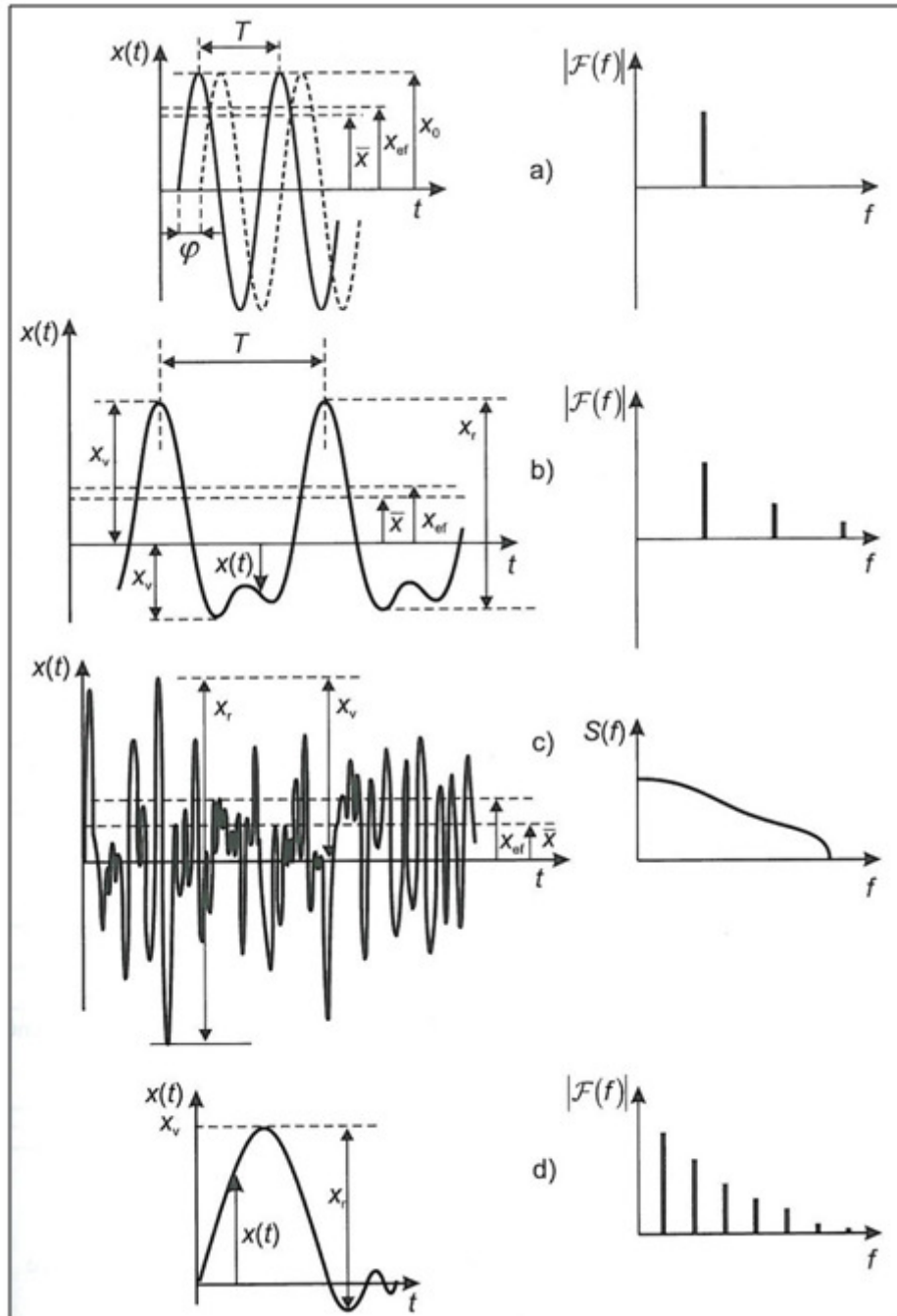
Obr. 2.6. Časové průběhy vibrací a odpovídající spektrální veličiny
