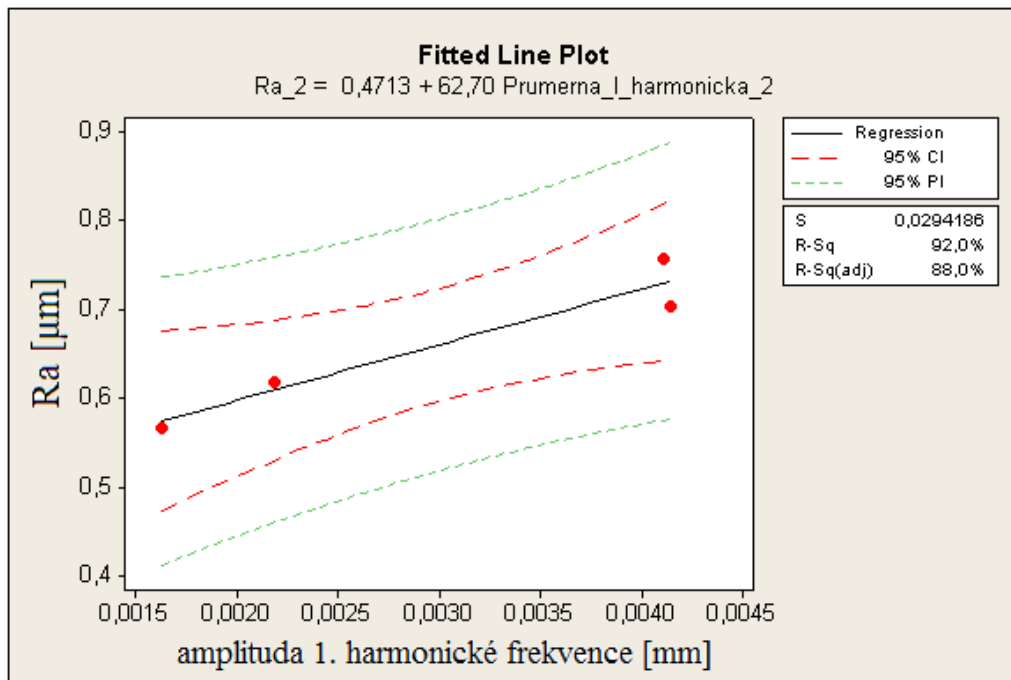
Obr. 7.9. Závislost průměrné aritmetické úchylky posuzovaného profilu Ra na amplitudě 1. harmonické frekvence při konstantní a_p a proměnné v_f v 2. roce
