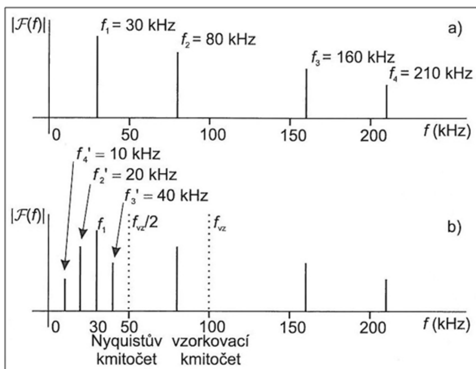
Obr. 2.9. Projev aliasingu
