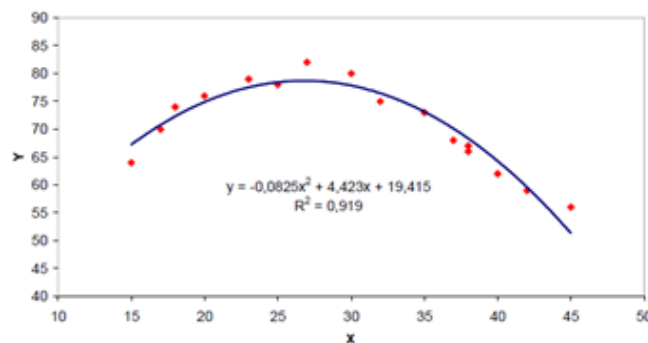
Obr. 2.17. Kvadratická regrese
