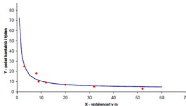
Obr. 2.18. Hyperbolická regrese
