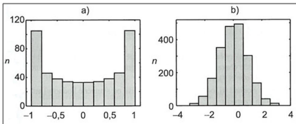
Obr. 2.10. Histogram
