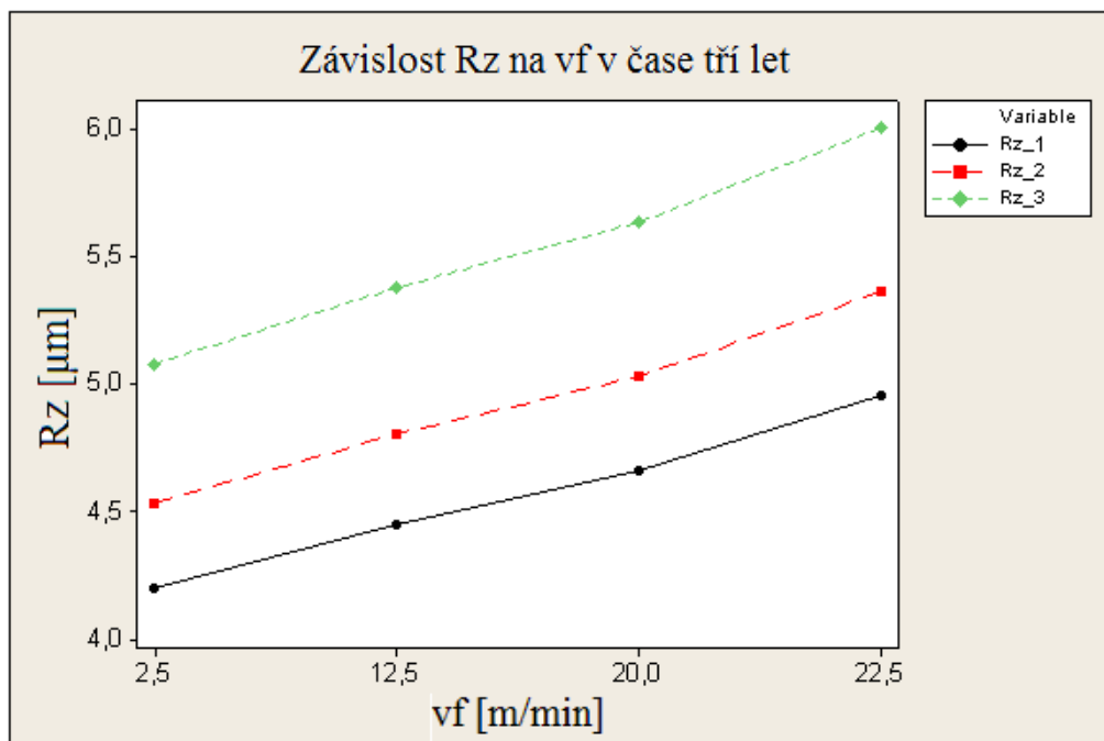
Obr. 7.16. Závislost parametru úchylky posuzovaného profilu Rz na posuvové rychlosti v době tří let
