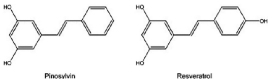
Obr.6 – Chemická struktura dvou zástupců stilbenů (Bioprospect, 2015)
