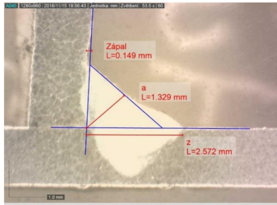
Obr. 33 Makrostruktura svaru [1]
