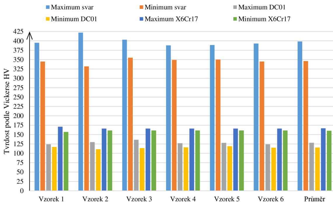
Obr. 70 Porovnání hodnot HV v různých oblastech vzorků
