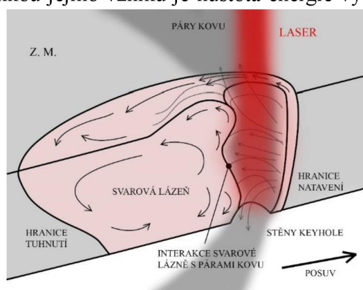
Obr. 7 Metalurgické procesy v key hole [20]
