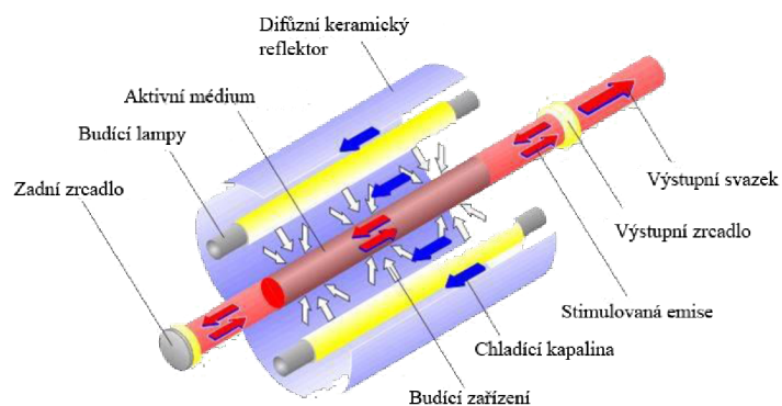
Obr. 16 Konstrukce laserového zdroje [34]
