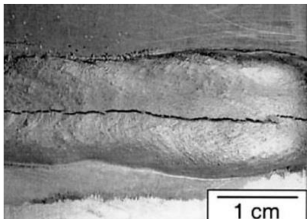
Obr. 28 Podélná trhlina [51]
