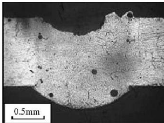
Obr. 27 Pomezita svaru [50]
