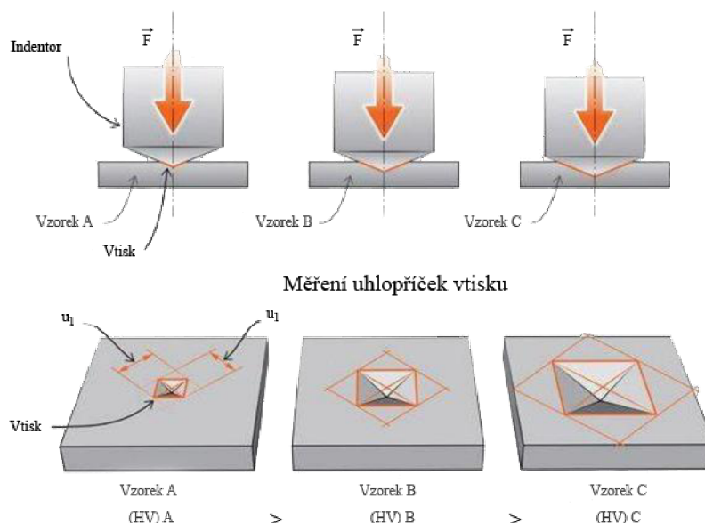
Obr. 35 Průběh zkoušky tvrdosti dle Vickerse [78]
