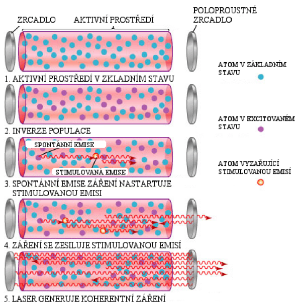
Obr. 10 Proces buzení atomů v rezonátoru [26]
