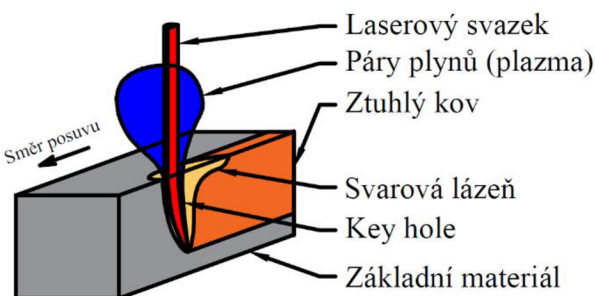
Obr. 6 Penetrační režim svařování [18]
