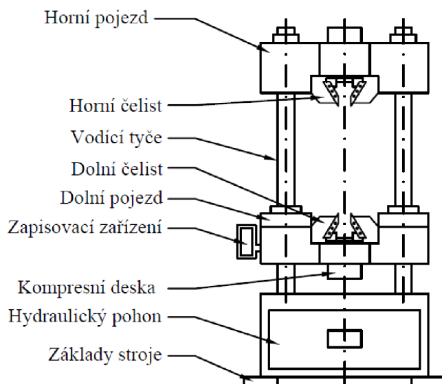
Obr. 30 Trhačický lis [70]
