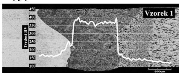
Obr. 71 Průběh tvrdosti na vzorku 1
