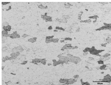
Obr. 40 Výchozí struktura DC01
