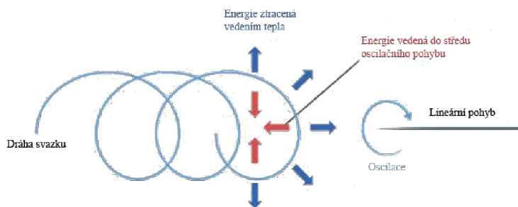
Obr. 21 Schéma pohybových vektorů při rozmítání svazku [43]
