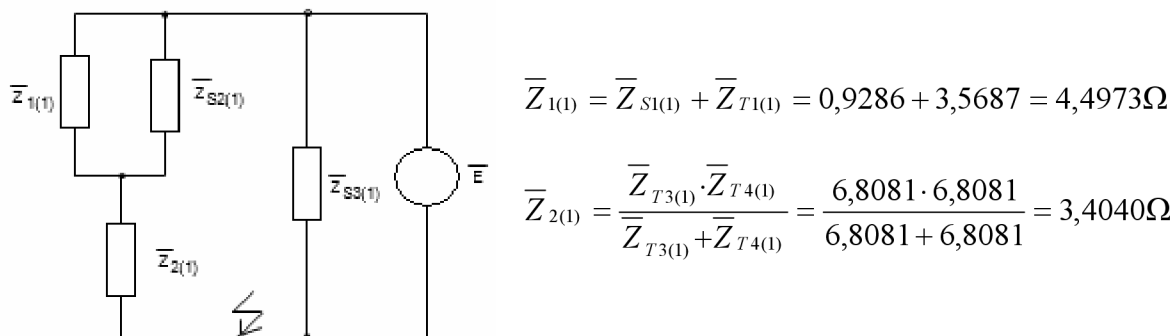
Obrázek 13: Zjednodušování obvodu 1
