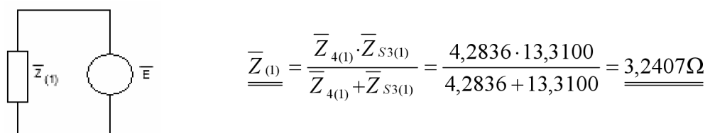
Obrázek 75: Výsledná sousledná 3f zkratová impedance po zavedení přímé transformace
