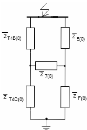
Obrázek 26: Zjednodušení obvodu 7
