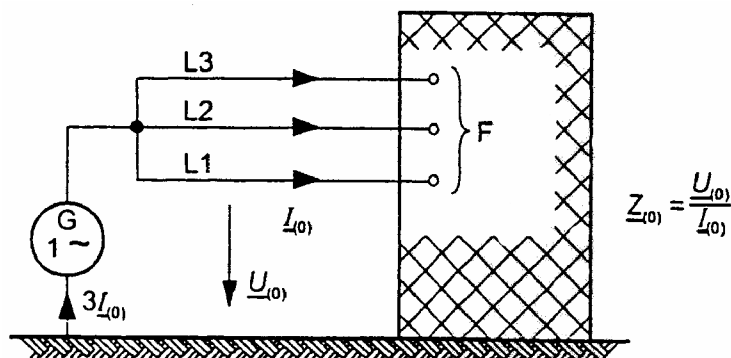
Obrázek 6: Netočivá složka zkratové impedance \underline{Z}_{(0)} v místě zkratu F
