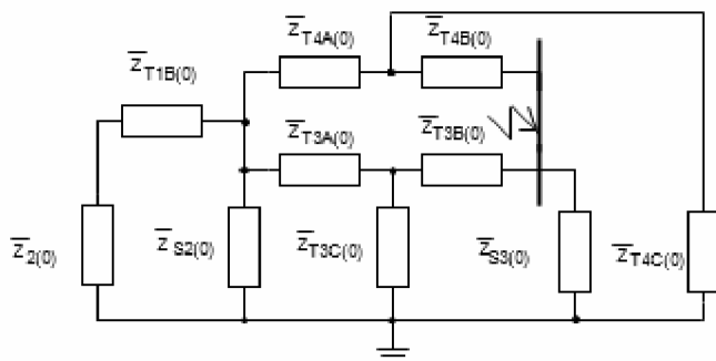
Obrázek 58: Zjednodušování obvodu 2
