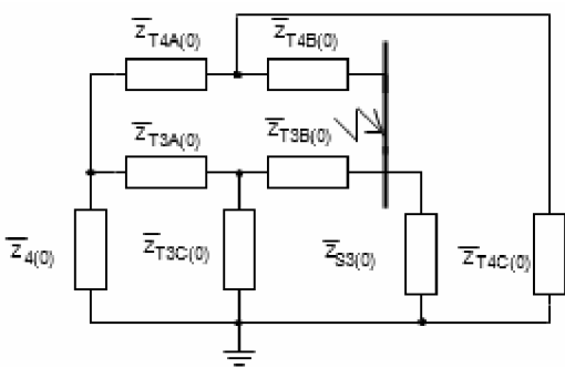
Obrázek 60: Zjednodušování obvodu 4
