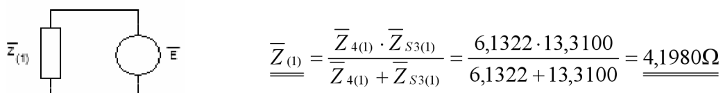
Obrázek 54: Výsledná sousledná 3f impedance před zavedením přímé transformace
