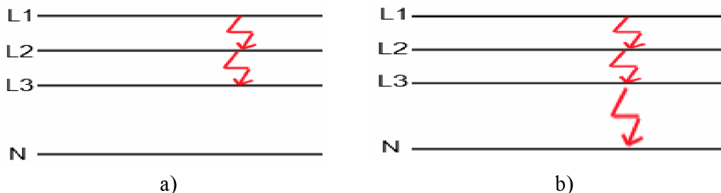
Obrázek 1: Druhy souměrných zkratů [2]
