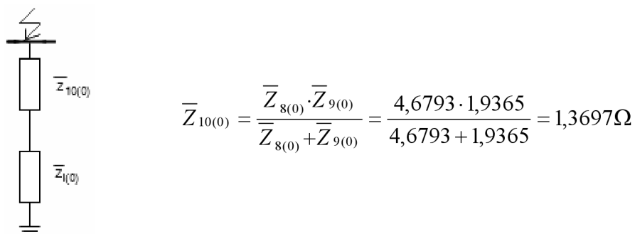
Obrázek 67: Zjednodušení obvodu 10
