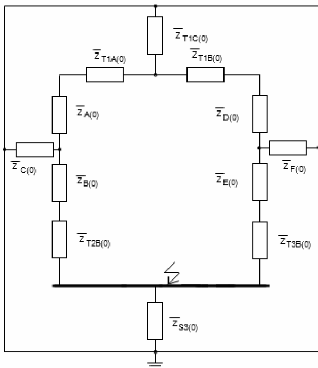
Obrázek 78: Zjednodušení obvodu 1 –
