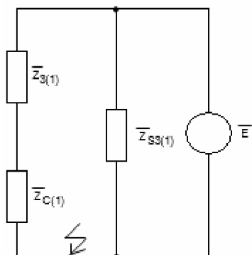
Obrázek 35: Zjednodušování obvodu 3
