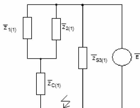
Obrázek 34: Zjednodušování obvodu 2
