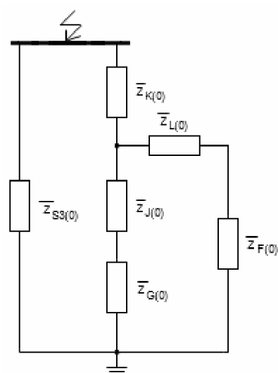
Obrázek 44: Zjednodušování obvodu 5 - Transfigurace \bar{Z}_{4(0)} , \bar{Z}_{5(0)} , \bar{Z}_{6(0)}
