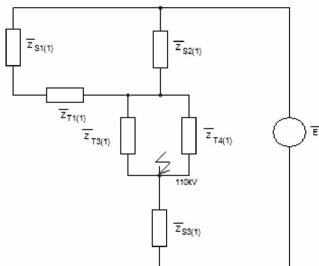
Obrázek 50: Překreslené schéma sousledné složky
