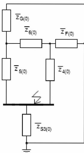
Obrázek 81: Zjednodušení obvodu 4
