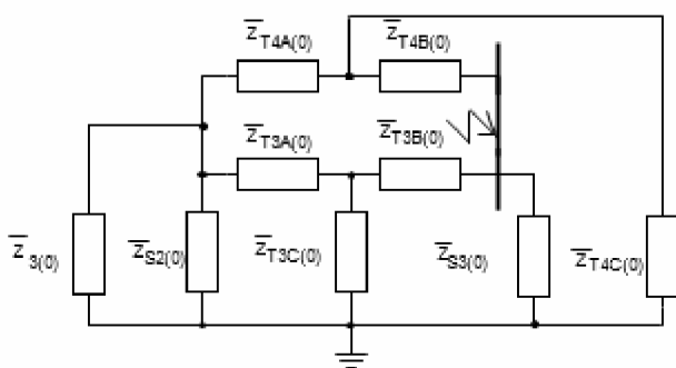
Obrázek 59: Zjednodušování obvodu 3
