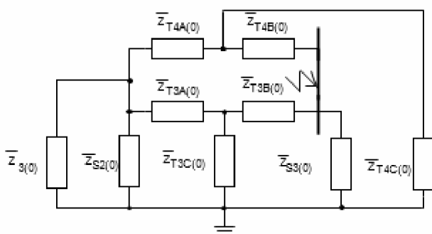
Obrázek 21: Zjednodušení obvodu 3
