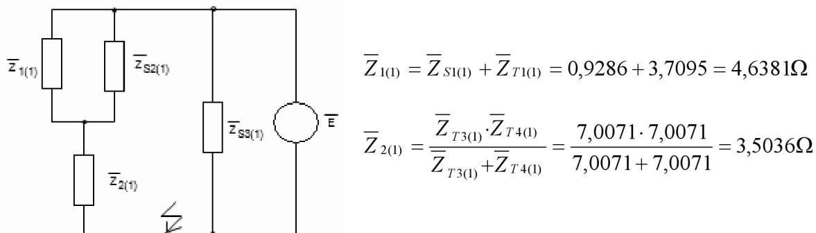
Obrázek 51: Zjednodušování obvodu 1
