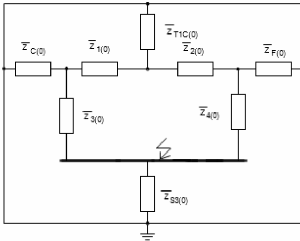
Obrázek 79: Zjednodušení obvodu 2
