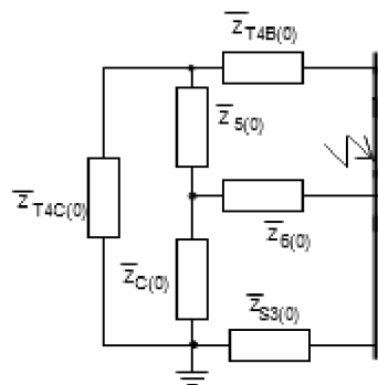
Obrázek 24: Zjednodušování obvodu 5
