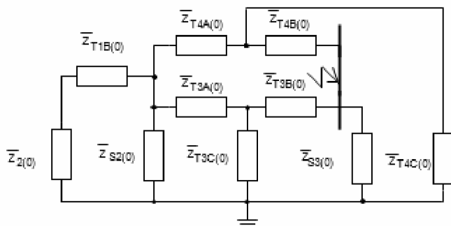
Obrázek 20: Zjednodušení obvodu 2
