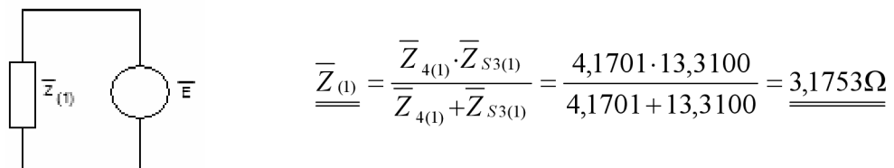
Obrázek 37: Výsledná sousledná 3f zkratová impedance po zavedení přímé transformace
