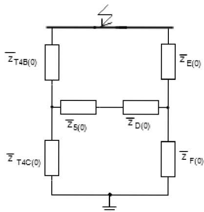
Obrázek 25: Zjednodušení obvodu 6 – Transfigurace \bar{Z}_{6(0)} , \bar{Z}_{C(0)} , \bar{Z}_{S3(0)}
