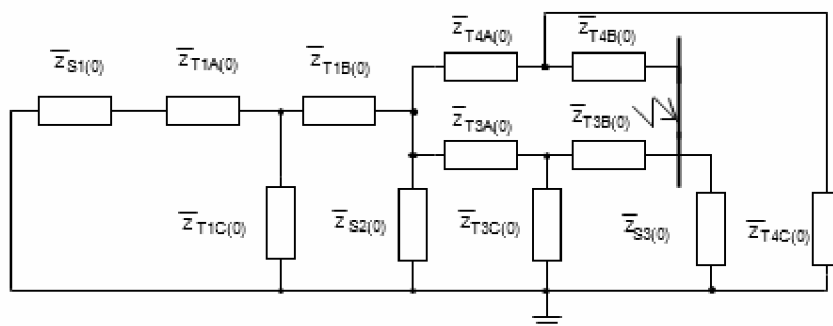
Obrázek 56: Překreslené schéma netočivé složky
