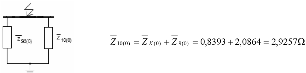
Obrázek 46: Zjednodušení obvodu 7
