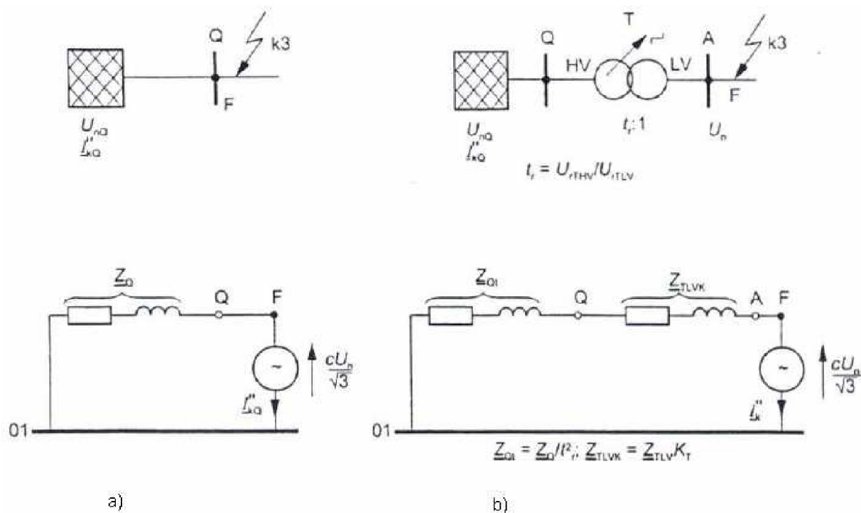
Obrázek 7: Schéma soustavy a ekvivalentní náhradní schéma síťových napáječů a) Bez transformátoru b) S transformátorem
