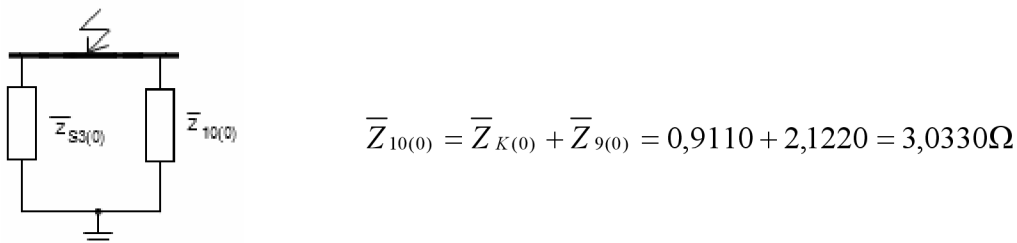
Obrázek 84: Zjednodušení obvodu 7
