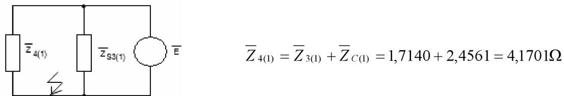
Obrázek 36: Zjednodušení obvodu 4
