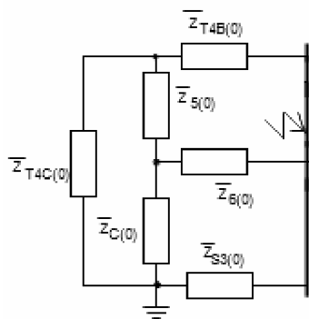
Obrázek 62: Zjednodušování obvodu 5
