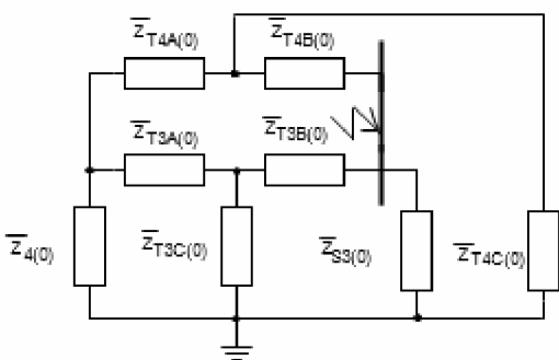
Obrázek 22: Zjednodušení obvodu 4
