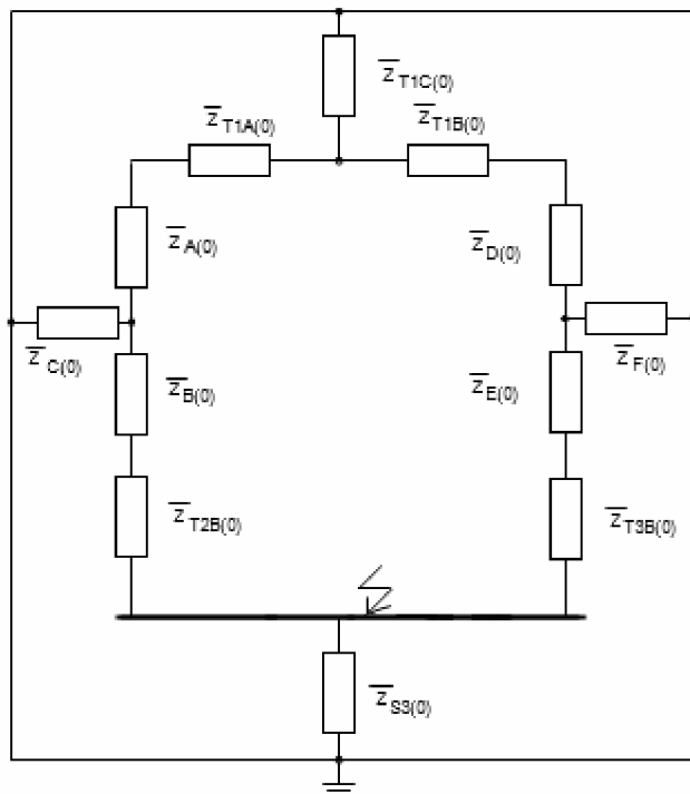
Obrázek 40: Zjednodušení obvodu 1 –
