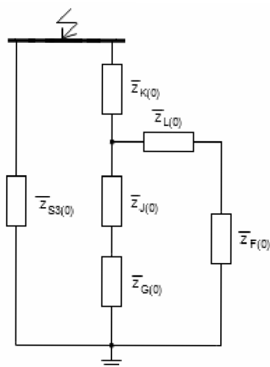
Obrázek 82: Zjednodušení obvodu 5 - Transfigurace \bar{Z}_{4(0)} , \bar{Z}_{5(0)} , \bar{Z}_{6(0)}
