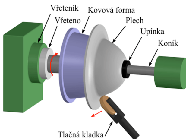
Obr. 6 Schéma kovotlačení [19]
