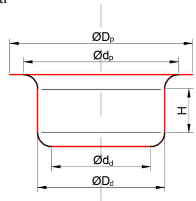
Obr. 32 Označení průměrů
