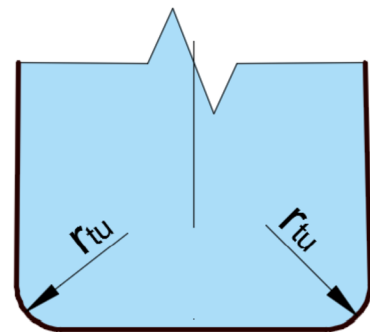
Obr. 38 Zaoblení tažníku
