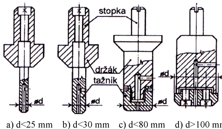
Obr. 20 Provedení tažníků [9]
