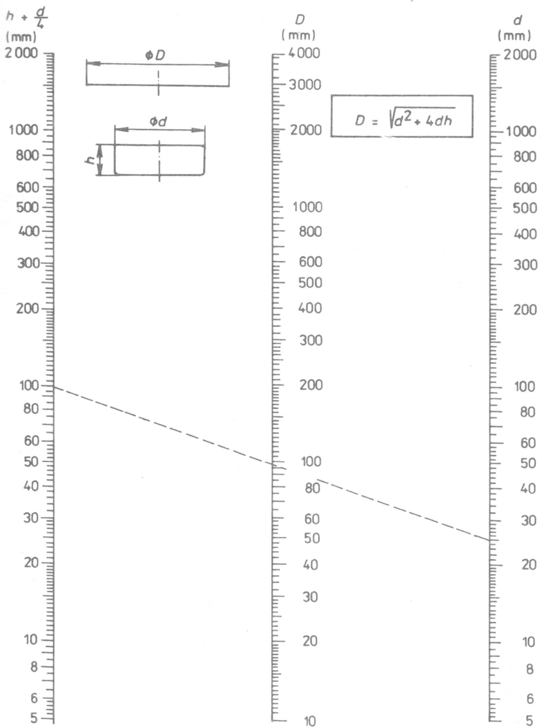
Obr. 5. Graf pro výpočet průměru přístřihu
