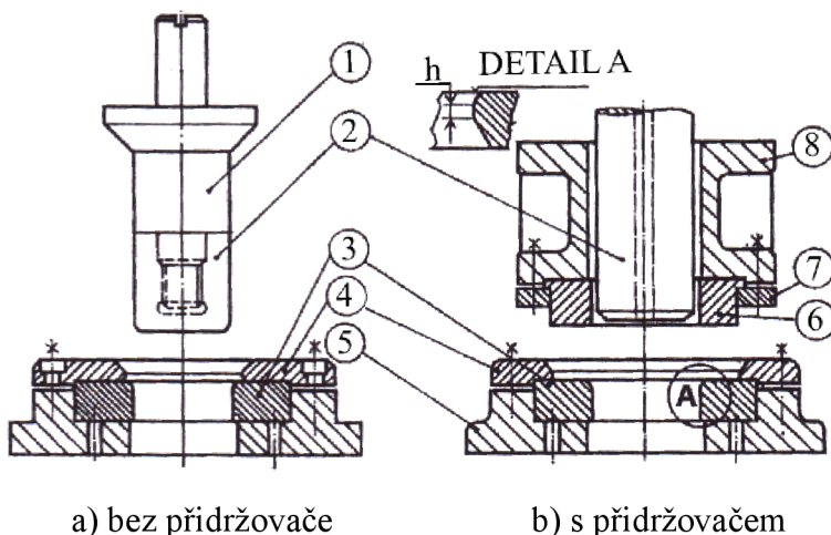
Obr. 18 Tažidla [9]
