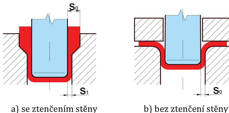
Obr. 5 Rozdělení tažení
