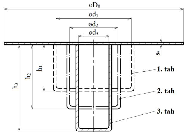
Obr. 15 Víceoperační tažení [5]
