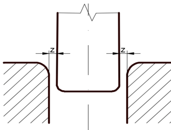
Obr. 36 Tažná mezera
