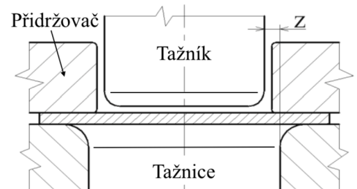
Obr. 16 Tažná mezera
