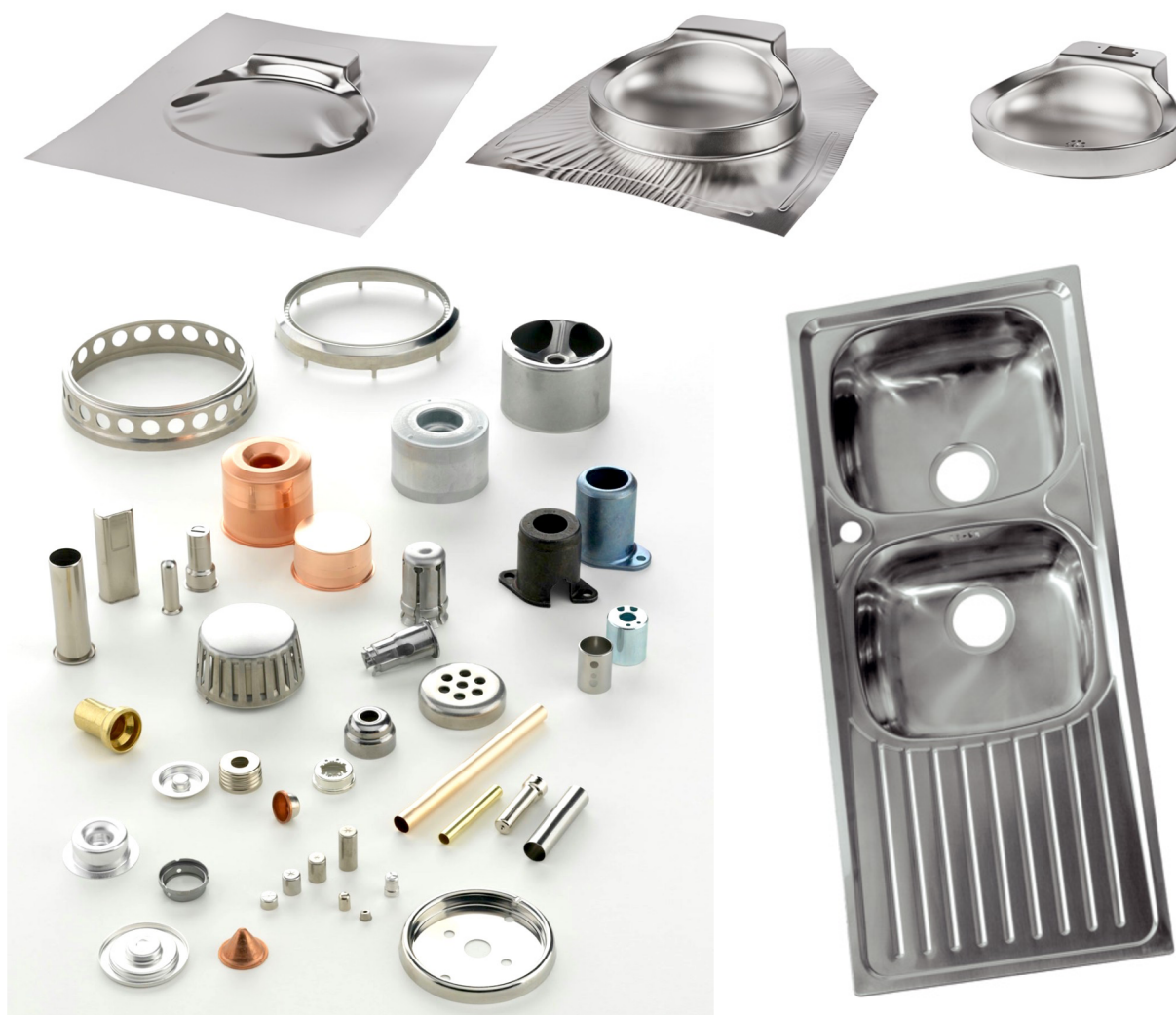
Obr. 1 Příklady součástí vyrobených tažením [4], [8], [7]
