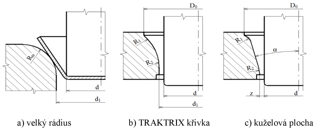
Obr. 21 Úpravy tažné hrany tažnic [6]
