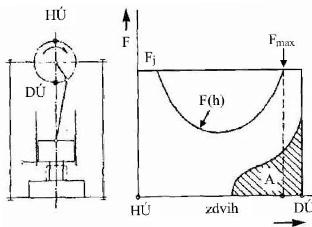
Obr. 26 Schéma klikového mechanismu [17]
