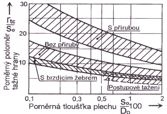
Obr. 23 Doporučené hodnoty r_0 [9]
