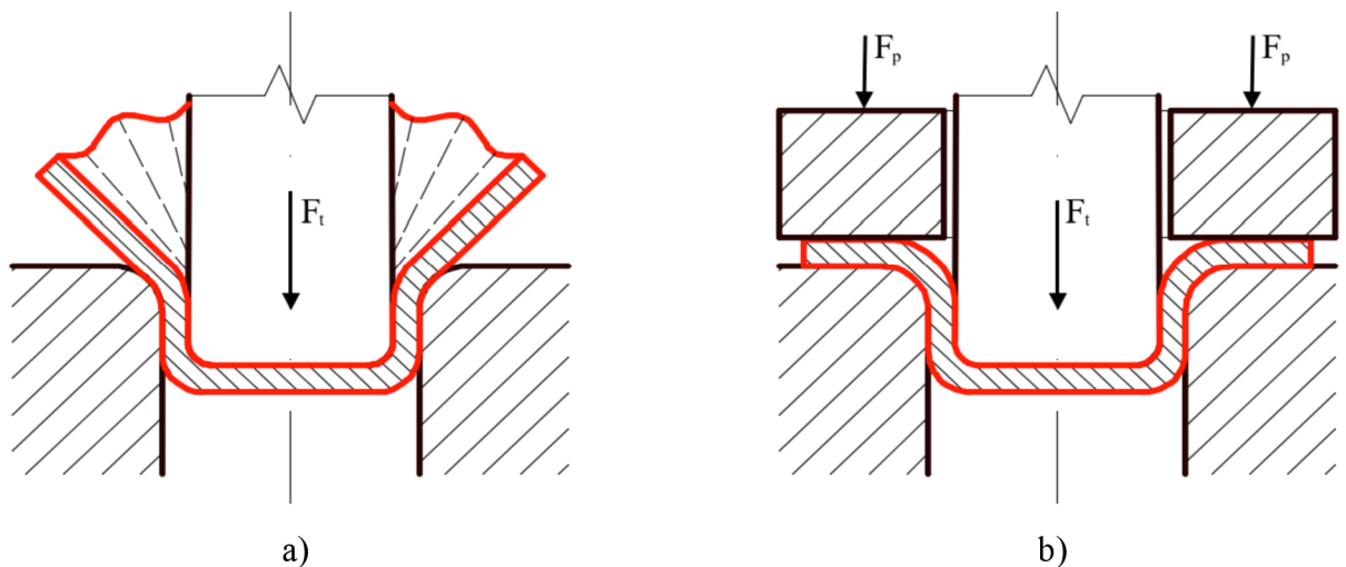
Obr. 24 Použití přídržovače
