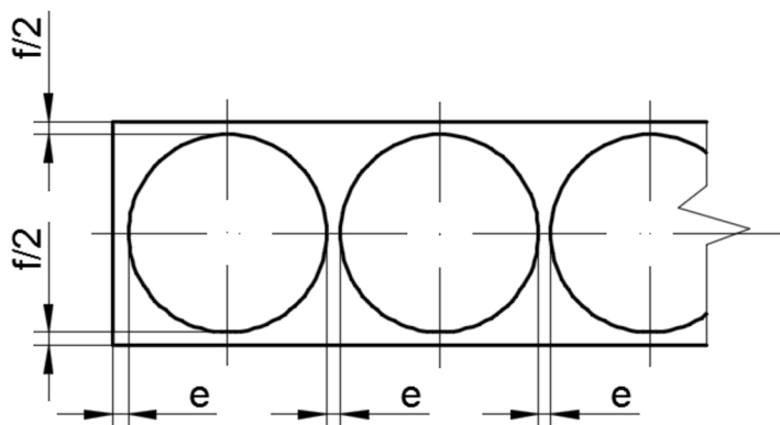
Obr. 33 Velikost můstku a přepážky
