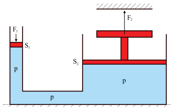
Obr. 27 Princip hydraulického lisy
