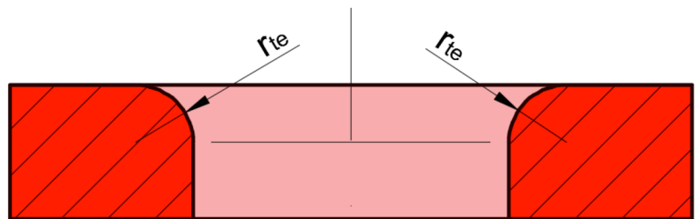
Obr. 37 Zaoblení tažnice
