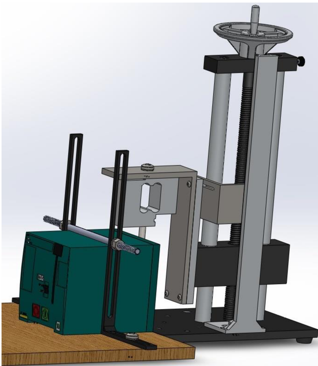
Obrázek 4-1: Měřicí pracoviště
