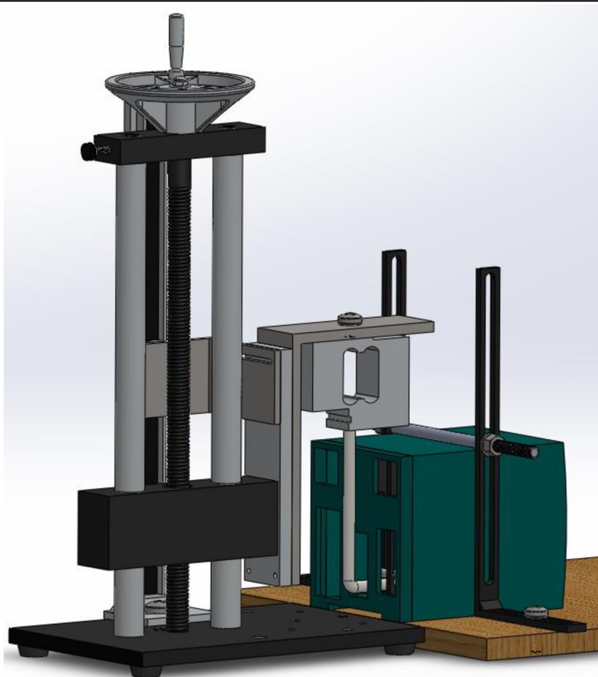
Obrázek 4-2: Měřicí pracoviště
