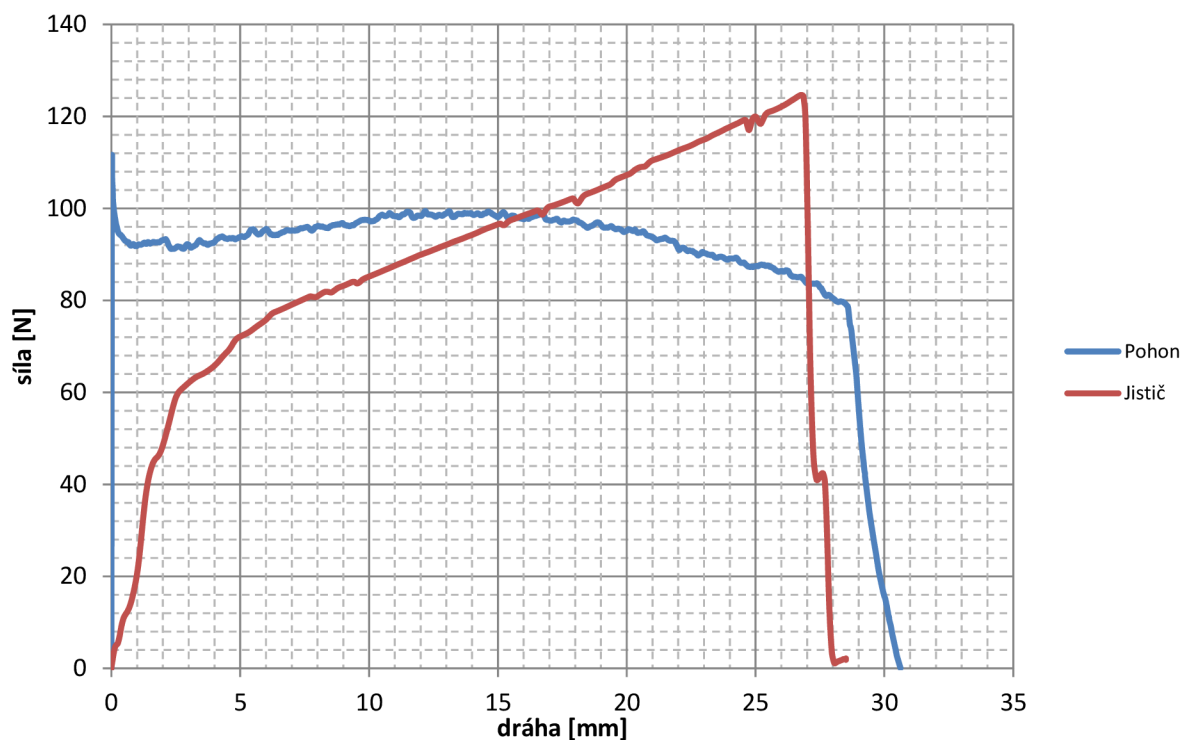
Obrázek 5-9: Porovnání sil pohonu a jističe pro stav Vypnuto – Zapnuto
