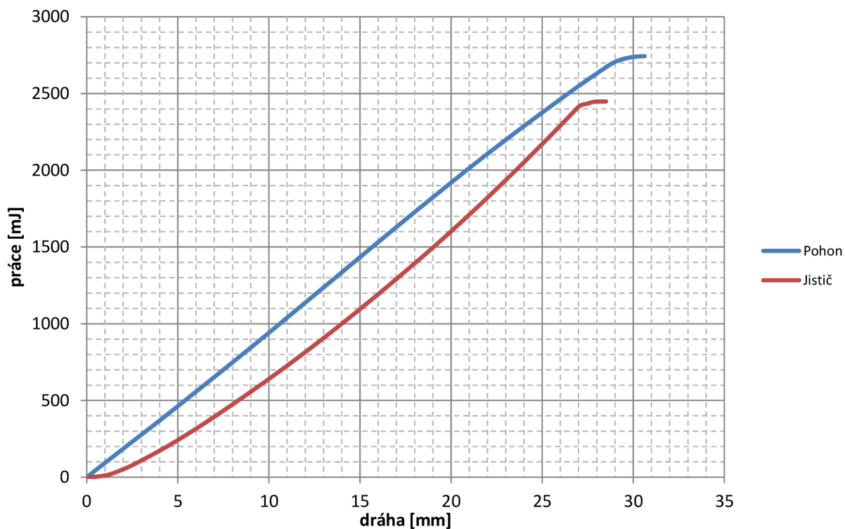
Obrázek 5-10: Porovnání práce pohonu a jističe pro stav Vypnuto – Zapnuto
