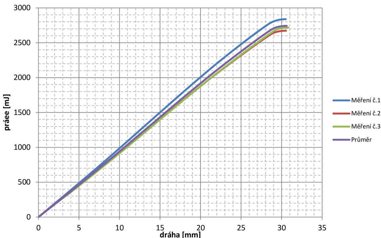
Obrázek 5-2: Průběh vykonané práce pohomu ze stavu Vypnuto – Zapnuto
