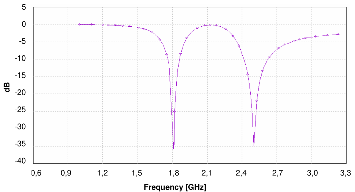
Obr. 5.3.1.2. Graf činitele odrazu S_{11} antény s umístěním SRR nejbliže ke středu
