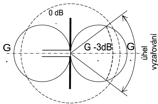
Obr. 2.3.3. Vyzařovací charakteristika půlvlnného dipólu
