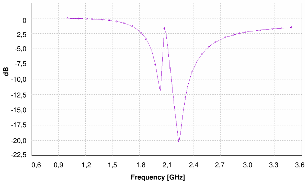
Obr. 5.2.2.4. Graf činitele odrazu S_{11} antény s nejbližšími frekvenčními pásmy vytvořenými pomocí dvojice SRR
