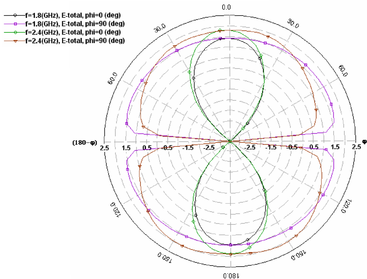
Obr. 6.2.3. Vyzářovací charakteristiky celé antény s balunem
