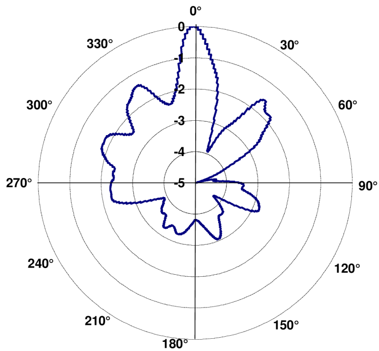
Obr. 7.3. Směrová charakteristika antény v rovině H pro f = 1,8 GHz
