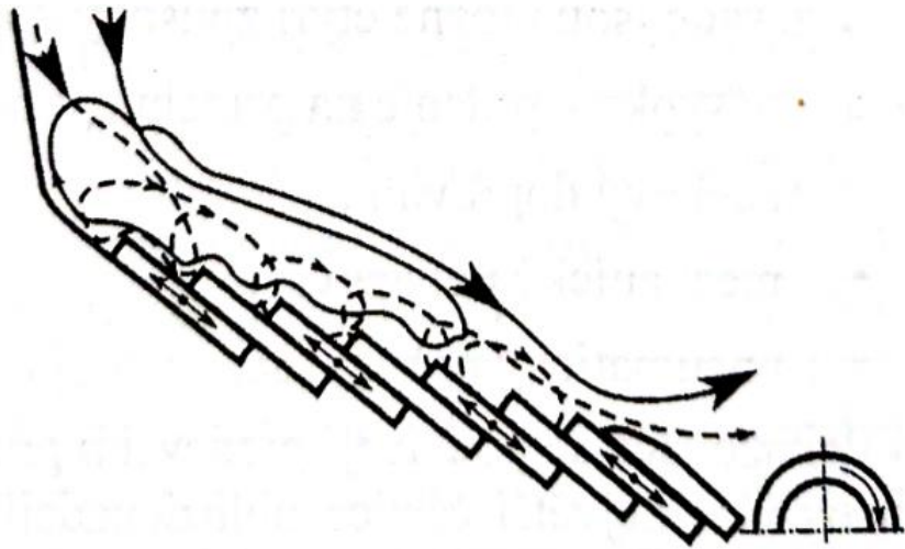
Obr.3: Vratisuvný rošt typu Martin. [20]
