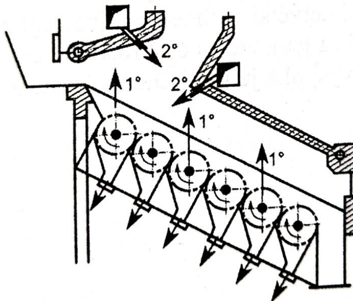
Obr.4: Válcový rošt. [20]
