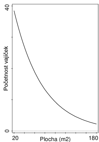
Obrázek 25. GLM závislosti početnosti vajíček \cdot sonda -1 na ploše tůně
