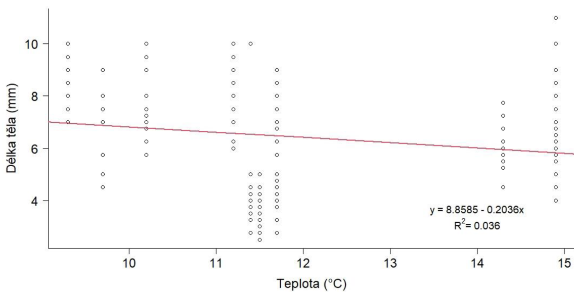
Příloha 8. Lineární regrese délky těla larev v období od 24.04.–15.05.2023, body jsou průměrné hodnoty ze všech lokalit.
