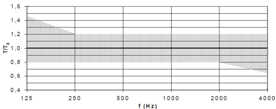
Obr. 2 : Přípustné rozmezí poměru dob dozvuku T/T_0 prostoru určeného především pro hudbu v závislosti na středním kmitočtu oktávového pásma. 2
