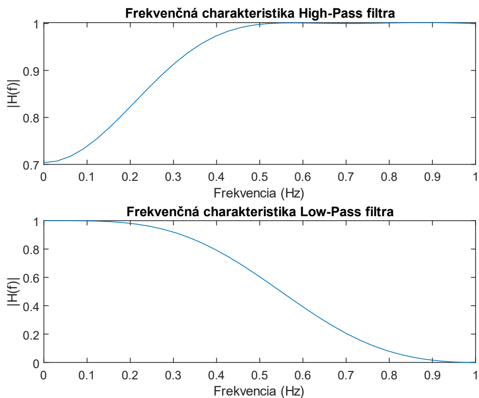
Obr. 2.3 Frekvenčná charakteristika využitých FIR filtrov
