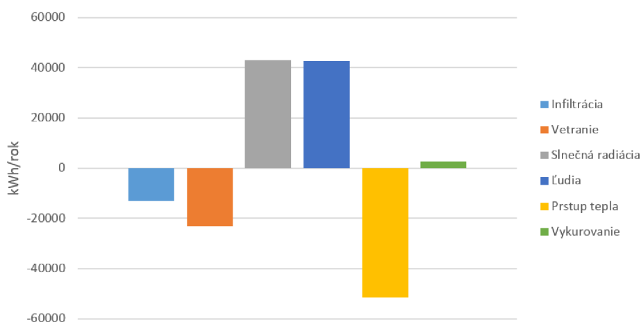
Obr. 4.16: Energetická bilancia pri uvažovaní teploty 13 °C a vplyvu osôb
