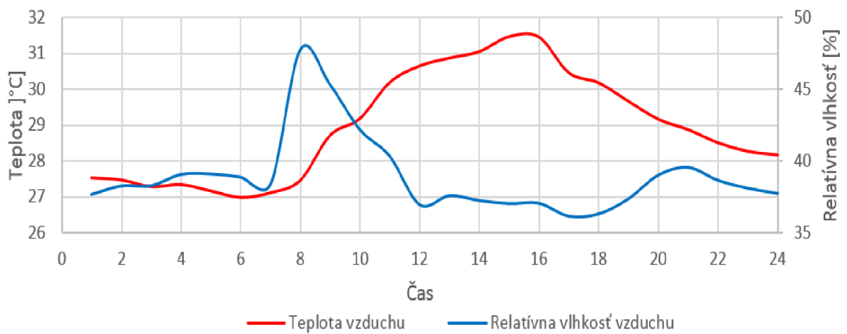
Obr. 4.11: Priebeh vnútornej teploty a relatívnej vlhkosti v letnom období pri uvažovaní vplyvu osôb
