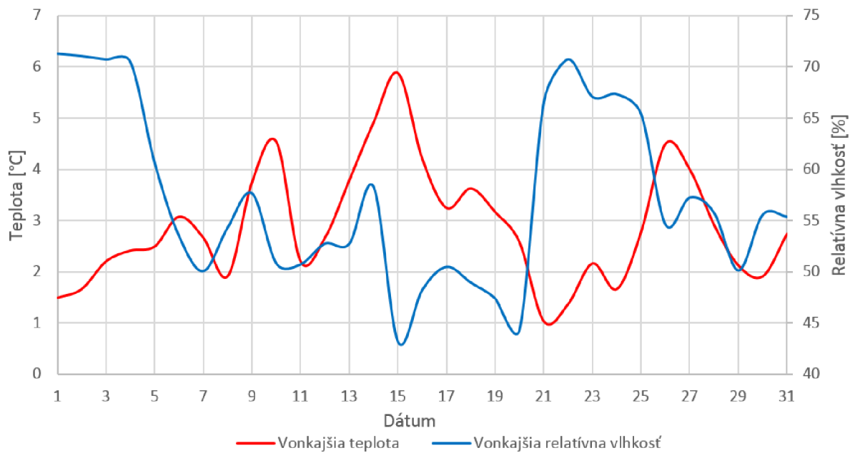
Obr. 4.3: Simulácia priebehu vonkajšej teploty a relatívnej vlhkosti, január
