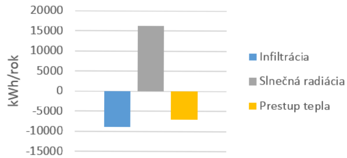
Obr. 4.22: Energetická bilancia internátu, súčasný stav
