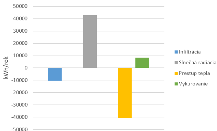
Obr. 4.15: Energetická bilancia pri uvažovaní teploty 13 °C bez vplyvu osôb
