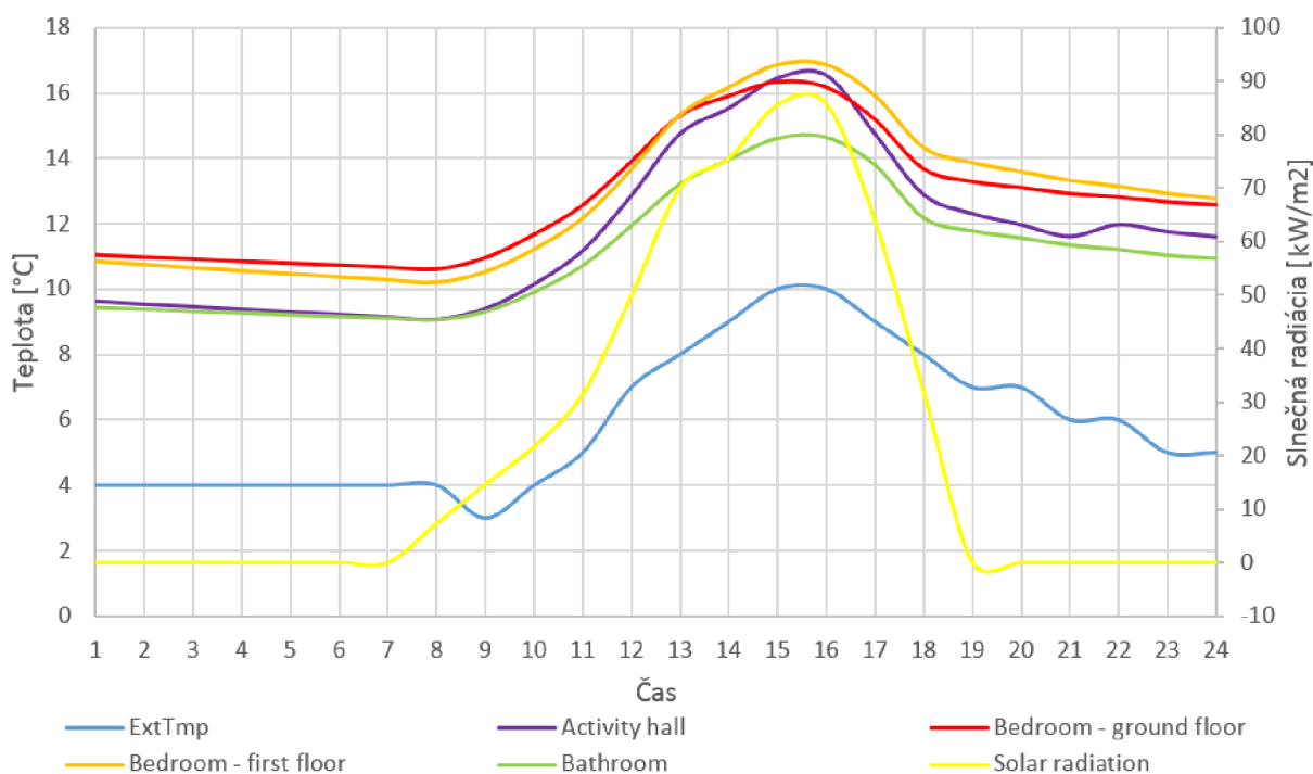
Obr. 4.17: Priebeh teplôt v internátu v chladnom dni
