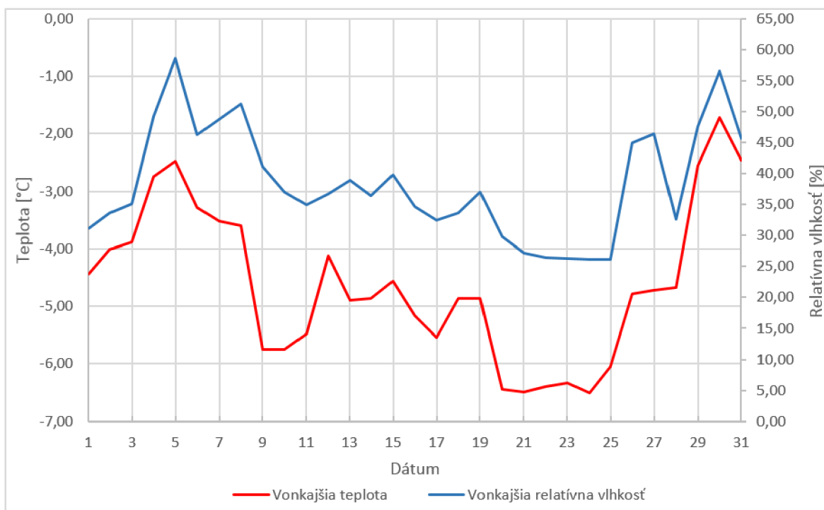
Obr. 3.3: Priemerné vonkajšie denné teploty a relatívne vlhkosti v januári 2016
