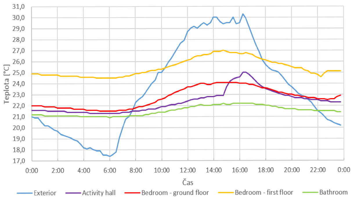
Obr. 3.15: Priebeh teplôt vzduchu v internátu, 2.7.2016
