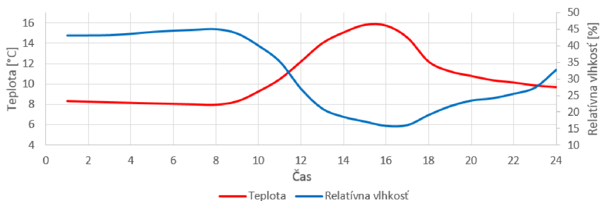
Obr. 4.8: Priebeh vnútornej teploty a relatívnej vlhkosti, zimné obdobie
