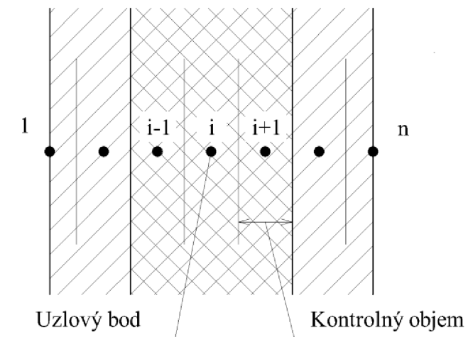
Obr. 2.11: Rozloženie konštrukcie na kontrolné objemy a poloha uzlových bodov
