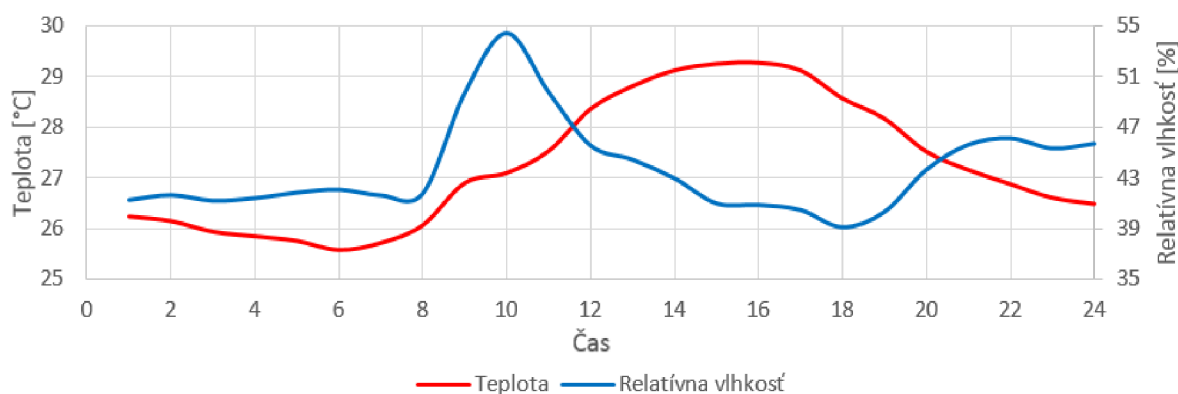
Obr. 4.9: Priebeh vnútornej teploty a relatívnej vlhkosti, letné obdobie
