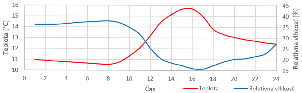
Obr. 4.23: Priebeh vnútornej teploty a relatívnej vlhkosti v miestnosti, zimné obdobie
