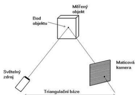
Obrázek 18: Triangulační trojúhelník 144
