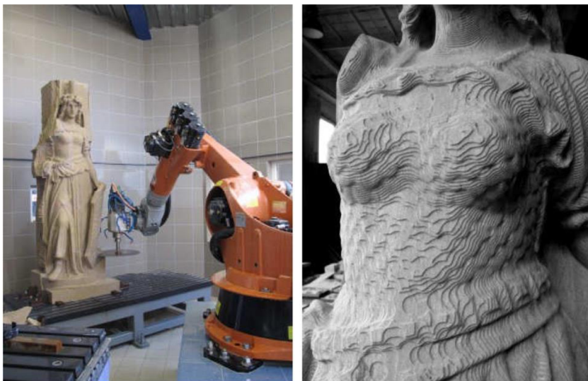
Obrázek 3: Robotické obrábění repliky Austrie 77
