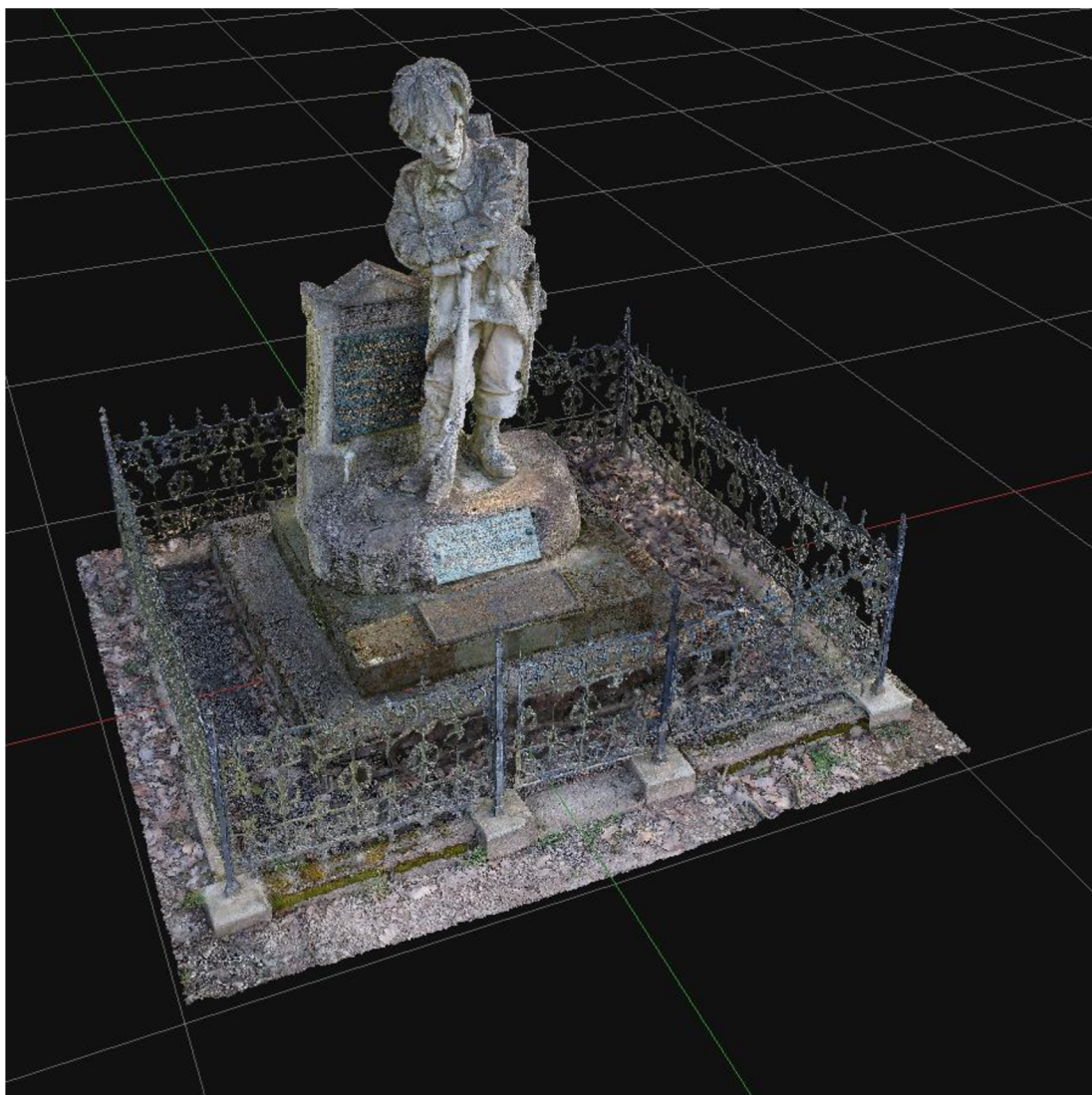
Obrázek 31: Náhled vytvořeného modelu pomníku číslo 292
