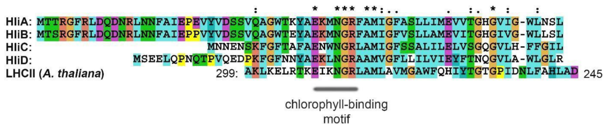
Obr. 5 Porovnání proteinových sekvencí Hlips z modelové sinice Synechocystis (HliA-D) spolu se sekvencí třetího transmembránového genu LHCII. Chl-vazný motiv (ExxNGR), konzervovaný v celé rodině LHC (like) proteinů je zvýrazněn (Konert et al., 2022).
