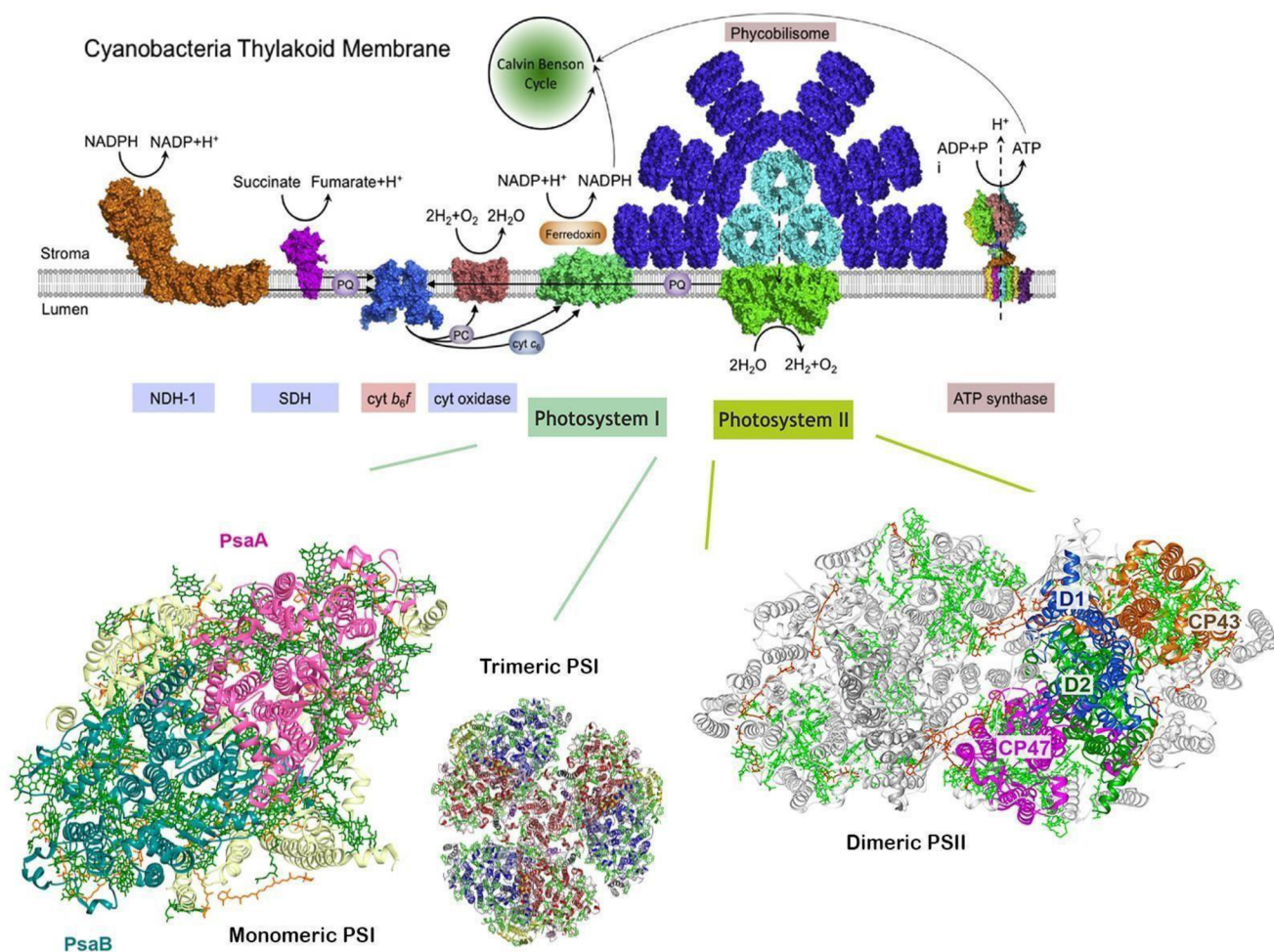
Obr. 1 Struktury proteinových komplexů účastníci se oxygenní fotosyntézy a respirace na tylakoidní membráně sinic. PSII spolu s NADPH dehydrogenázou (NDH-1) a sukcinát dehydrogenázou (SDH) redukuje plastochinon, který je poté oxidován cytochromem b 6 f (cyt b 6 f) za tvorby protonového gradientu. Elektrony jsou poté buď přeneseny na cytochrom c, nebo na plastocyanin. Cytochrom c je oxidován cytochrom c oxidázou (cyt oxidase), která se podílí na tvorbě protonového gradientu. Plastocyanin je oxidován PSI a dochází k redukci ferredoxinu. PSI můžeme najít buď ve formě monomeru obsahující jednotku PsaA a PsaB nebo ve formě trimeru (Jordan et al., 2001), který celkem obsahuje 6 podjednotek PsaA/PsaB. PSII existuje ve formě dimeru a hlavní podjednotky PSII jsou D1, D2, CP47, CP43. Na stromální straně je na PSII navázán gigantický komplex fykobilizom, který slouží jako externí světlosběrná anténa. Na lumenální straně se na PSII připojuje – kyslík tvořící komplex (OEC). Poslední enzym účastníci se světelné fáze fotosyntézy je ATP syntáza, která syntetizuje ATP za spotřeby protonového gradientu (Xu et al., 2004).
