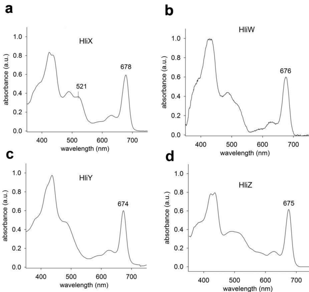
Obr. 11 Absorbanční spektra separovaných Hliů v CN gelu a) Z SDS-PAGE gelu byl vyříznut kousek gelu obsahující His-HliX-HliC dimer (viz Obr. 8b) a vložen do spektrofotometru. Spektrofotometr zaznamenal absorbanci světla od 350 nm – 750 nm, b-d) Měření spekter His-HliC, His-HliY a His-HliZ bylo provedeno identicky. Wavelength (nm) – vlnová délka, (a.u.) – náhodné jednotky.
