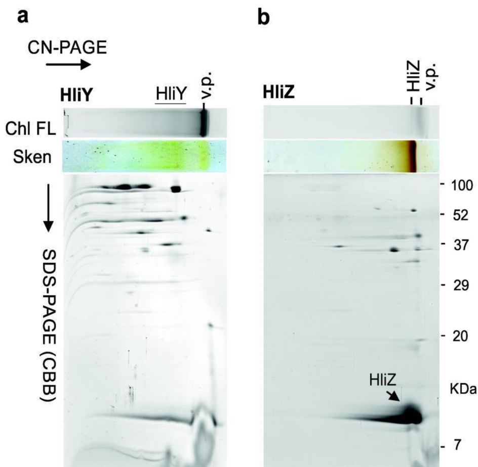
Obr. 9 2D CN/SDS-PAGE separace His-HliY a His-HliZ proteinů. Oba proteiny byly izolovány v pufru A po solubilizaci v DDM. a) Získaný proužek gelu z CN-PAGE byl před denurací skenován na fluorescenci Chl po osvětlení modrým světlem (Ch FL) pomocí Fuji LAS 4000. Proteinové komplexy byly poté separovány pomocí SDS elektroforézy (SDS-PAGE) a výsledný gel byl obarven v Coomassie blue (CBB). b) Identická analýza pro izolovaný His-HliX. v.p. – volné pigmenty.
