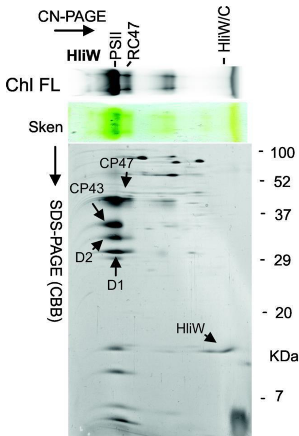
Obr. 10 2D CN/SDS-PAGE separace His-HliW proteinu izolovaného v pufru B a s použitím směsi detergentů GDN/DDM. Získaný proužek gelu z CN-PAGE byl před denurací skenován na fluorescenci Chl po osvětlení modrým světlem (Ch FL) pomocí Fuji LAS 4000. Proteinové komplexy byly poté separovány pomocí SDS elektroforézy (SDS-PAGE) a výsledný gel byl obarven v Coomassie blue (CBB). Podjednotky
