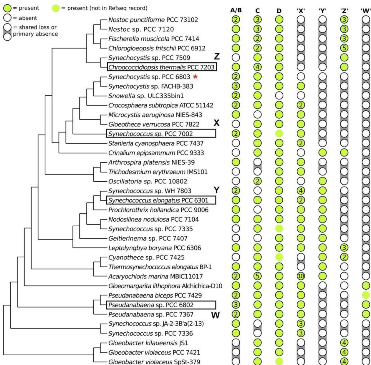
Obr. 6 Fylogenetický strom sinice, který zahrnuje všechny významné skupiny a zobrazuje přítomnost, či absenci jednotlivých typů Hlips. Hodnota v kroužku označuje počet kopií genů pro každou variantu Hlips u daného kmene. Zarámované jsou druhy, využité jako zdroj genu kódující HliW, HliX, HliY, HliZ proteiny pro expresi v Synechocystis (označený hvězdičkou) (J. Janouškovec, nepublikované výsledky).
